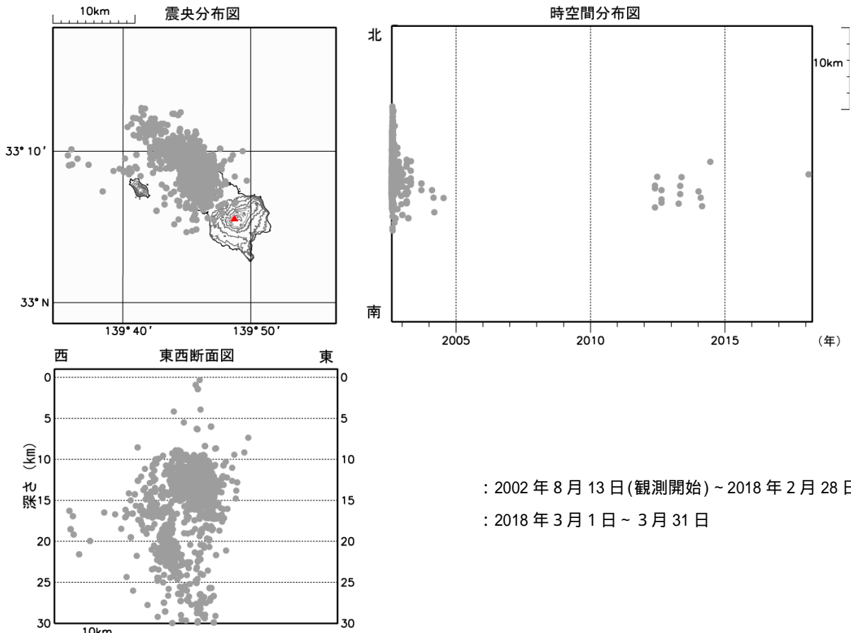
図3 八丈島 震源分布図(2002年8月13日～2018年3月31日) ・今期間、震源の求まる地震の発生はありません。
