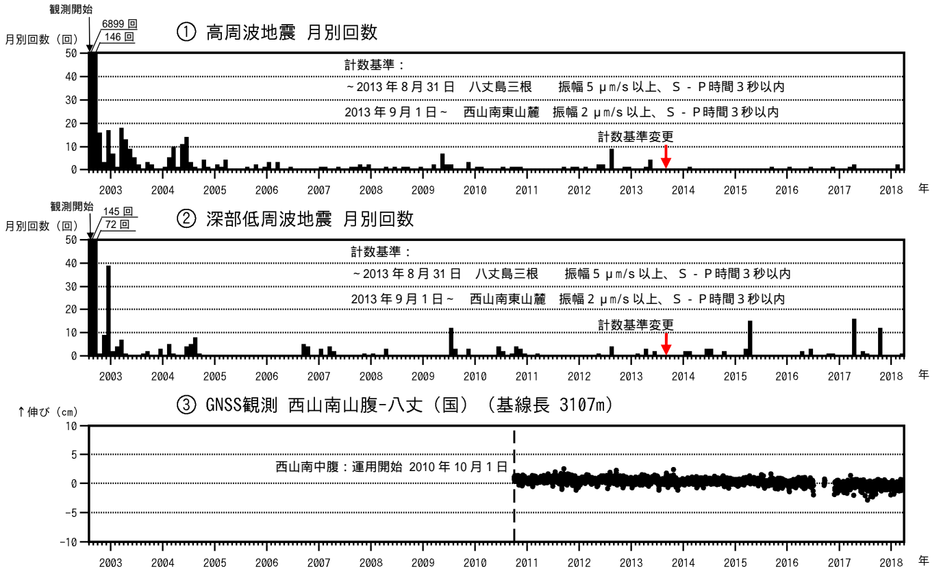
図2 八丈島 火山活動経過図(2002年8月13日~2018年3月31日)
