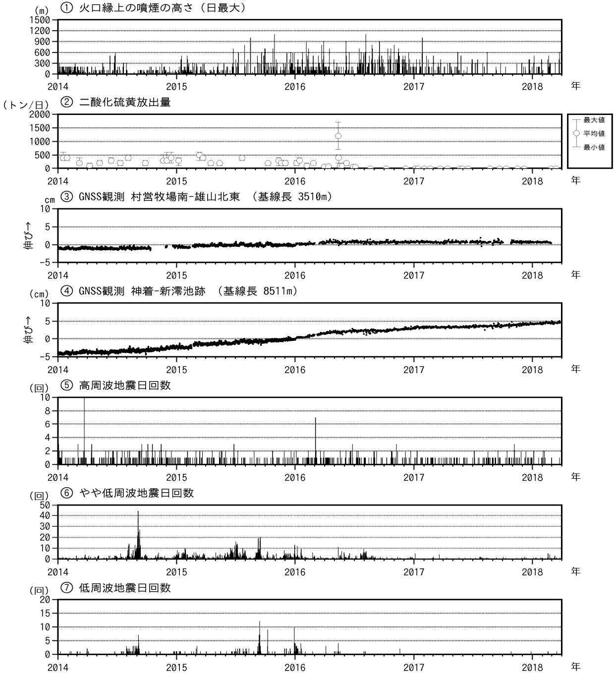
図6 三宅島 火山活動短期経過図(2014年1月1日~2018年3月31日)
