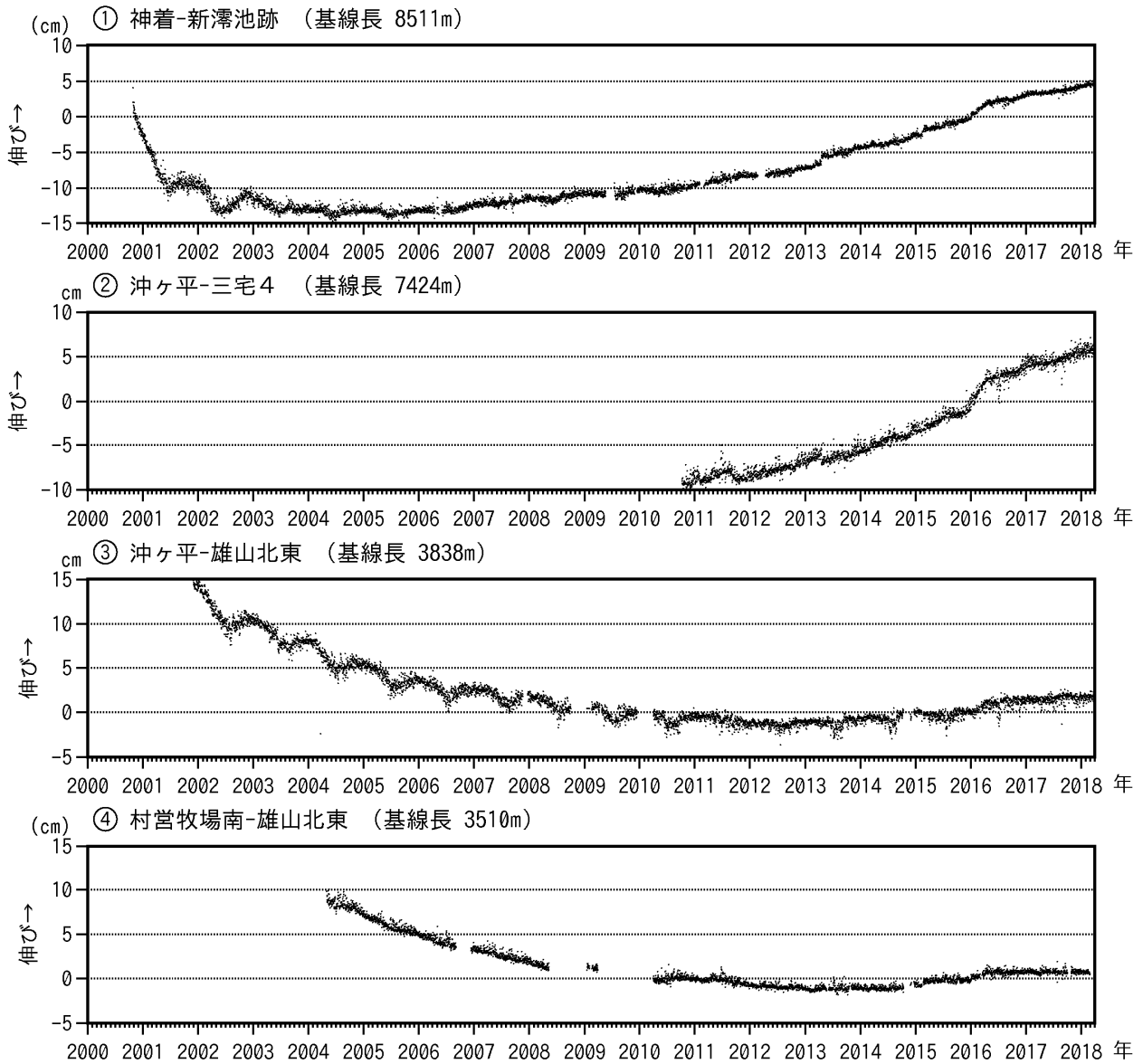
図7 三宅島 GNSS 連続観測結果 (2000年10月26日~2018年3月31日)
