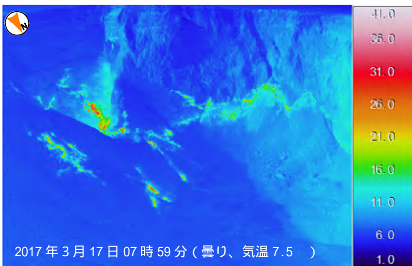
図 4 三宅島 赤外熱映像装置による山頂火口内の地表面温度分布 ・13日に実施した現地調査では、2月や昨年と同様に主火口内及びその周辺で引き続き高温領域が認められました。高温領域の分布に特段の変化は認められません。
