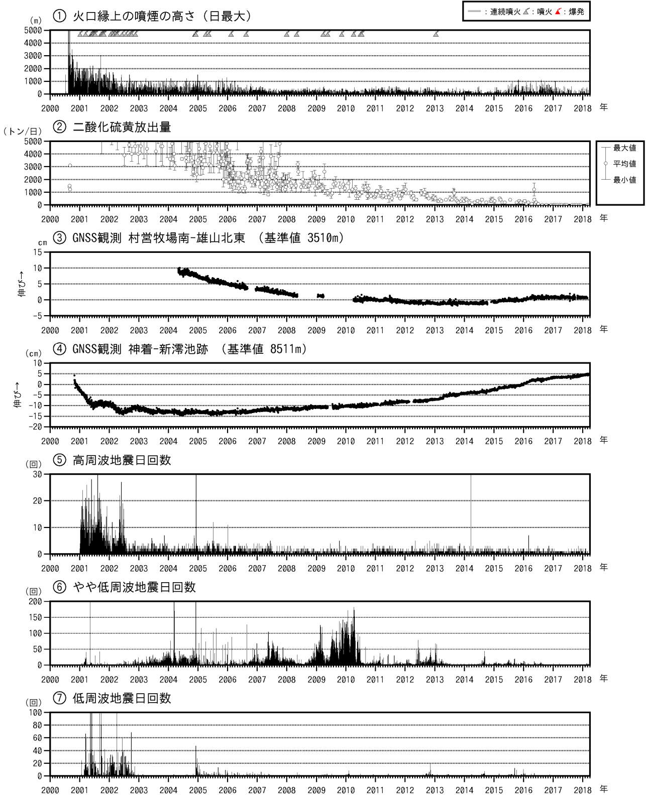
図5 三宅島 火山活動長期経過図(2000年1月1日~2018年3月31日)
