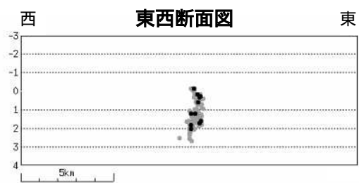
図10 三宅島 震源分布図(2017年2月1日~2018年2月28日) ・震源は山頂火口直下に分布しており、これまでと比べて特段の変化は認められません。
