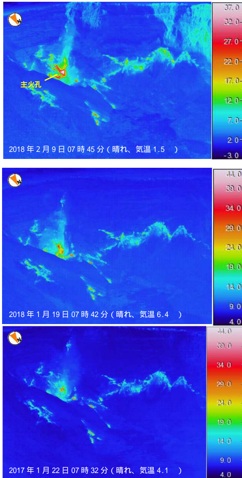
図4 三宅島 赤外熱映像装置による山頂火口内の地表面温度分布
