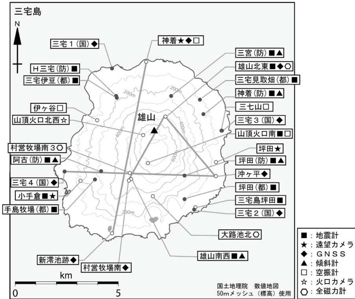
図 12 三宅島 観測点配置図
