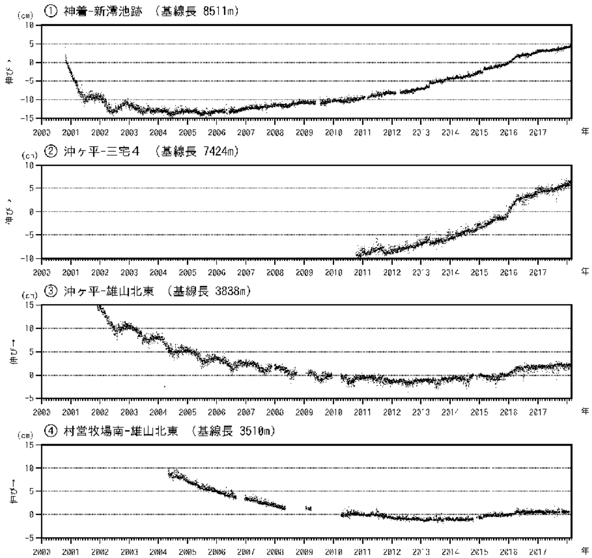
図9 三宅島 GNSS 連続観測結果 (2000年10月26日~2018年2月28日)
