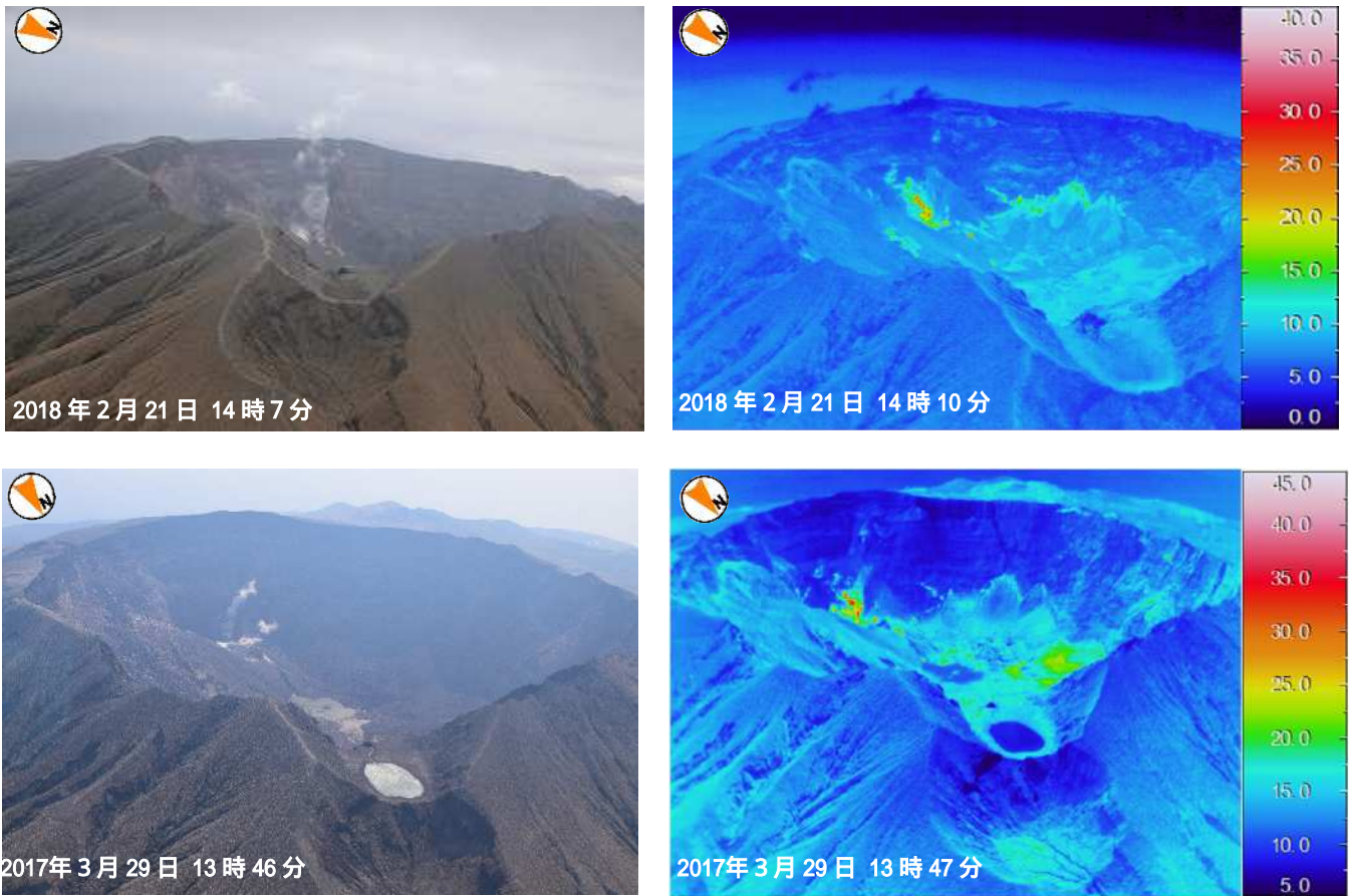
図5 三宅島 山頂火口の様子と赤外熱映像装置によるその地表面温度分布（陸上自衛隊の協力による） 上段：天気：晴れ 気温：2.4 （高度約1000mより撮影） 下段：天気：曇り 気温：12.4 （高度約1200mより撮影） ・火口の地形及び主火孔付近の高温領域の分布に特段の変化は認められません。
