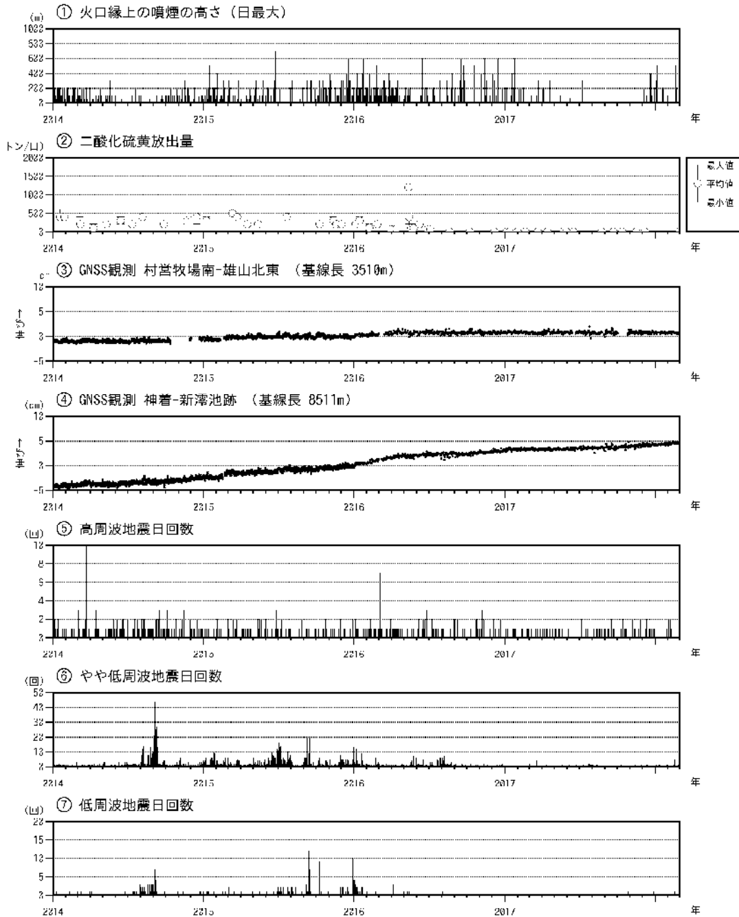
図 8 三宅島 火山活動短期経過図（2014 年 1 月 1 日～2018 年 2 月 28 日）
