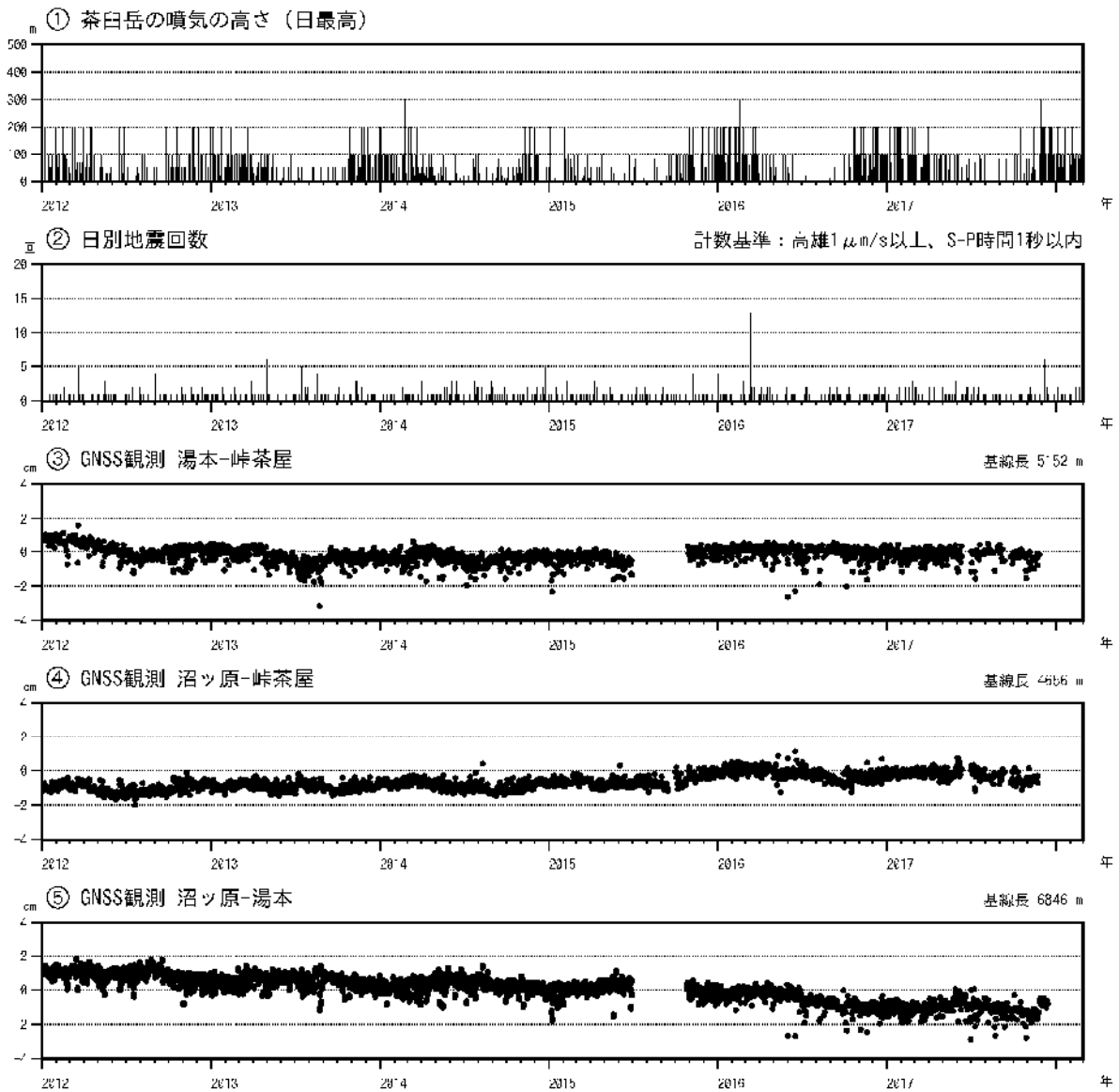
図3 那須岳 火山活動経過図(2012年1月1日~2018年2月28日)
