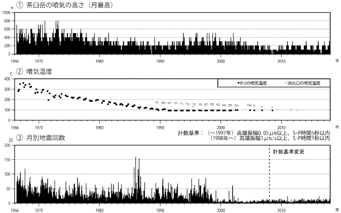
図2 那須岳 火山活動経過図(1966年1月～2018年2月)
