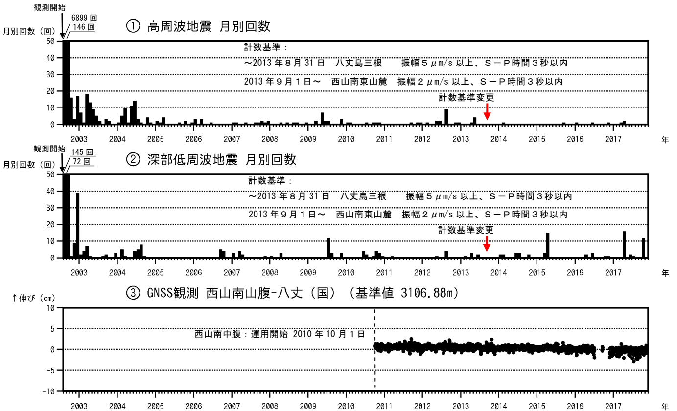
図2 八丈島 火山活動経過図 (2002年8月13日~2017年11月30日)
