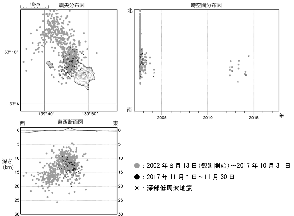
図3 八丈島 震源分布図（2002年8月13日～2017年11月30日）
