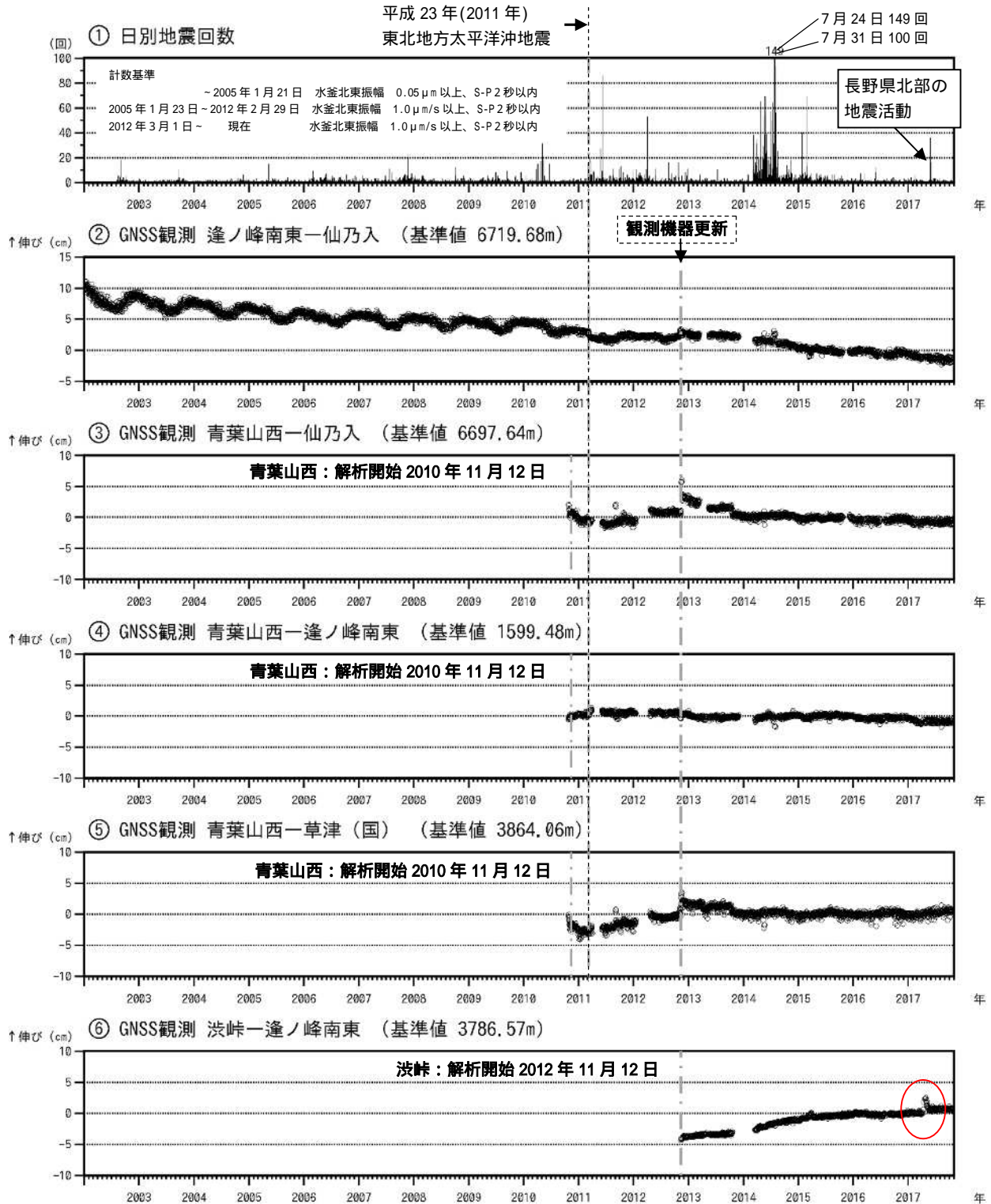
図9 草津白根山 火山活動経過図 (2002年4月1日~2017年10月31日)
