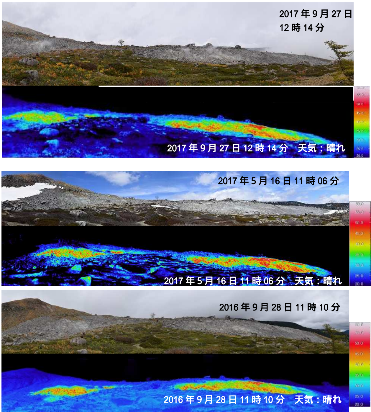
図6 草津白根山 水釜火口北東部の状況
