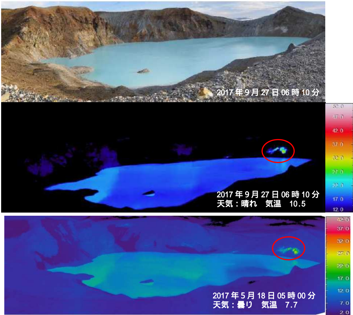
図3 草津白根山 湯釜火口内壁の赤外熱映像
