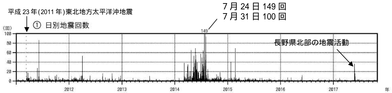
図8 草津白根山 日別地震回数（2011年1月1日～2017年10月31日） ・2014年8月下旬以降は2015年1月と2月に一時的な増加がみられたものの、概ね少ない状態で経過しています。
