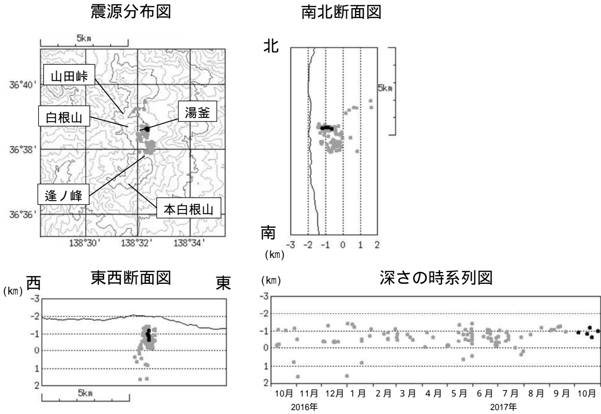
図7 草津白根山 震源分布図（2016年10月1日～2017年10月31日） : 2016年10月1日～2017年9月30日 : 2017年10月1日～10月31日
