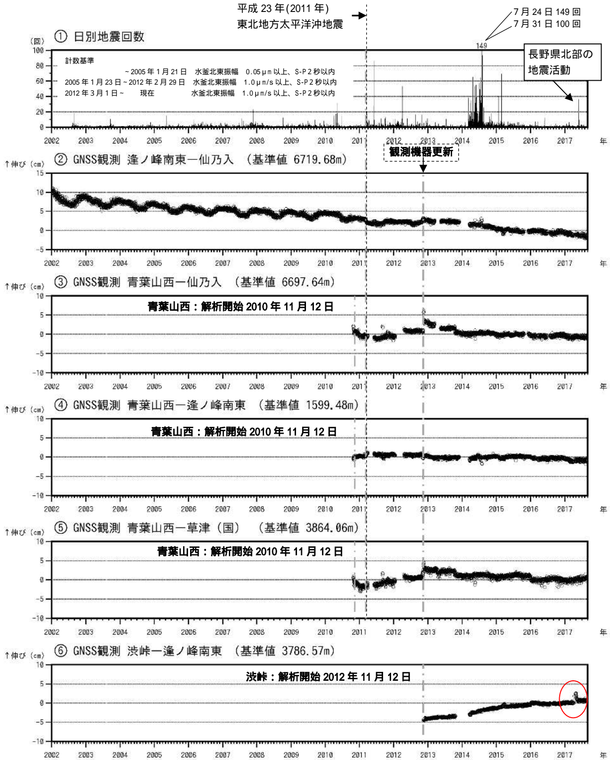
図5 草津白根山 火山活動経過図 (2002年4月1日~2017年8月31日)
