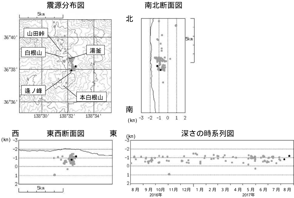
図3 草津白根山 震源分布図（2016年8月1日～2017年8月31日） : 2016年8月1日～2017年7月31日 : 2017年8月1日～8月31日
