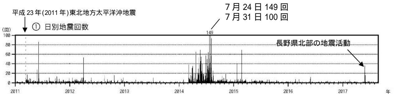
図4 草津白根山 日別地震回数（2011年1月1日～2017年8月31日） ・2014年8月下旬以降は2015年1月と2月に一時的な増加がみられたものの、概ね少ない状態で経過しています。
