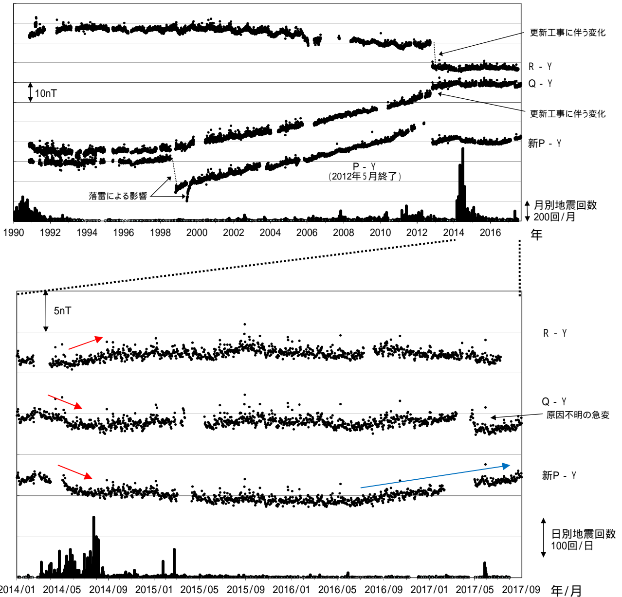
図6 草津白根山 全磁力連続観測による全磁力値の変化及び地震回数 上段：1990年～2017年9月2日、下段：2014年1月～2017年9月2日
