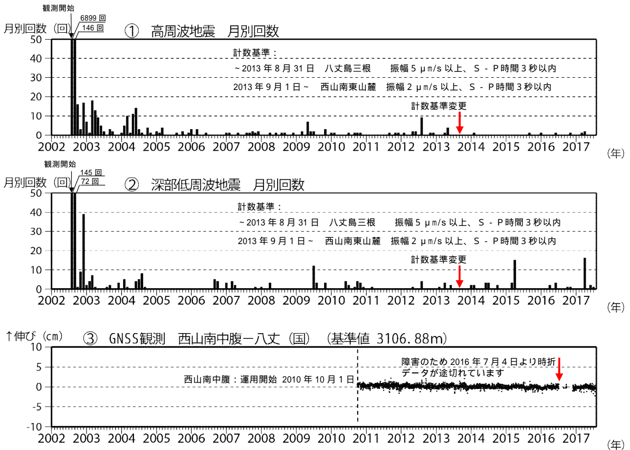
図2 八丈島 火山活動経過図(2002年8月13日~2017年7月31日)
