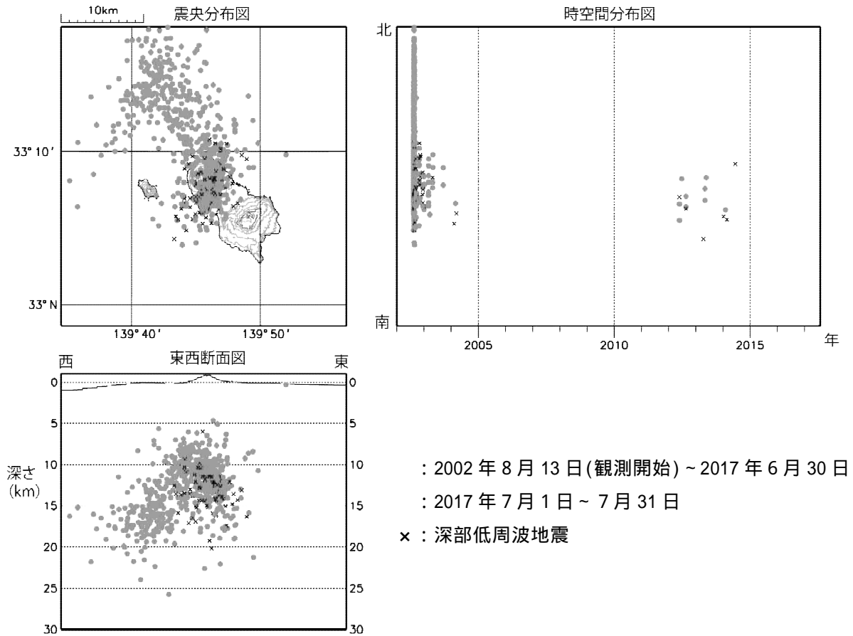
図3 八丈島 震源分布図(2002年8月13日～2017年7月31日) ・今期間、八丈島付近に震源が求まる高周波地震及び深部低周波地震はありませんでした。
