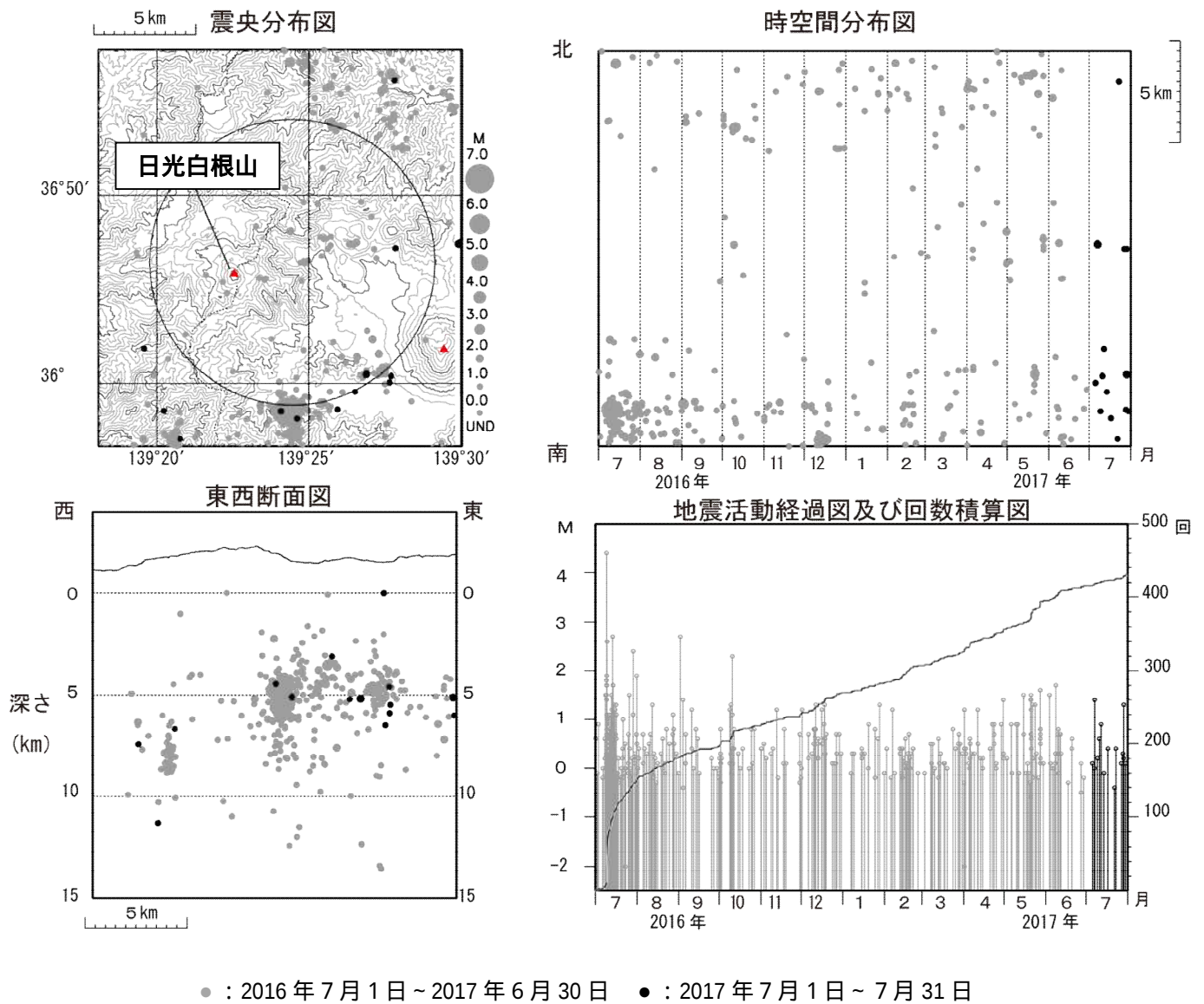
図 3 日光白根山 広域地震観測網による山体・周辺の地震活動(2016 年 7 月 1 日 ~ 2017 年 7 月 31 日) ・震央分布図中の円は図 2 - の計数対象地震（五色沢で S - P 時間 1 秒以内）のおよその範囲を示しています。 ・震源の深さは全て海面以下として決定しています。 ・図中の震源要素は一部暫定値が含まれており、後日変更することがあります。 ・日光白根山付近を震源とする地震の発生は少なく、地震活動は低調に経過しています。
