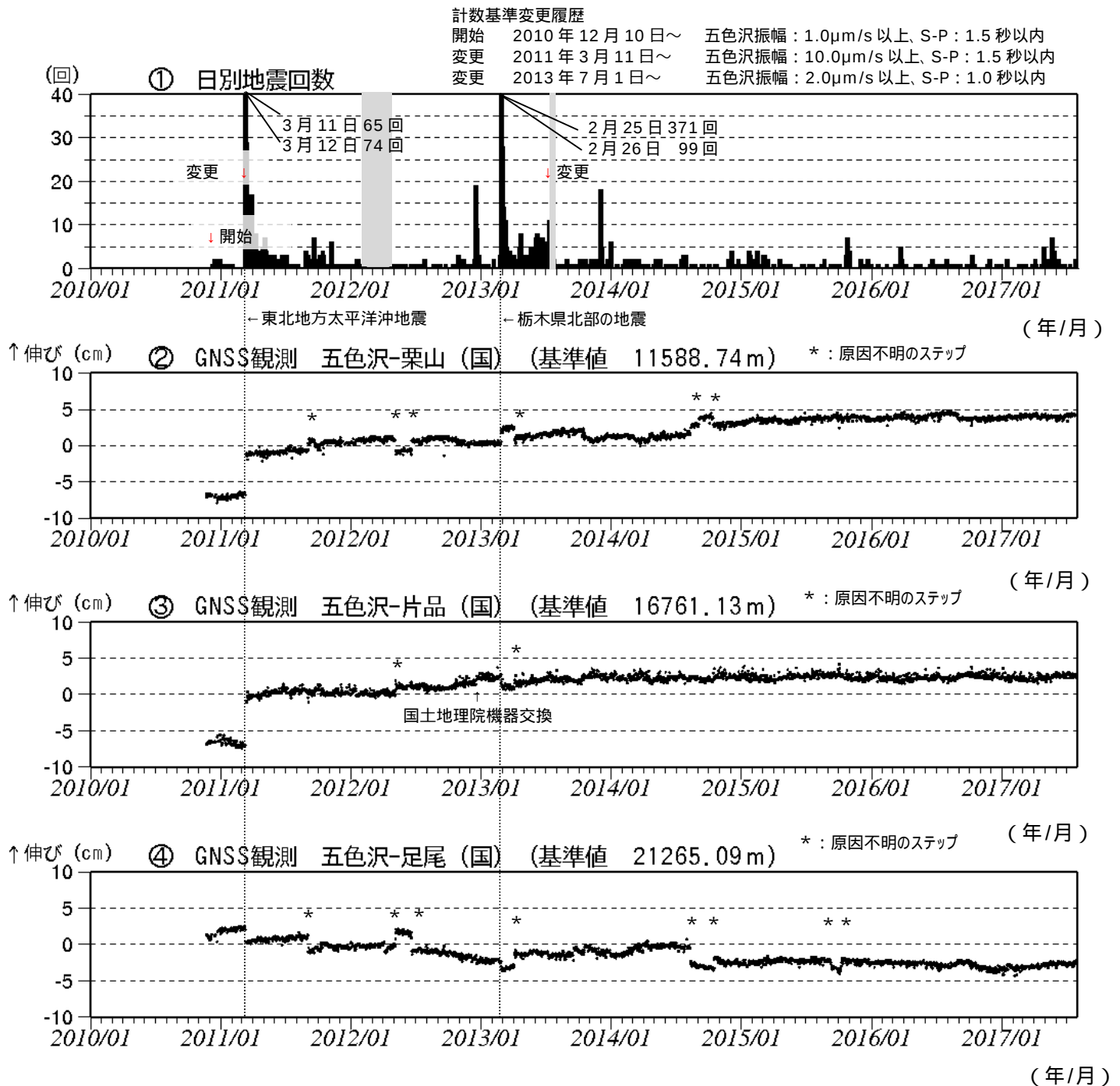
図2 日光白根山 火山活動経過図 (2010 年 11 月 20 日～2017 年 7 月 31 日)
