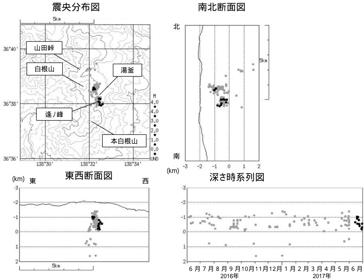
図5 草津白根山 震源分布図（2016年6月1日～2017年6月30日） : 2016年6月1日～2017年5月31日 : 2017年6月1日～6月30日
