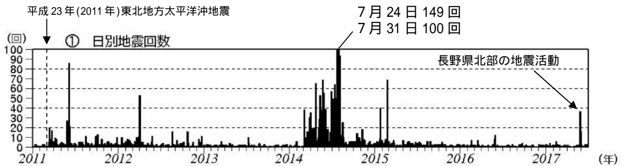
図6 草津白根山 日別地震回数（2011年1月1日～2017年6月30日） ・2014年3月上旬から湯釜付近及びその南側を震源とする火山性地震が増加しました。2014年8月下旬以降は2015年1月と2月に一時的な増加がみられたものの、概ね少ない状態で経過しています。 ・5月27日～28日に一時的に地震回数が増加しましたが、この地震の多くは山頂から比較的離れた長野県北部の地震（M4.4）に伴う一連の地震活動によるものです。
