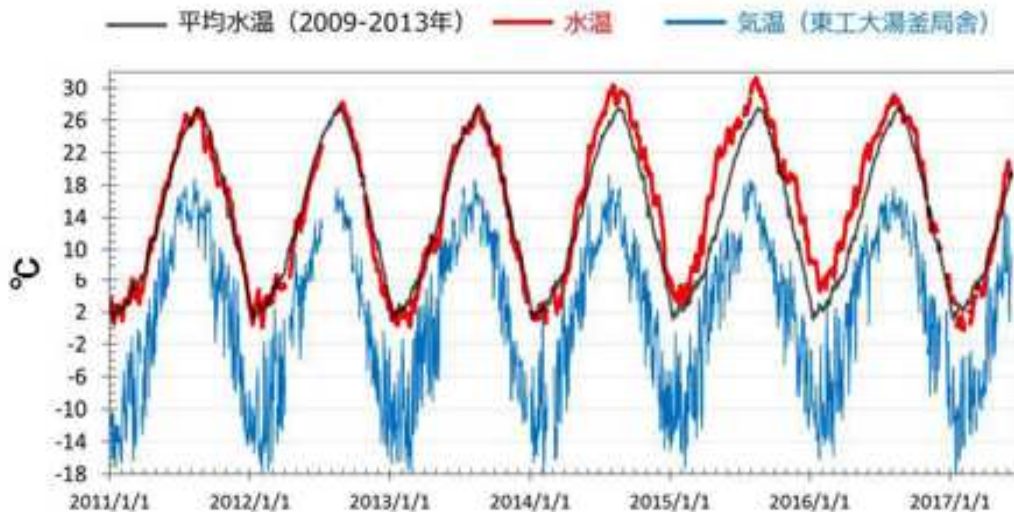
図4 草津白根山 湯釜火口湖の水温 (赤線：実際に観測された水温、灰色線：2009～13年に測定された毎年同一日の水温を平均し、その日付に対して示したもの、青色：東工大湯釜局舎で測定された気温)(東京工業大学(2017)) ・湯釜水温は、2014年5月頃から2016年8月頃まで平年より数 高い状態でしたが、2016年8月以降は平年値に戻っています。
