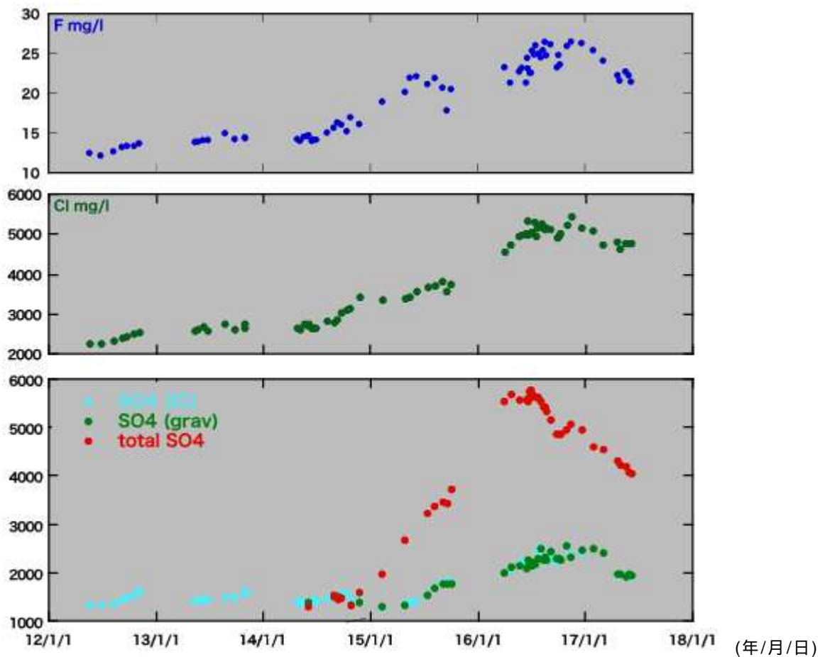
図3 草津白根山 湯釜湖水の化学組成変化(2012年～2017年6月)(東京工業大学・上智大学(2017)) ・湯釜湖水の化学組成は、2014年以降、火山活動が活発な状態であることを示していましたが、2017年に入って低下傾向に転じていることが確認されました。
