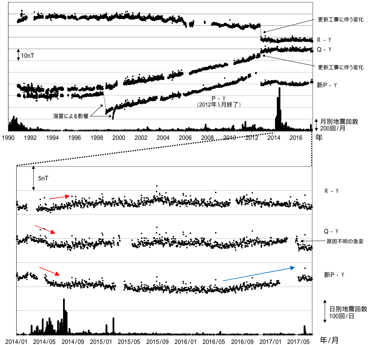
図8 草津白根山 全磁力連続観測による全磁力値の変化及び地震回数
