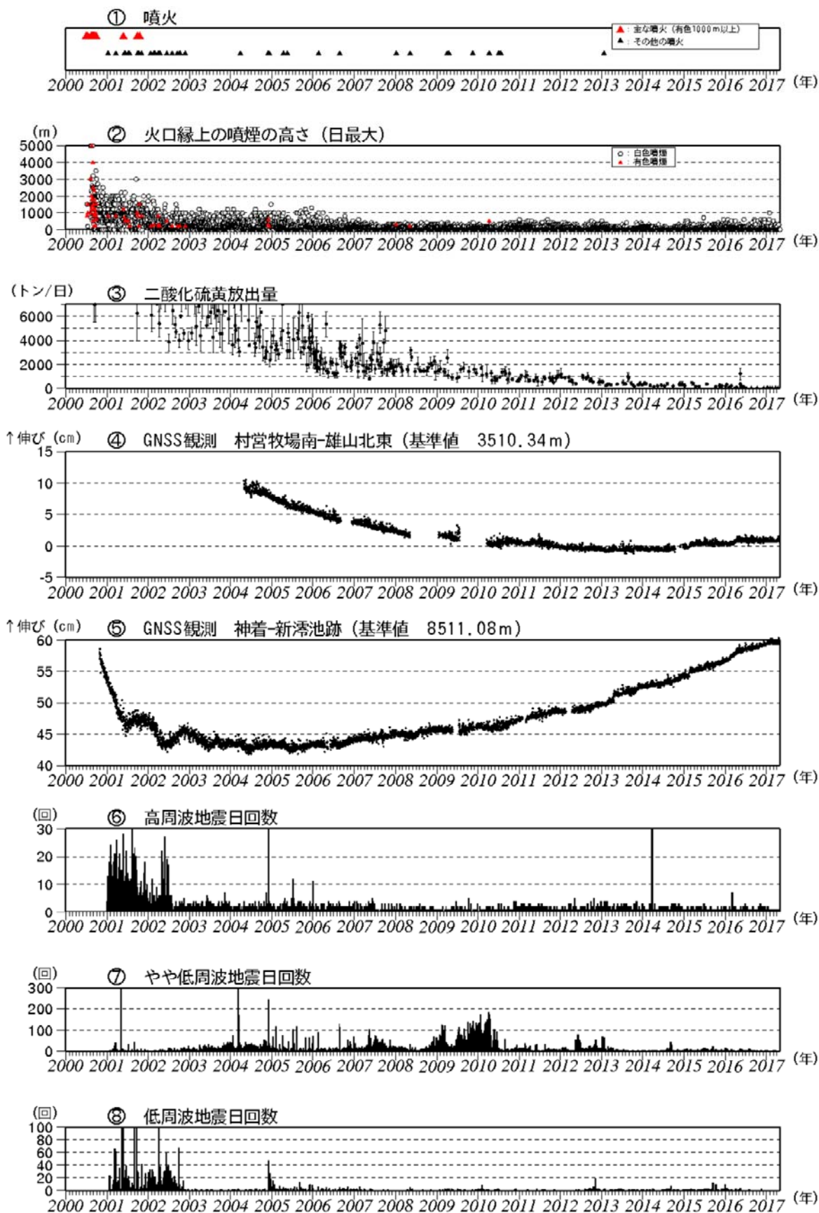
図5 三宅島 火山活動長期経過図 (2000年1月1日~2017年4月30日)
