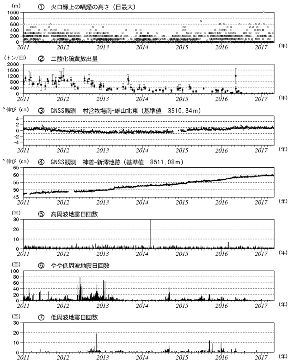
図6 三宅島 火山活動短期経過図（2011年1月1日～2017年4月30日）
