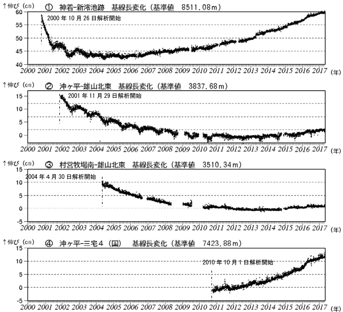
図7 三宅島 GNSS 連続観測結果 (2000年10月26日~2017年4月30日)
