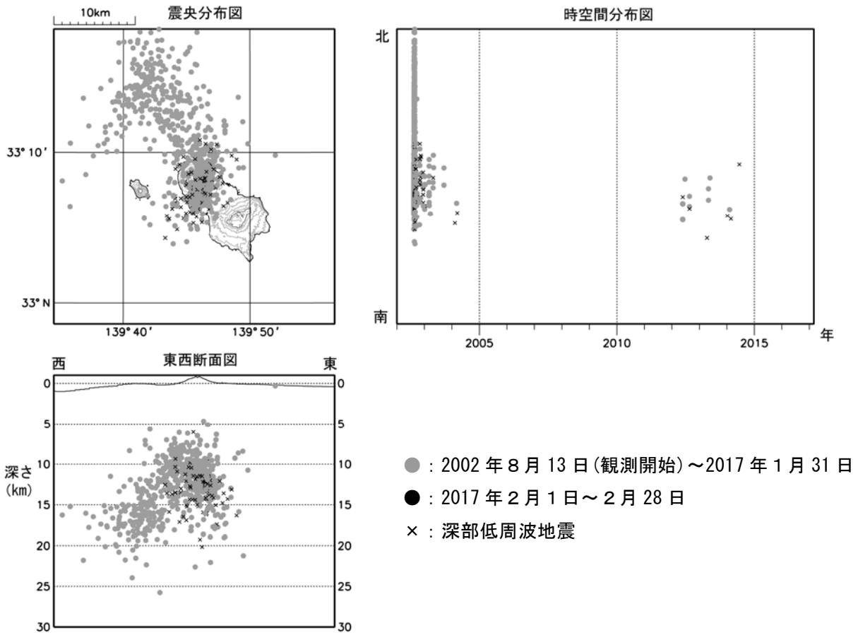
図3 八丈島 震源分布図（2002年8月13日～2017年2月28日） ・今期間、八丈島付近に震源が求まる高周波地震及び深部低周波地震はありませんでした。
