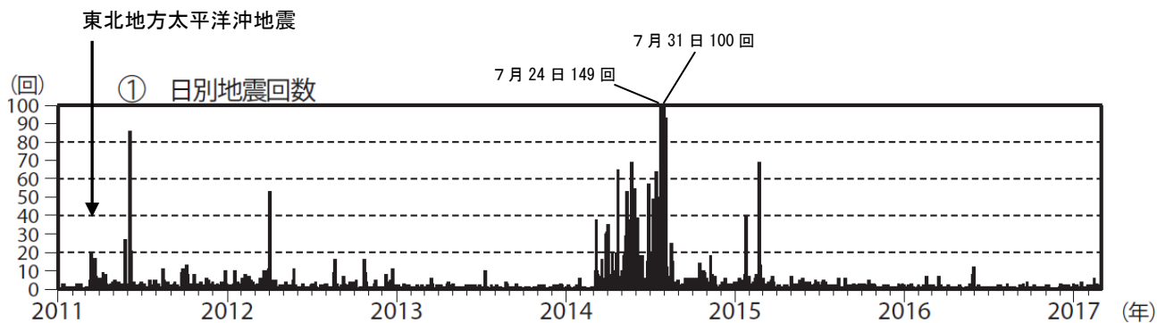
図6 草津白根山 日別地震回数 (2011年1月1日~2017年2月28日)
