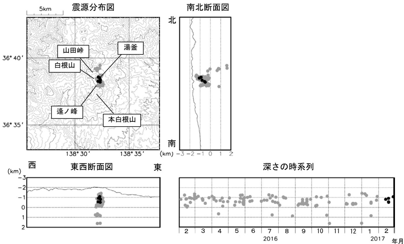
図5 草津白根山 震源分布図 (2016年2月1日~2017年2月28日)
