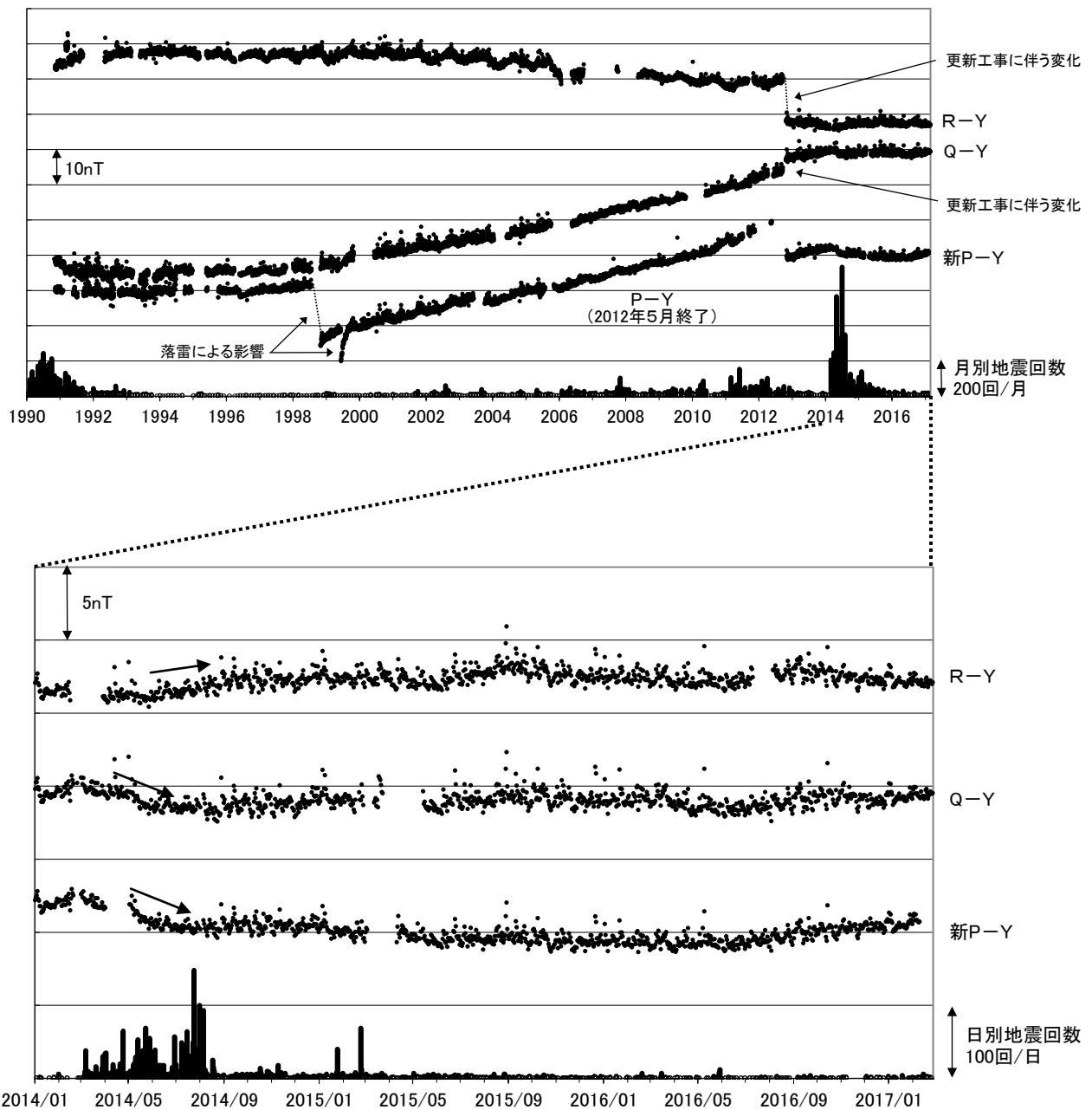
図8 草津白根山 全磁力連続観測による全磁力値の変化及び地震回数 上段：1990年～2017年1月25日、下段：2014年1月～2017年2月26日
