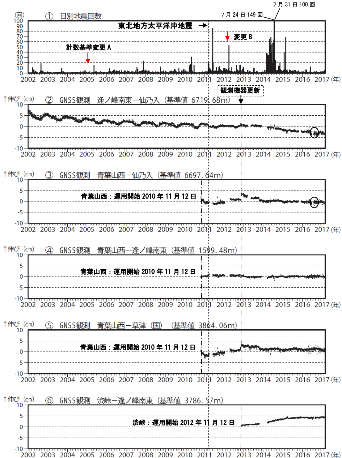
図7 草津白根山 火山活動経過図（2002年4月1日～2017年2月28日）
