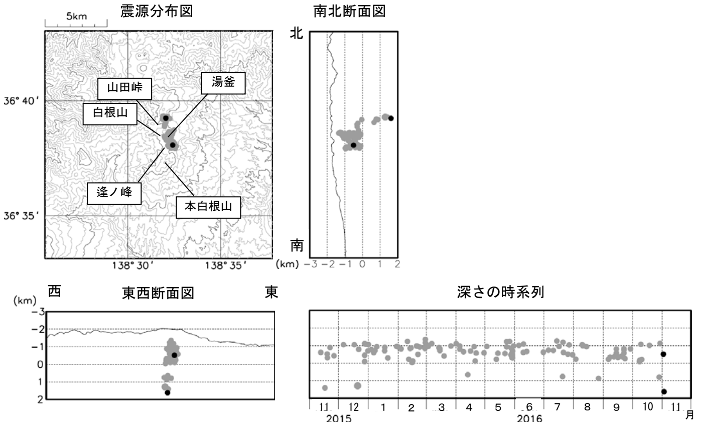
図3 草津白根山 震源分布図（2015年11月1日～2016年11月30日）
