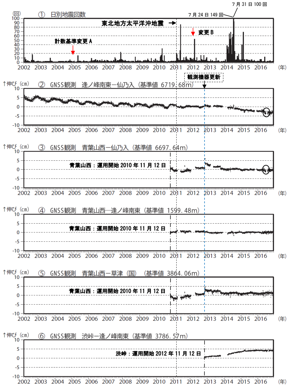
図5 草津白根山 火山活動経過図（2002年4月1日～2016年11月30日）
