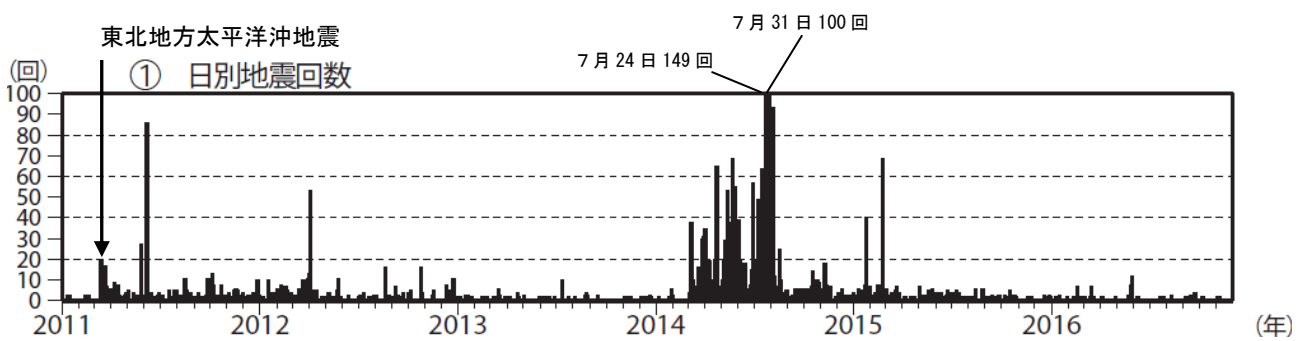
図4 草津白根山 日別地震回数（2011年1月1日～2016年11月30日）
