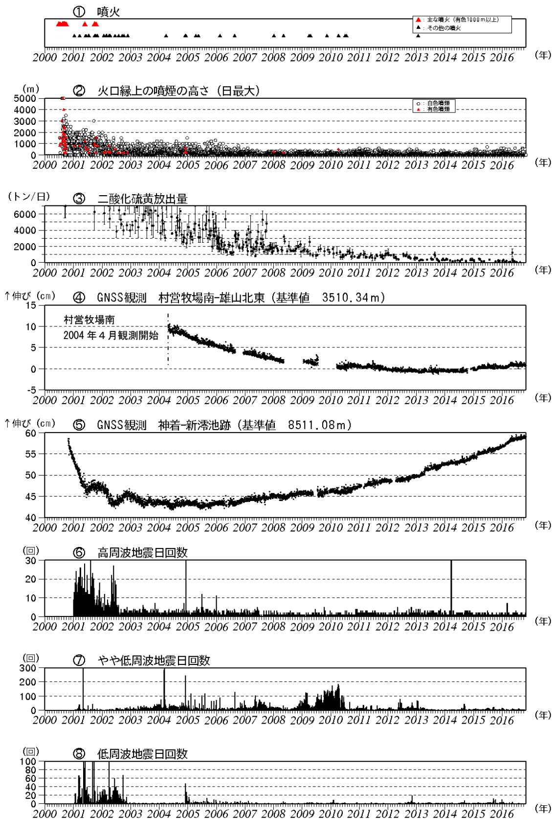
図4 三宅島 火山活動長期経過図 (2000年1月1日~2016年10月31日) ※図4の説明は次ページに掲載しています。
