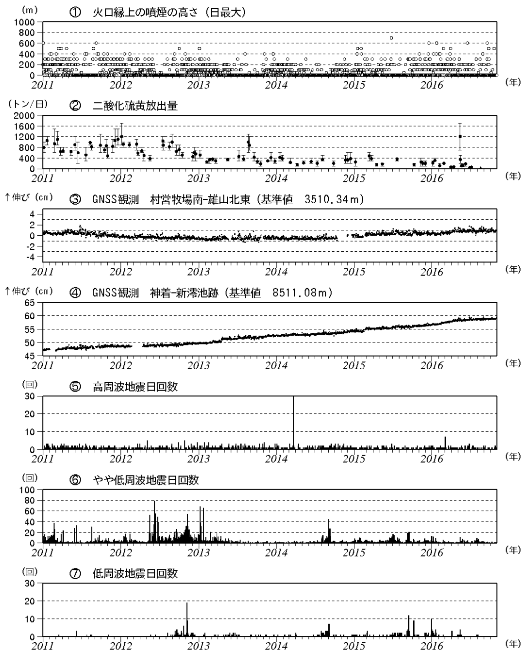
図5 三宅島 火山活動短期経過図 (2011年1月1日～2016年10月31日)
