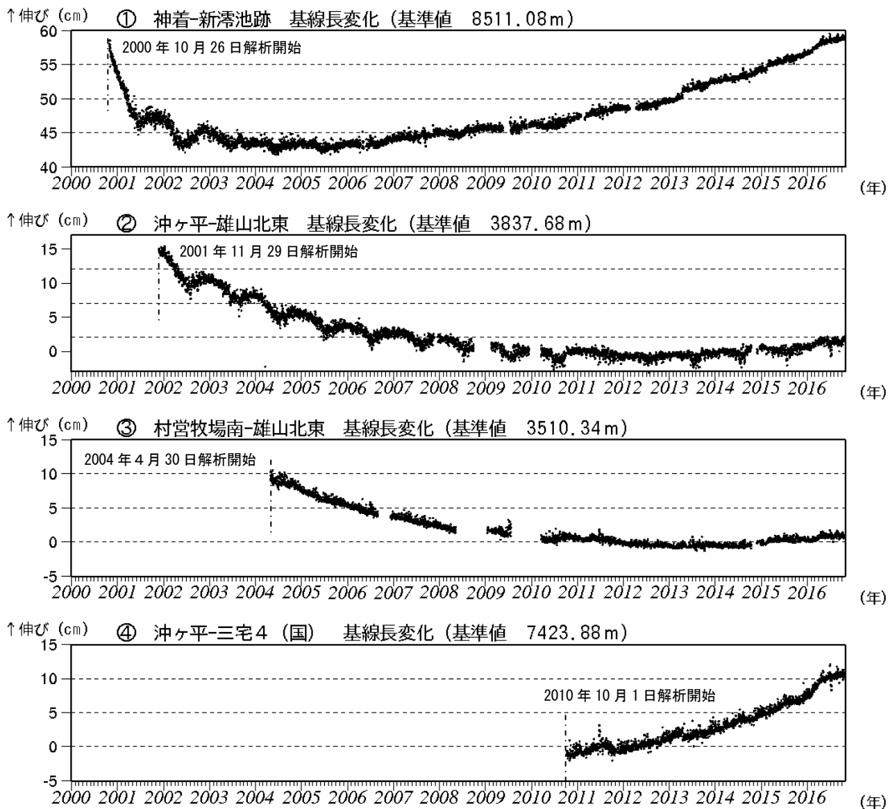
図6 三宅島 GNSS 連続観測結果 (2000 年 10 月 26 日～2016 年 10 月 31 日) (国) : 国土地理院
