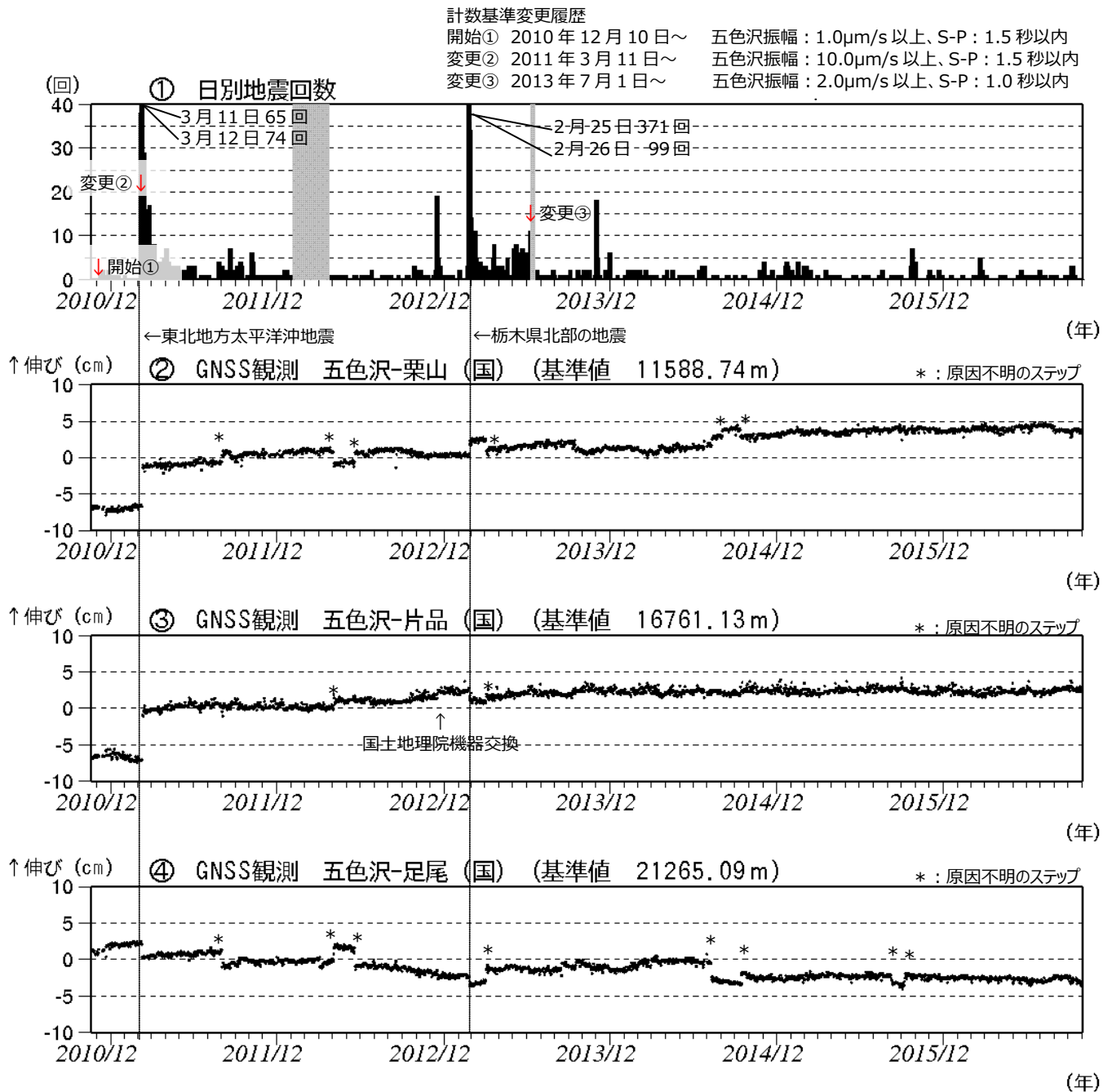
図2 日光白根山 火山活動経過図 (2010 年 11 月 20 日～2016 年 10 月 31 日)
