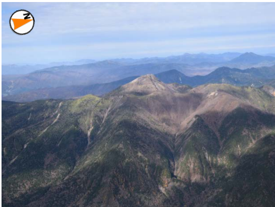
図 7 日光白根山南方の状況 (図 8 の③から撮影)
