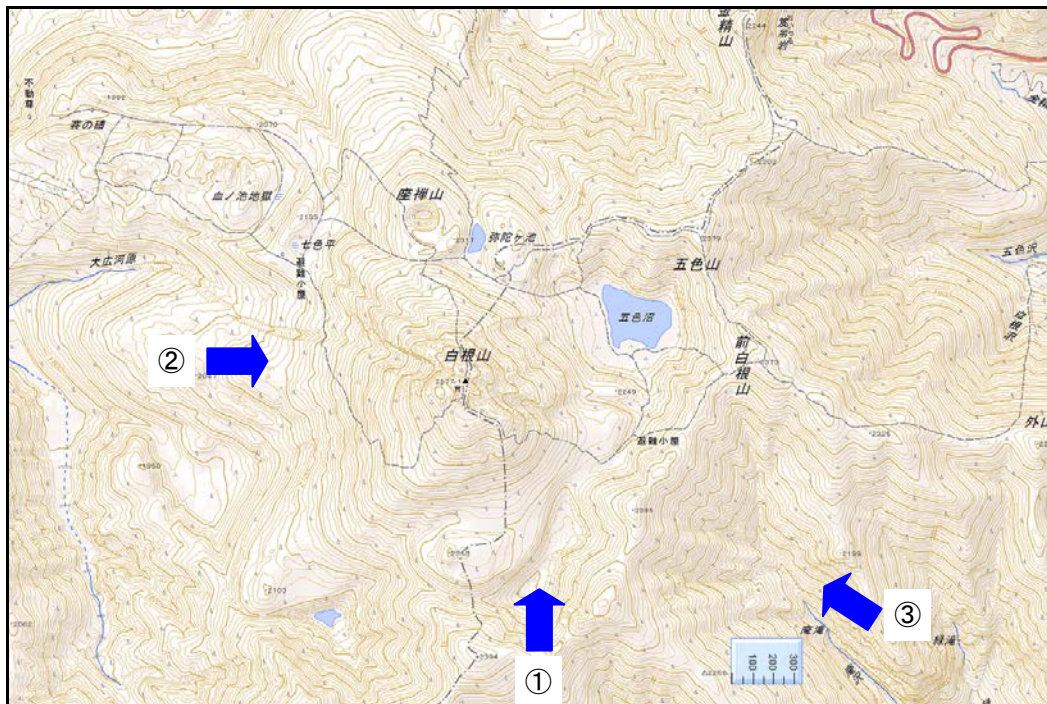
図 8 日光白根山山頂付近 図中の矢印は図 5～7 の撮影位置と撮影方向を示しています
