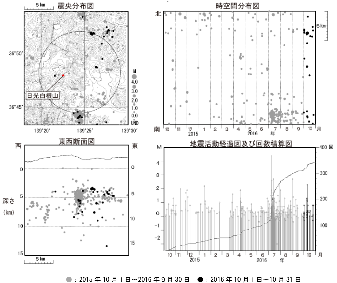
図3 日光白根山 広域地震観測網による山体・周辺の地震活動(2015 年 10 月 1 日～2016 年 10 月 31 日) ・震央分布図中の円は図2-①の計数対象地震（五色沢でS-P時間1秒以内）のおよその範囲を示しています。 ・M（マグニチュード）は地震の規模を表します。 ・震源の深さは全て海面以下として決定しています。 ・図中の震源要素は一部暫定値が含まれており、後日変更することがあります。 ・日光白根山付近を震源とする地震の発生は少なく、地震活動は低調に経過しています。
