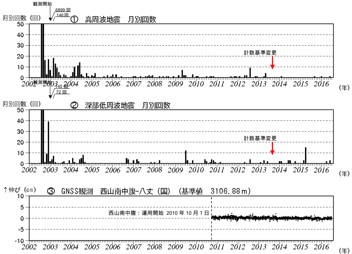
図2 八丈島 火山活動経過図(2002年8月13日~2016年7月31日)
