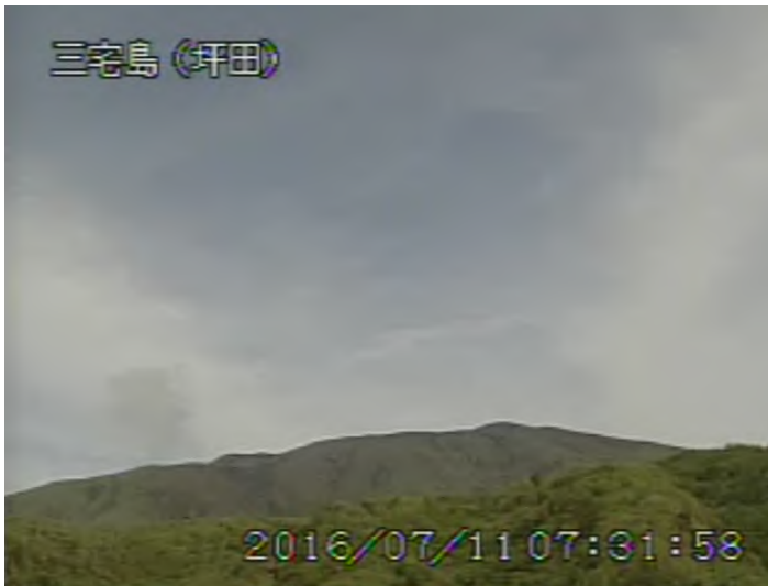
図 1 三宅島 山頂火口からの噴煙の状況 （7月11日、坪田遠望カメラによる）
