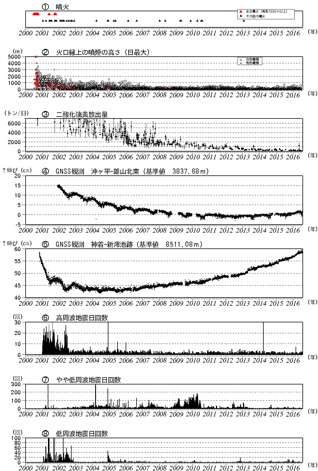
図4 三宅島 火山活動長期経過図 (2000年1月1日~2016年7月31日) 図4の説明は次ページに掲載しています。
