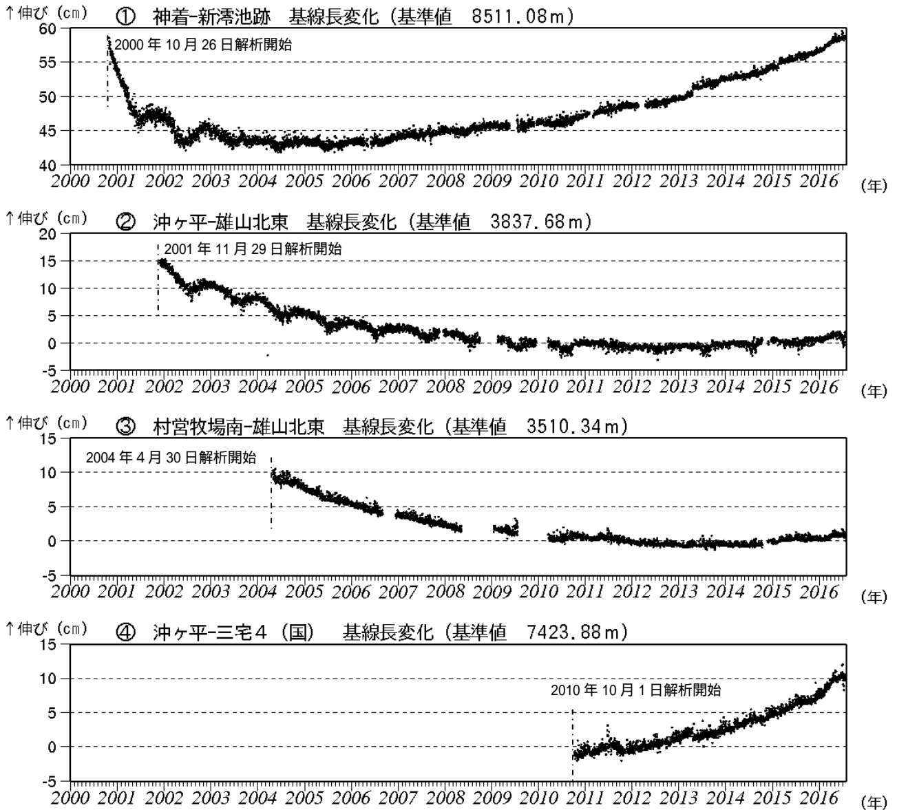
図6 三宅島 GNSS 連続観測結果 (2000年10月26日~2016年7月31日) (国): 国土地理院
