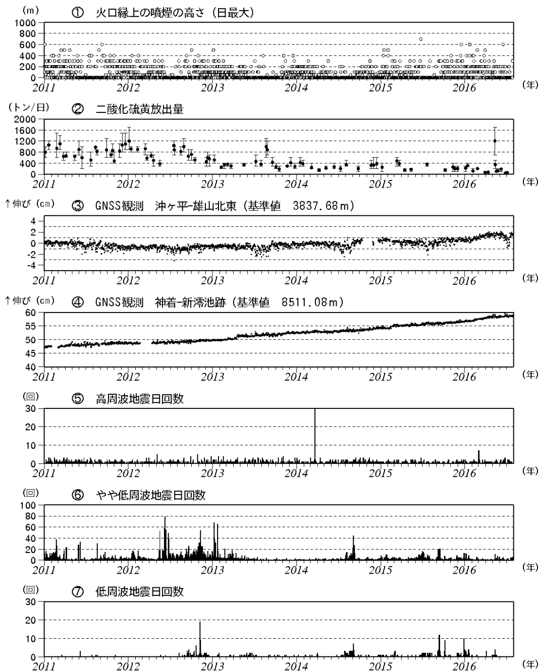
図5 三宅島 火山活動短期経過図(2011年1月1日~2016年7月31日)
