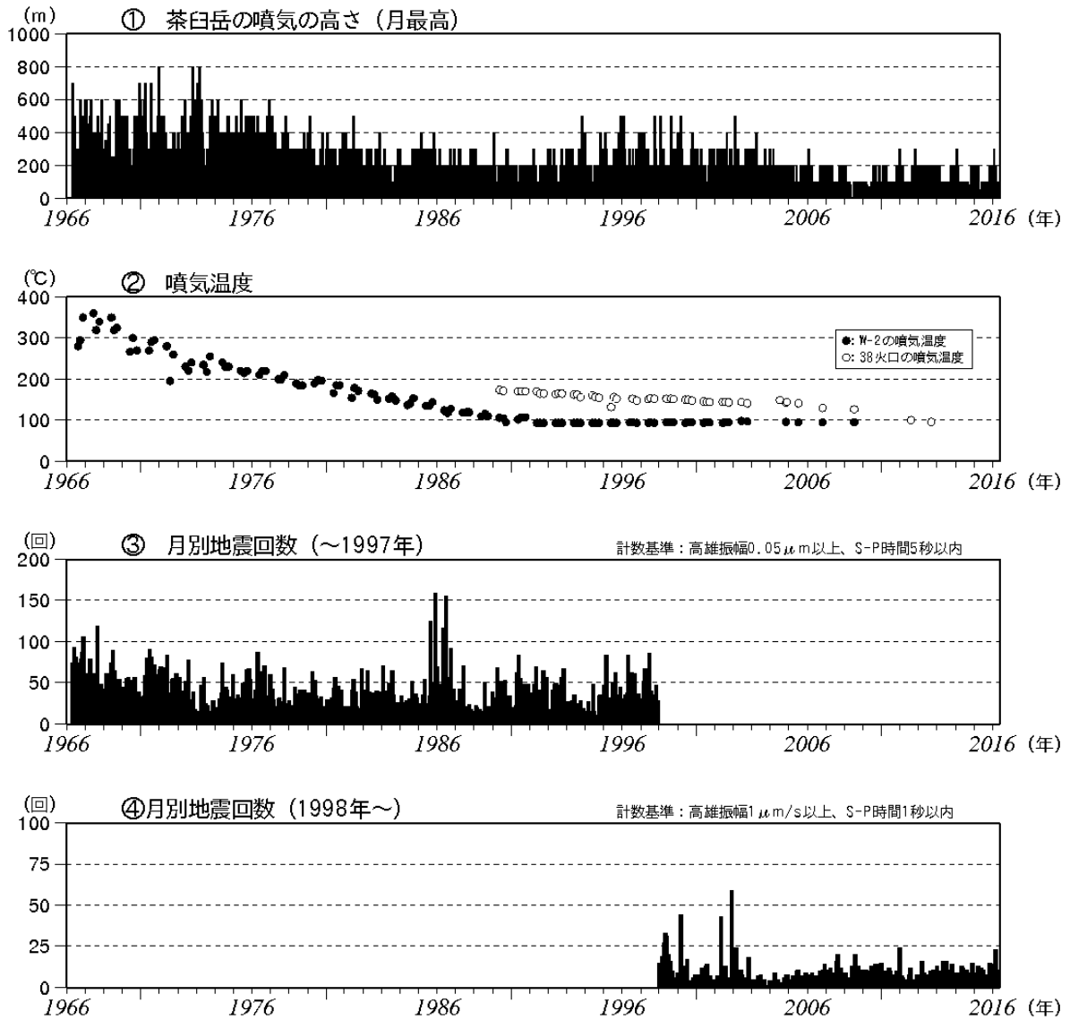
図2 那須岳 火山活動長期経過図(1966年1月~2016年5月) 定時観測(09時・15時)による月最大値 噴気温度(W-2及び38火口はいずれも茶臼岳西側斜面の温度観測定点) 那須岳周辺も含めた月別地震回数(~1997年) 那須岳山体付近に発生した月別地震回数(1998年~)
