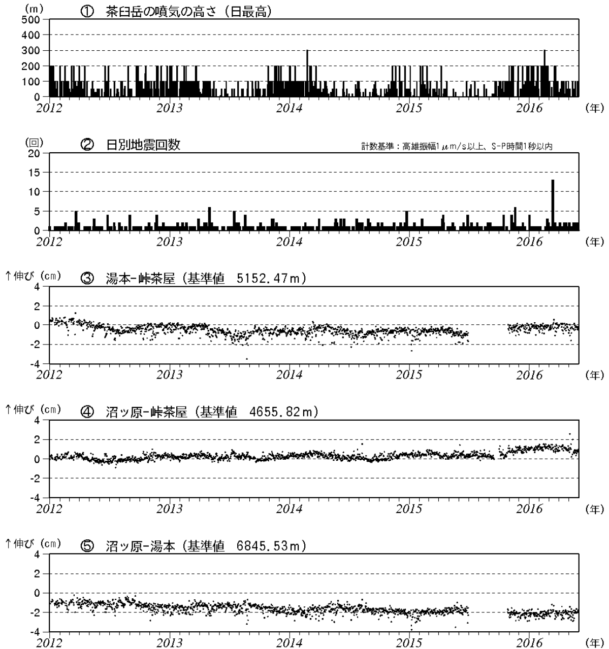
図3 那須岳 火山活動経過図(2012年1月1日~2016年5月31日) 定時観測(09時・15時)による日最大値
