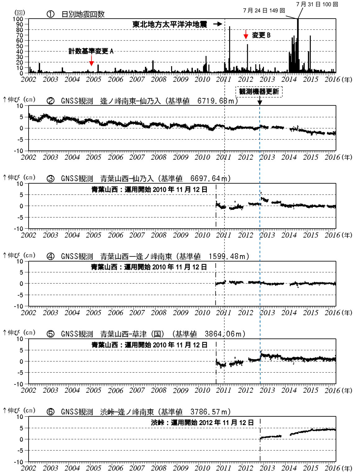
図5 草津白根山 火山活動経過図 (2002年4月1日~2016年4月30日)
