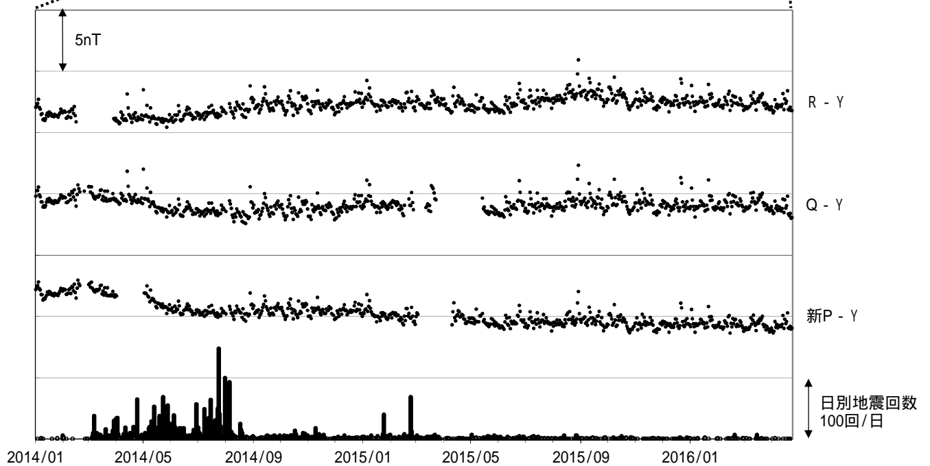
図 7 草津白根山 全磁力連続観測による全磁力値の変化及び日別地震回数（2014 年 1 月～2016 年 4 月 23 日）
