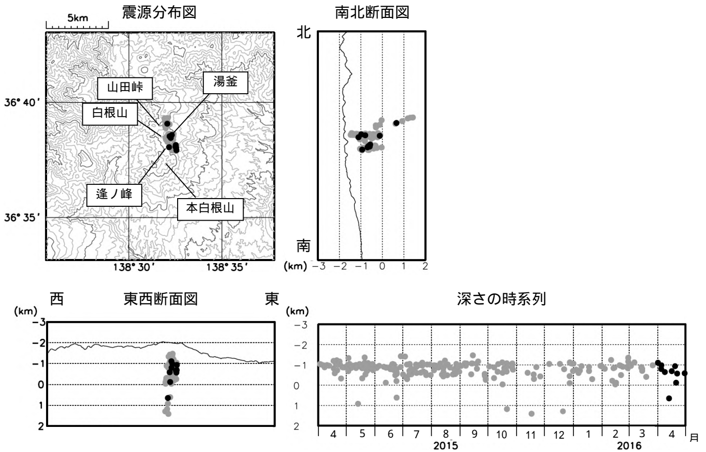
図3 草津白根山 震源分布図(2015年4月1日~2016年4月30日) : 2015年4月1日~2016年3月31日 : 2016年4月1日~4月30日
