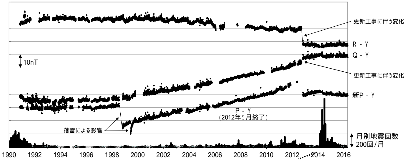
図 6 草津白根山 全磁力連続観測による全磁力値の変化及び月別地震回数（1990 年～2016 年 4 月 23 日）
