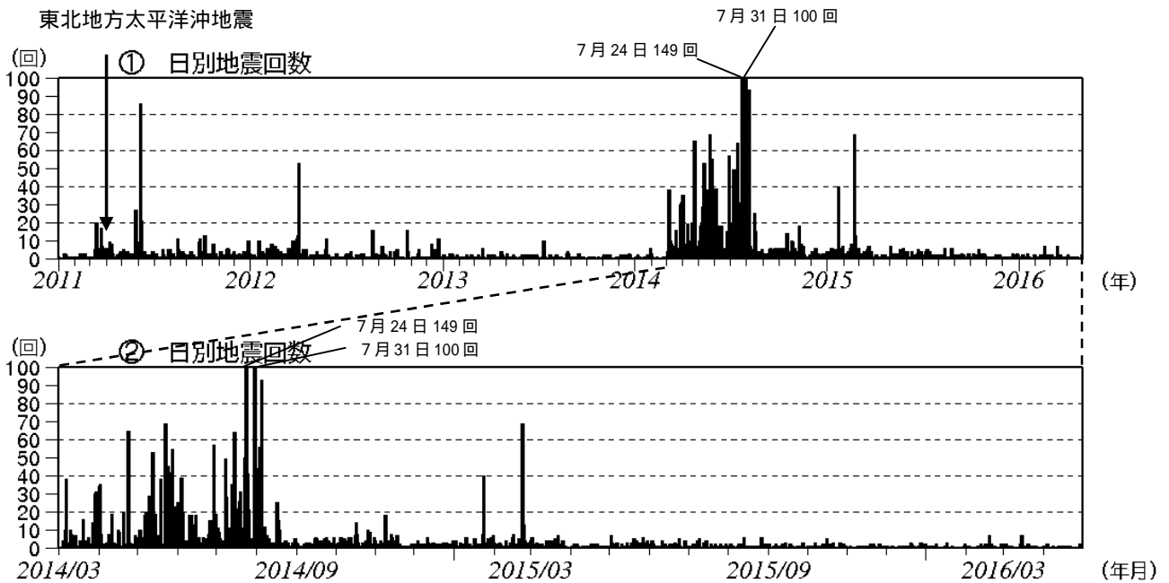
図4 草津白根山 日別地震回数(2011年1月1日~2016年4月30日) ・2014年3月上旬から湯釜付近及びその南側を震源とする火山性地震が増加しました。2014年8月下旬以降は2015年1月と2月に一時的な増加がみられたものの、概ね少ない状態で経過しています。
