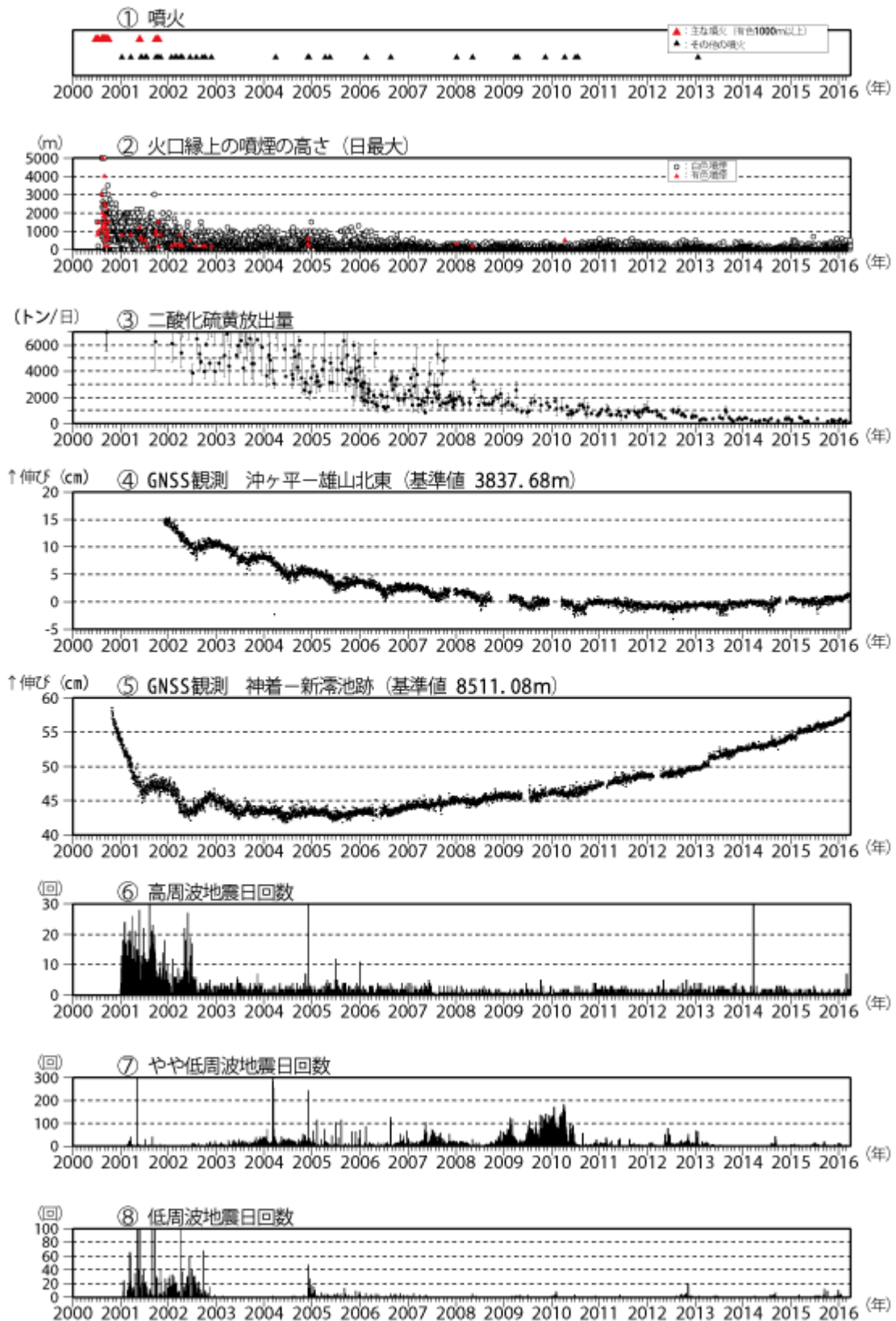
図4 三宅島 火山活動長期経過図 (2000年1月1日~2016年3月31日) 図5の説明は次ページに掲載しています。
