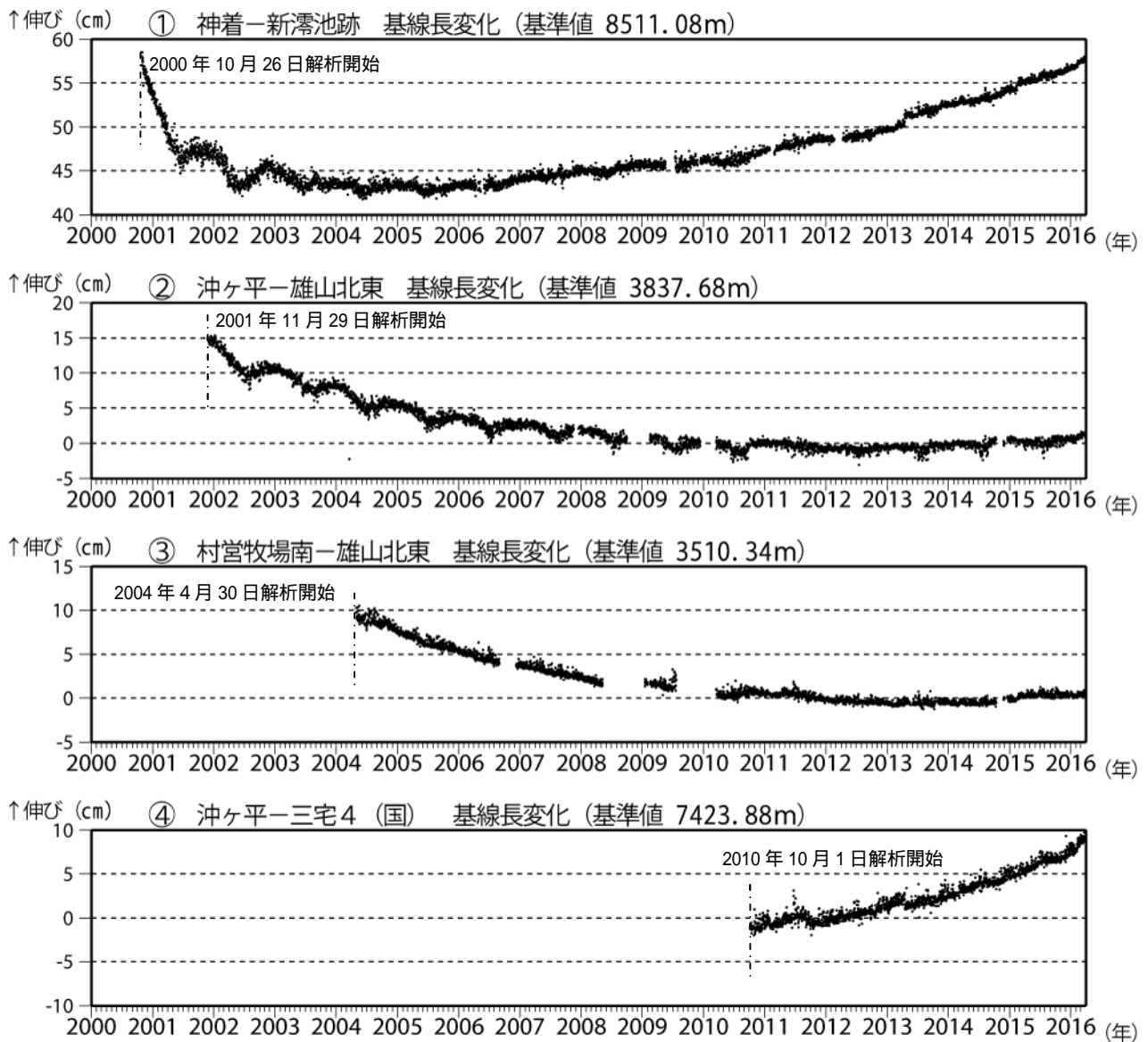
図6 三宅島 GNSS 連続観測結果 (2000年10月26日~2016年3月31日) (国): 国土地理院 ・基線 ~ は図9 (観測点配置図) の ~ にそれぞれ対応します。 ・グラフの空白部分は欠測を示します。 ・2010年10月以降のデータについては、電離層の影響を補正する等、解析方法を改良しています。
