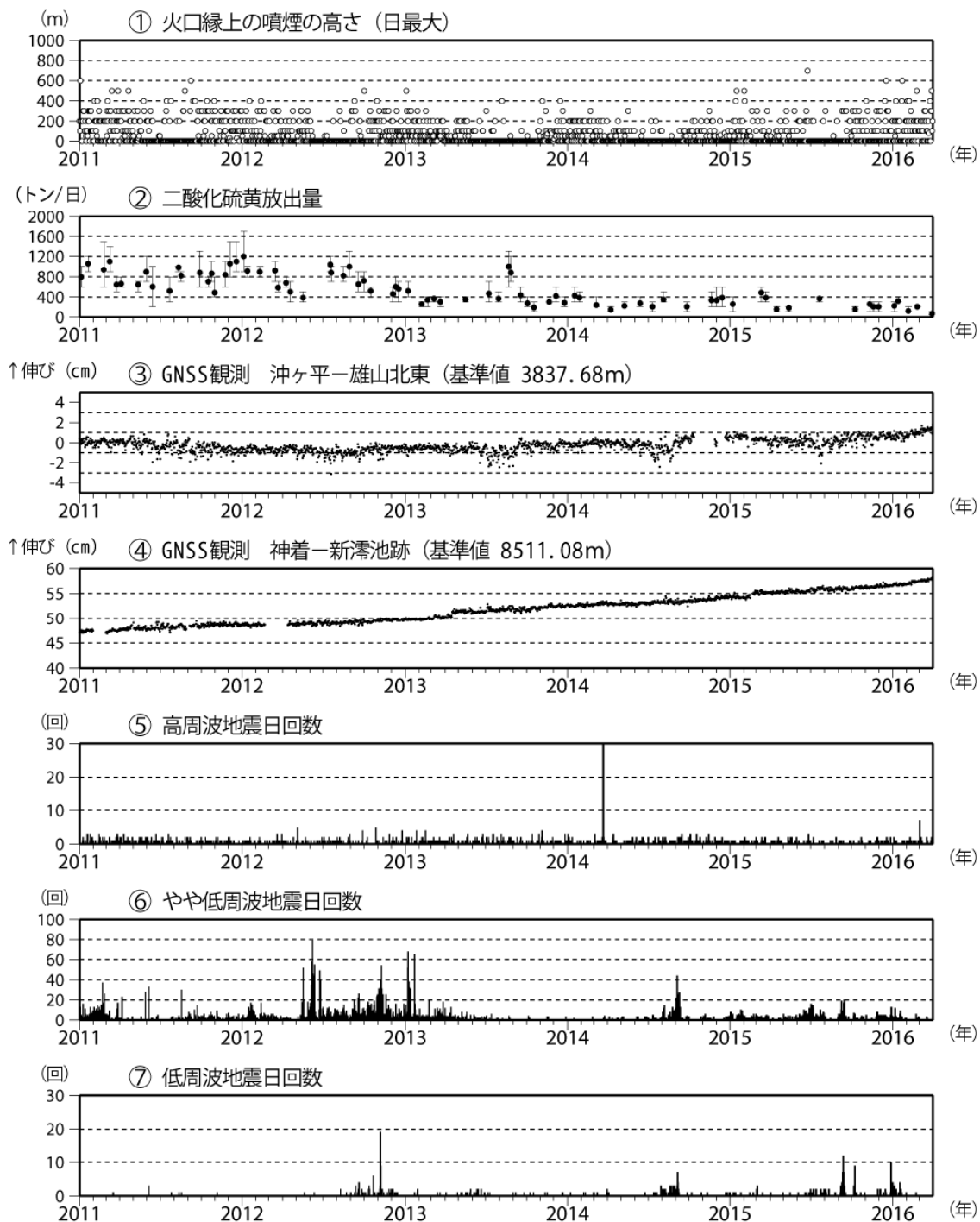
図5 三宅島 火山活動短期経過図(2011年1月1日~2016年3月31日)
