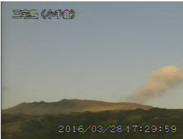
図 1 三宅島 山頂火口からの噴煙の状況 （3月28日、小手倉遠望カメラによる）
