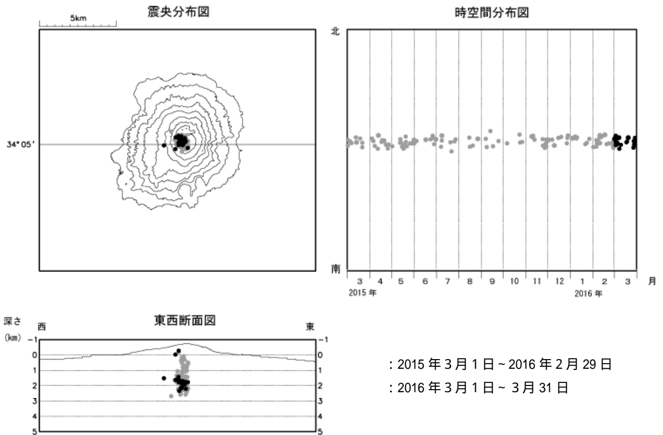
図7 三宅島 震源分布図(2015年3月1日~2016年3月31日) ・震源は山頂火口直下に分布しており、これまでと比べて特段の変化は認められません。
