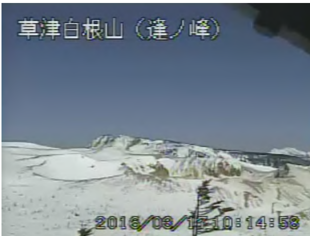
図 2 草津白根山 湯釜付近の状況
