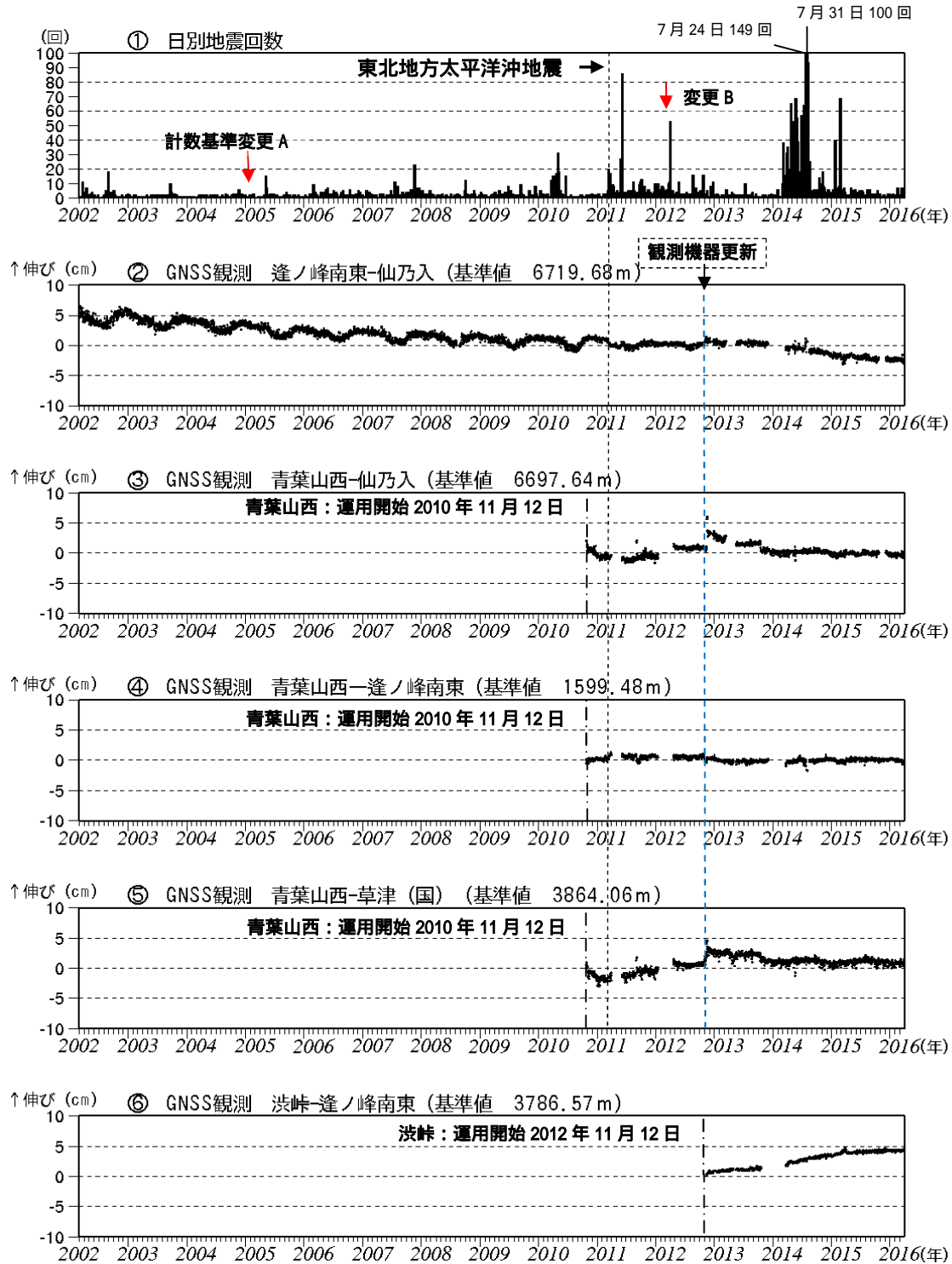
図5 草津白根山 火山活動経過図 (2002年3月1日~2016年3月31日)
