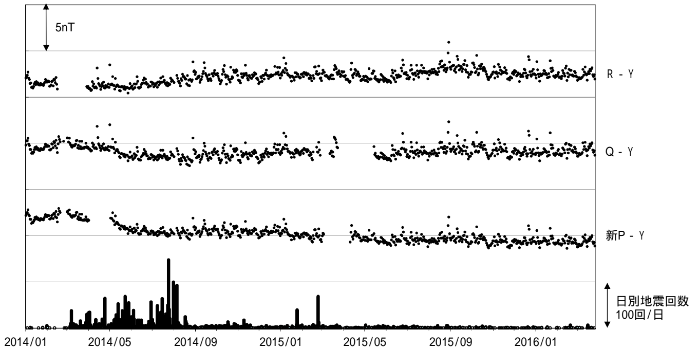
図 7 草津白根山 全磁力連続観測による全磁力値の変化及び日別地震回数 (2014 年 1 月～2016 年 3 月 25 日)
