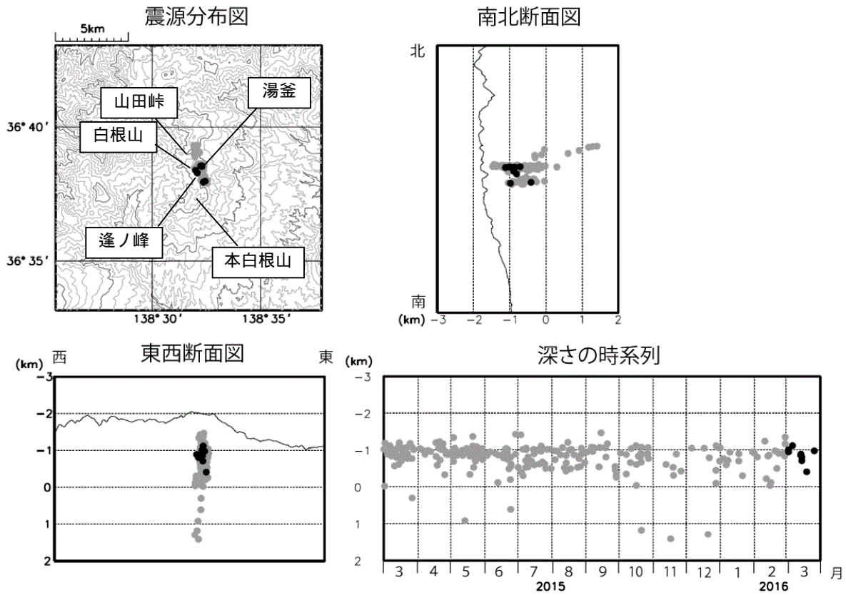
図3 草津白根山 震源分布図(2015年3月1日~2016年3月31日) : 2015年3月1日~2016年2月29日 : 2016年3月1日~3月31日
