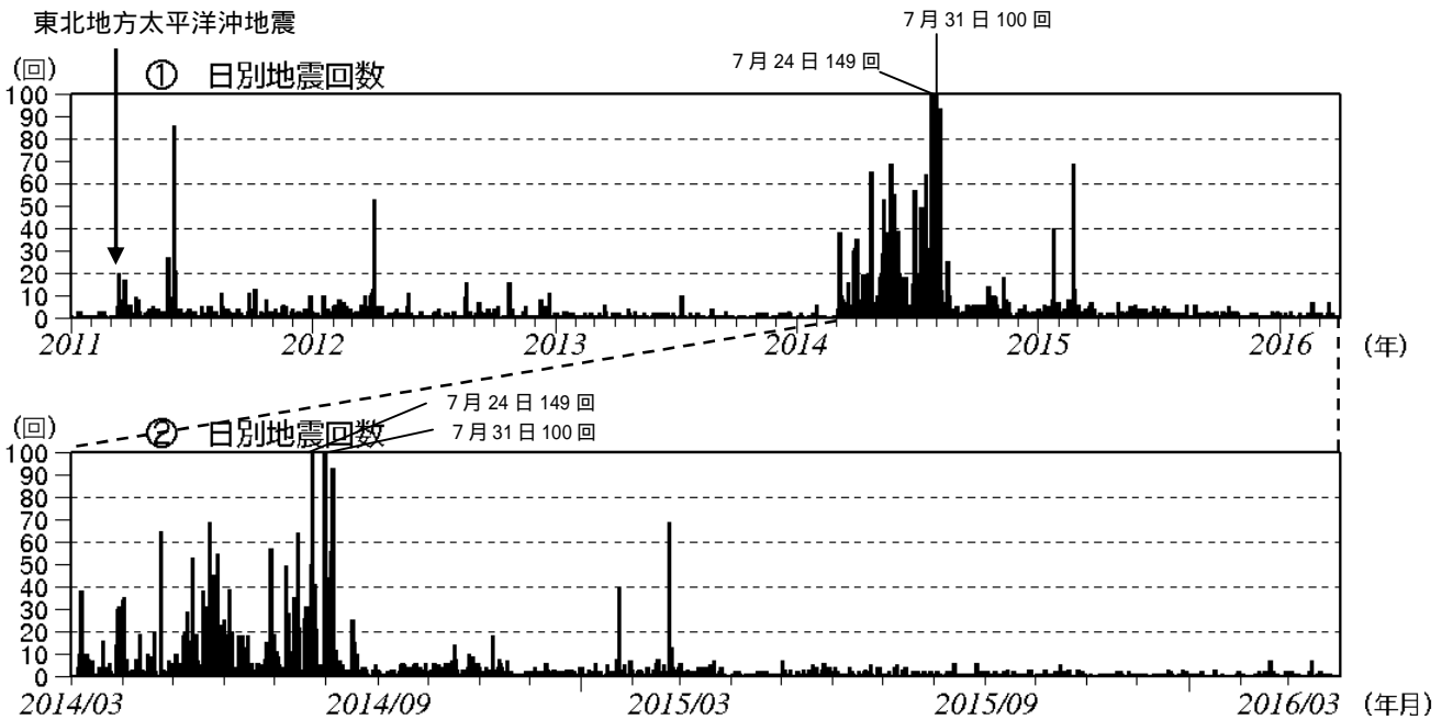
図4 草津白根山 日別地震回数(2011年1月1日~2016年3月31日)
