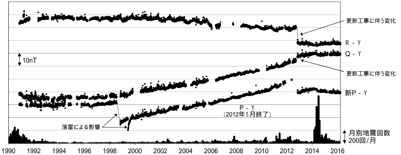
図 6 草津白根山 全磁力連続観測による全磁力値の変化及び月別地震回数 (1990 年～2016 年 3 月 25 日)
