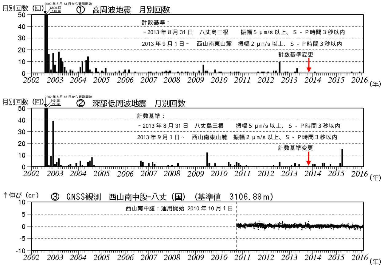
図2 八丈島 火山活動経過図(2002年8月13日~2016年2月29日)
