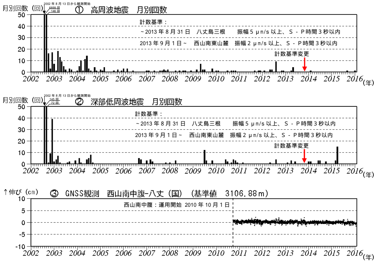
図2 八丈島 火山活動経過図(2002年8月13日~2016年1月31日)
