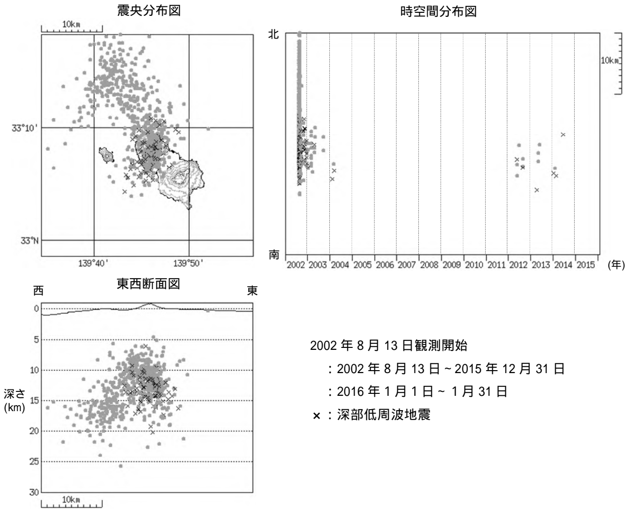
図3 八丈島 震源分布図(2002年8月13日~2016年1月31日) ・今期間、八丈島付近に震源が決定された高周波地震及び深部低周波地震はありませんでした。
