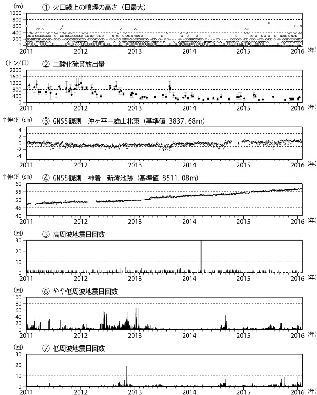
図6 三宅島 火山活動短期経過図(2011年1月1日～2016年1月31日)
