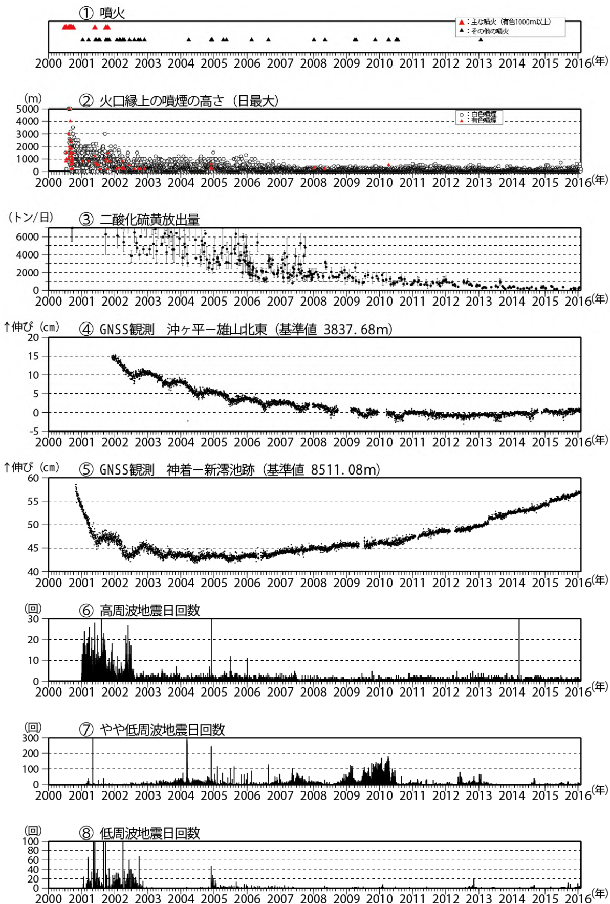
図5 三宅島 火山活動長期経過図 (2000年1月1日~2016年1月31日)
