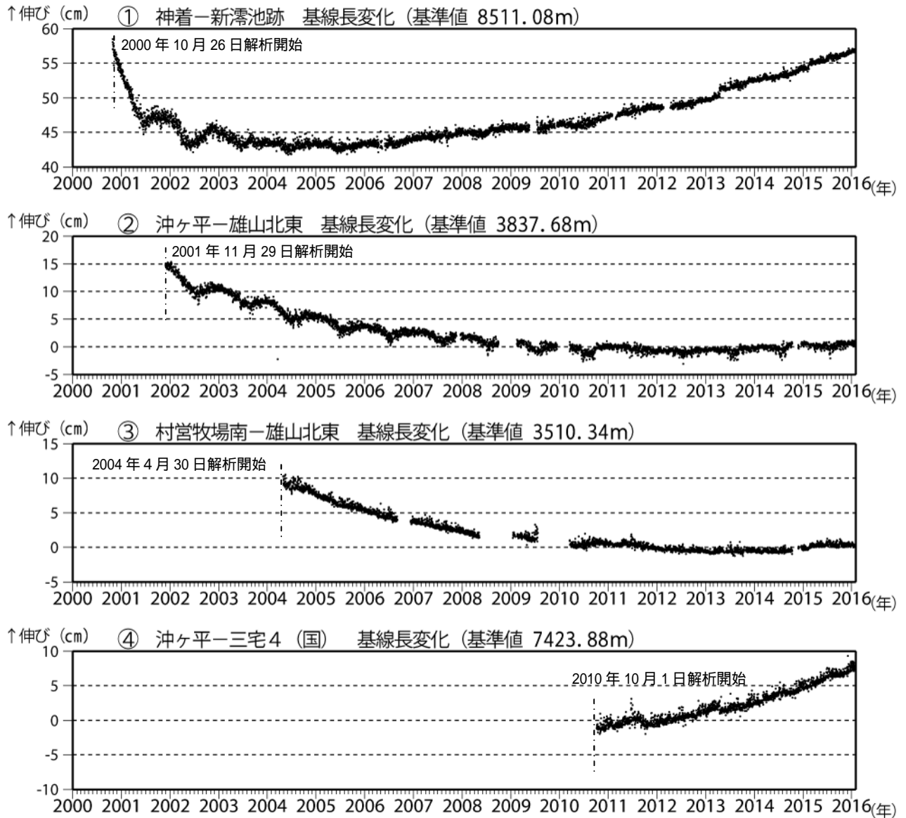
図7 三宅島 GNSS 連続観測結果 (2000年1月1日~2016年1月31日) (国): 国土地理院
