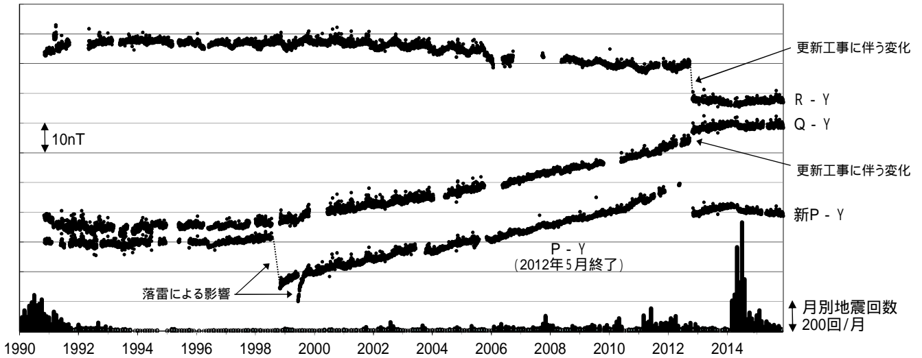
図 6 草津白根山 全磁力連続観測による全磁力値の変化及び月別地震回数（1990 年～2015 年 11 月 25 日）
