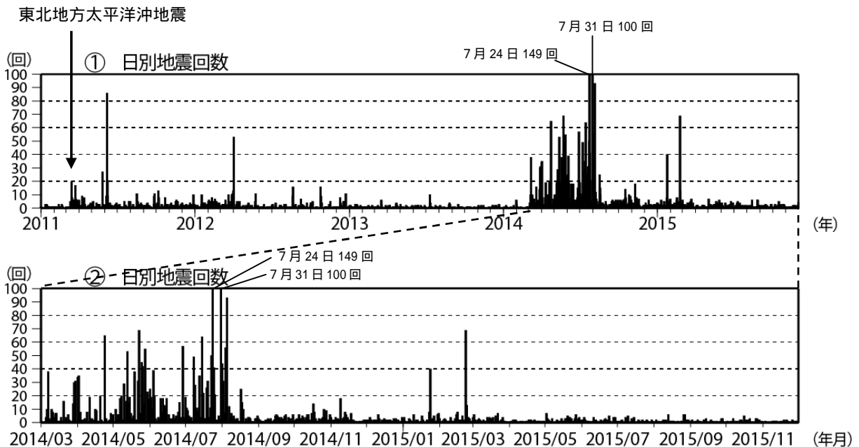
図4 草津白根山 日別地震回数（2011年1月1日～2015年11月30日） ・2014年3月上旬から湯釜付近及びその南側を震源とする火山性地震が増加しました。その後、消長を繰り返しながら多い状態が継続していましたが、2014年8月下旬以降は概ね少ない状態で経過しています。2015年1月と2月に一時的な火山性地震の増加がみられました。
