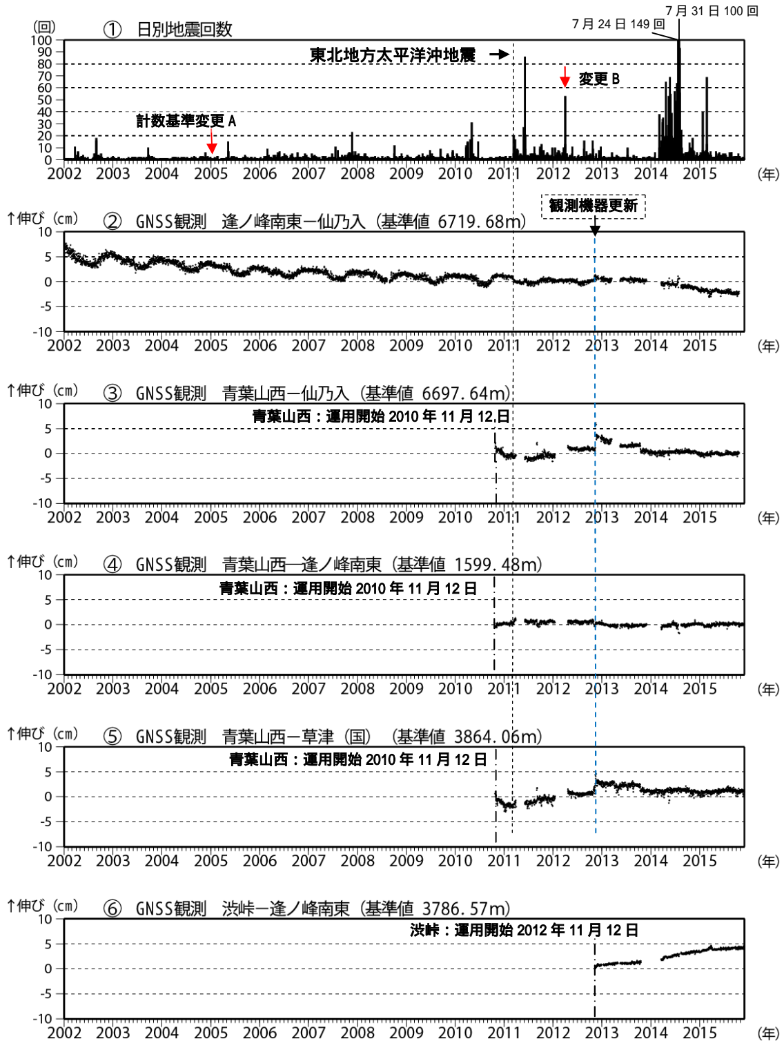
図5 草津白根山 火山活動経過図 (2002年1月1日~2015年11月30日)
