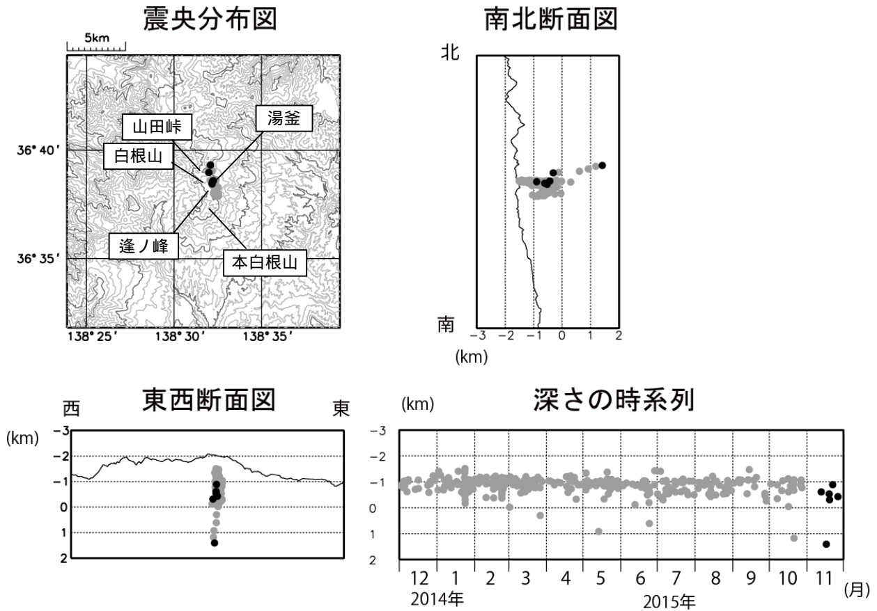
図3 草津白根山 震源分布図（2014年12月1日～2015年11月30日） : 2014年12月1日～2015年10月31日 : 2015年11月1日～11月30日
