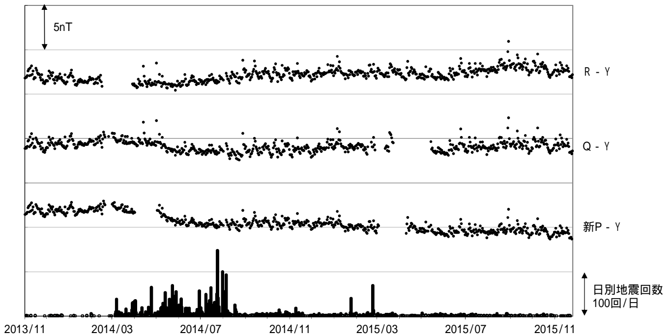
図 7 草津白根山 全磁力連続観測による全磁力値の変化及び日別地震回数（2013 年 11 月～2015 年 11 月 25 日）
