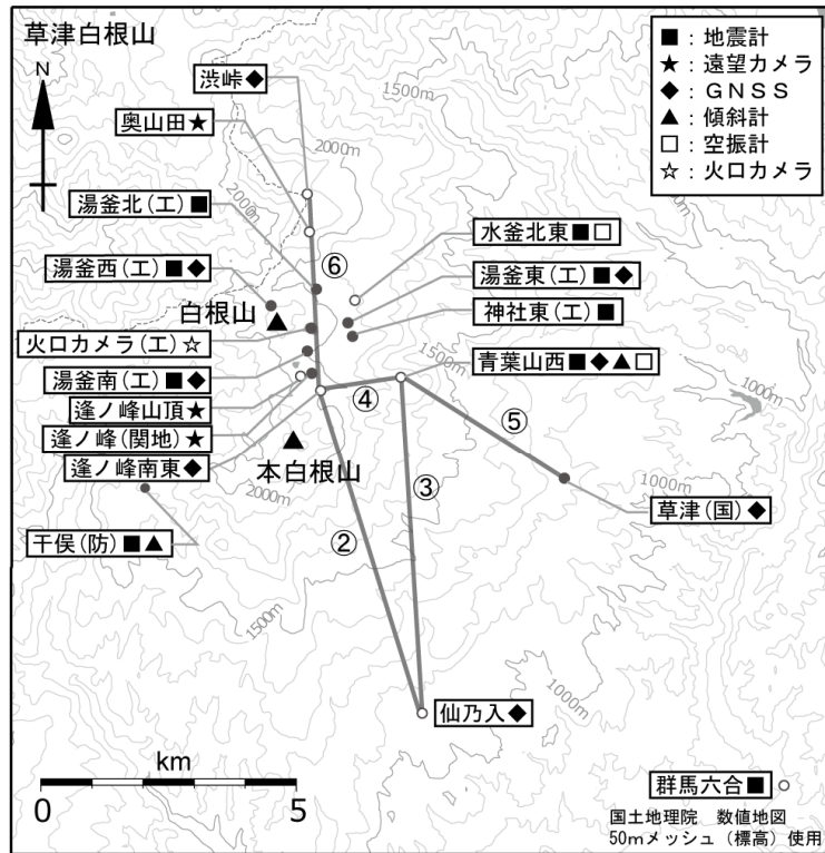
図 1 草津白根山 観測点配置図
