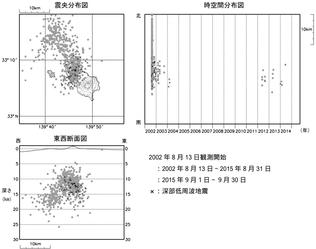
図3 八丈島 震源分布図(2002年8月13日~2015年9月30日) 今期間、八丈島付近に震源が決定された高周波地震及び深部低周波地震はありませんでした。
