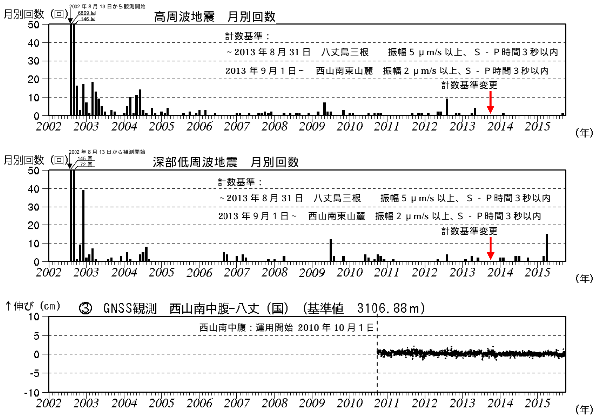
図2 八丈島 火山活動経過図(2002年8月13日~2015年9月30日)
