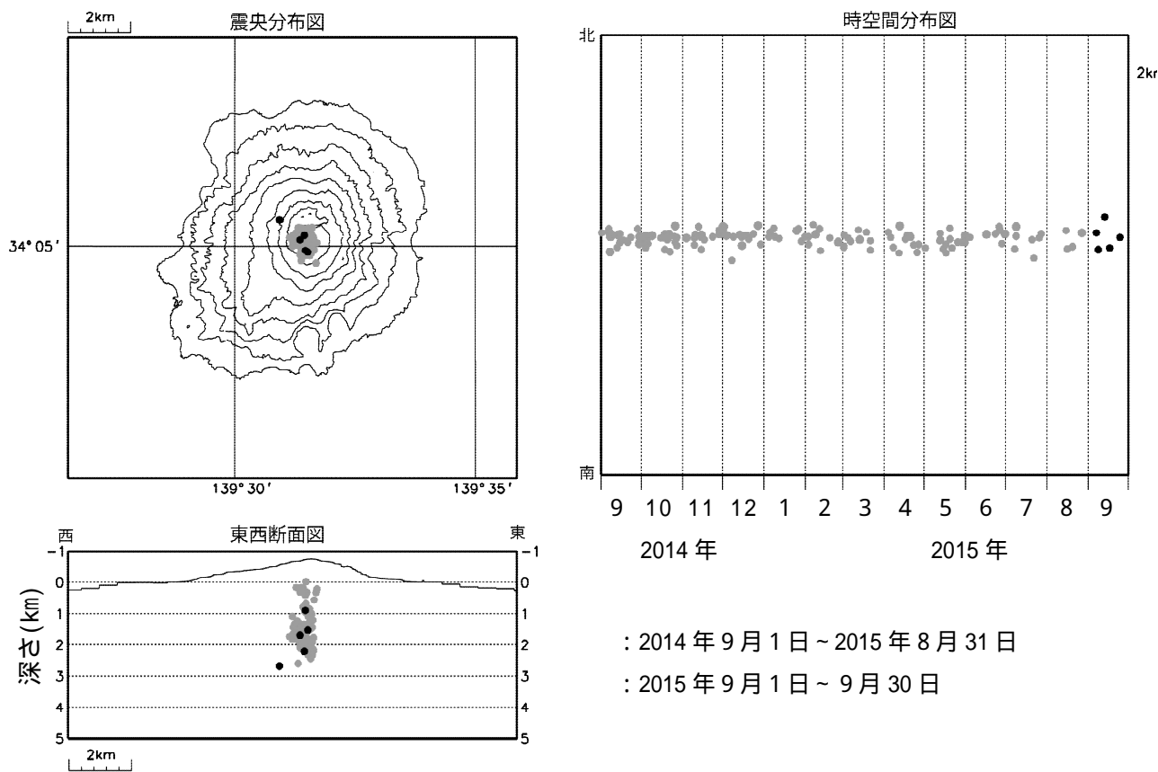
図 6 三宅島 震源分布図 (2014 年 9 月 1 日 ~ 2015 年 9 月 30 日) 震源は山頂火口直下に分布しており、これまでと比べて特段の変化は認められません。
