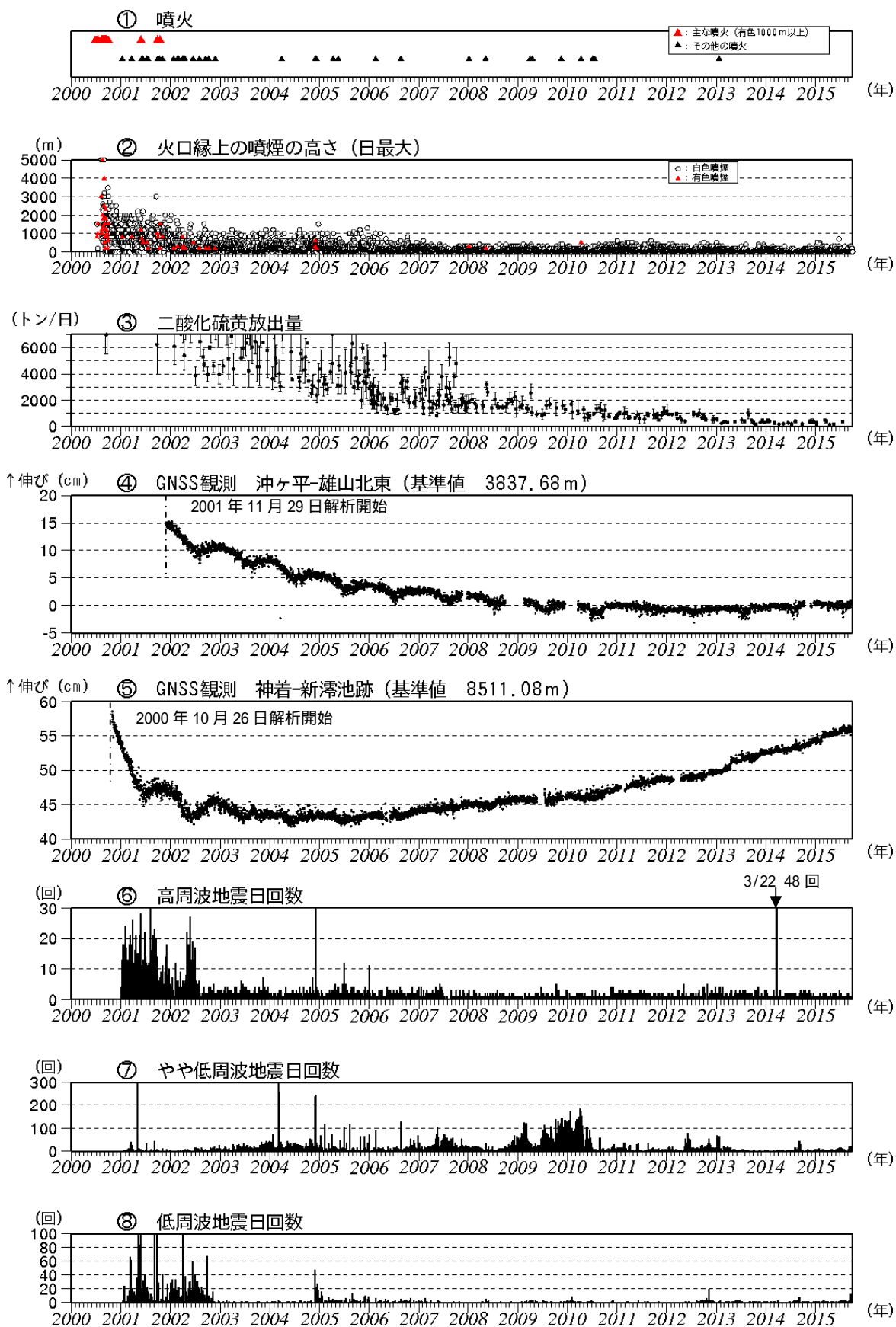
図4 三宅島 火山活動経過図（2000年1月1日～2015年9月30日）
