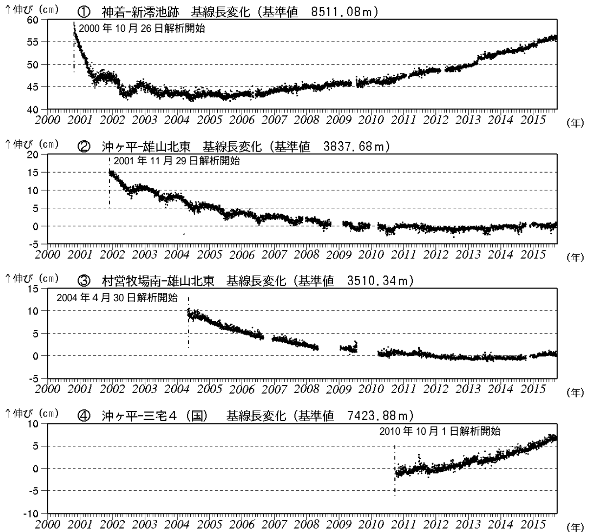
図5 三宅島 GNSS 連続観測結果(2000年1月1日～2015年9月30日) (国): 国土地理院 ・基線 ~ は図8(観測点配置図)の ~ にそれぞれ対応します。 ・グラフの空白部分は欠測を示します。 ・2010年10月以降のデータについては、電離層の影響を補正する等、解析方法を改良しています。
