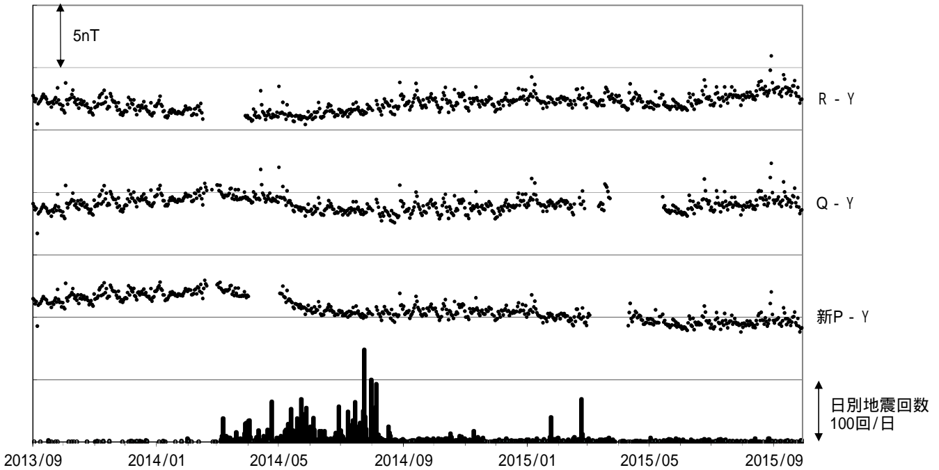
図7 草津白根山 全磁力連続観測による全磁力値の変化及び日別地震回数(2013年8月～2015年9月28日) 連続観測点P、Q、Rおよび新Pにおける八ヶ岳地球電磁気観測所(東京大学)(Y)との全磁力の夜間日 平均值差。最下段は草津白根山で観測された日別地震回数を示しています。 全磁力連続観測で、2014年5月頃からみられていた湯釜近傍地下の温度上昇を示すと考えられる 変化は、2014年7月以降停滞しています。グラフの空白部分は欠測を示します。
