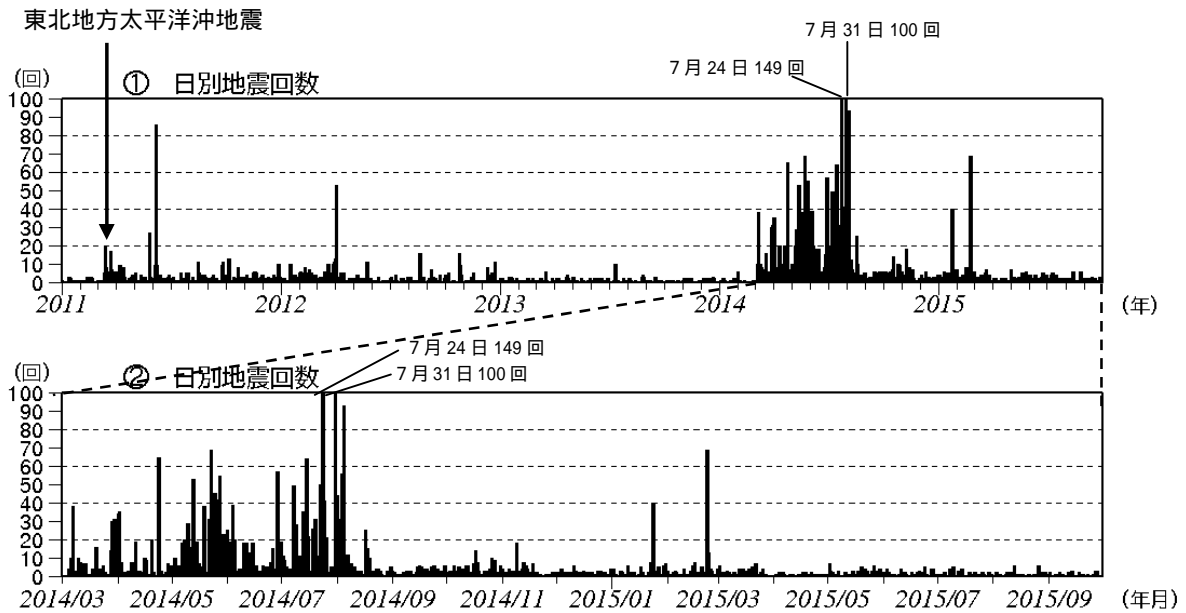
図2 草津白根山 日別地震回数(2011年1月1日~2015年9月30日)
