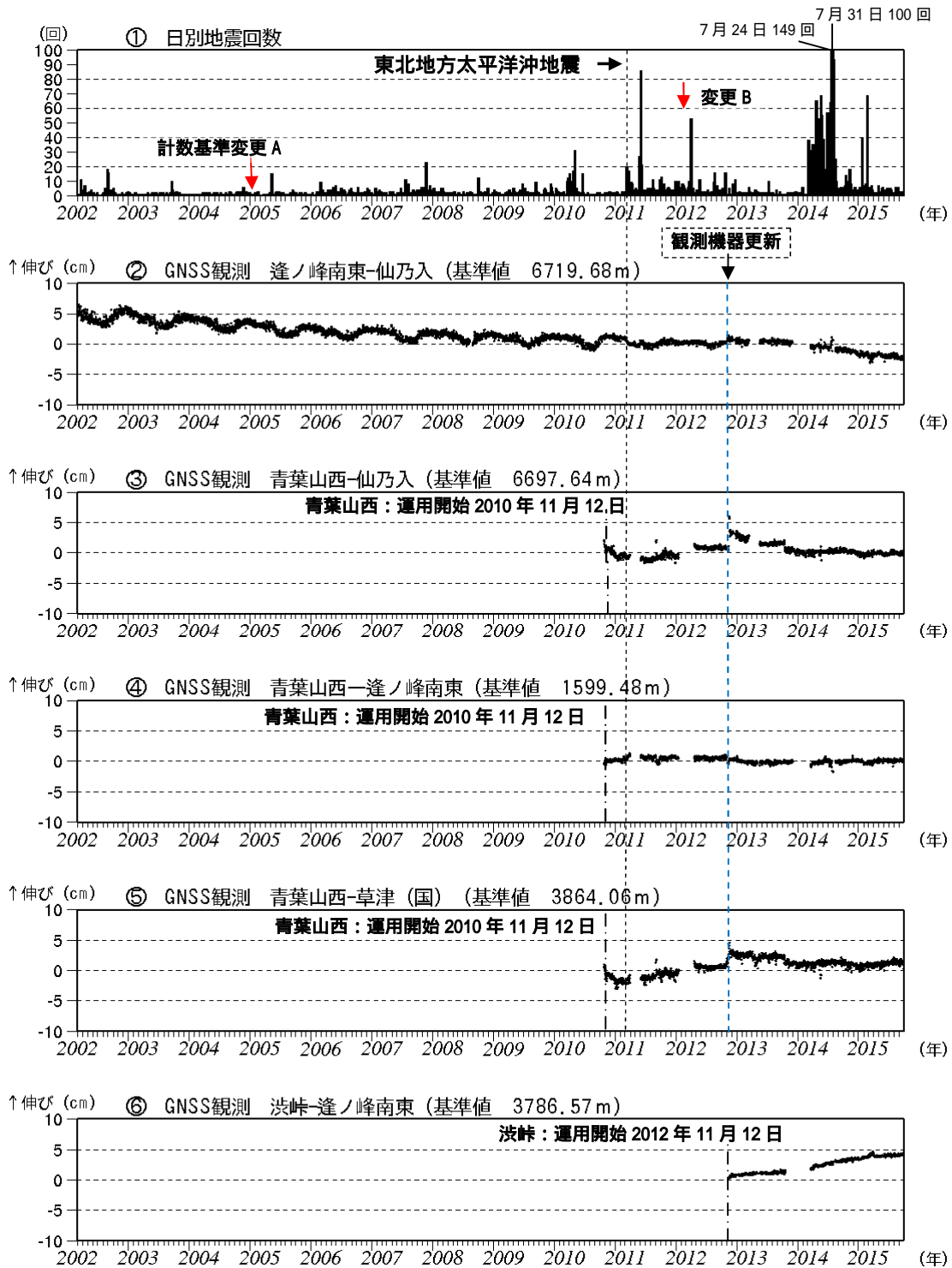
図3 草津白根山 火山活動経過図 (2002年1月1日~2015年9月30日)
