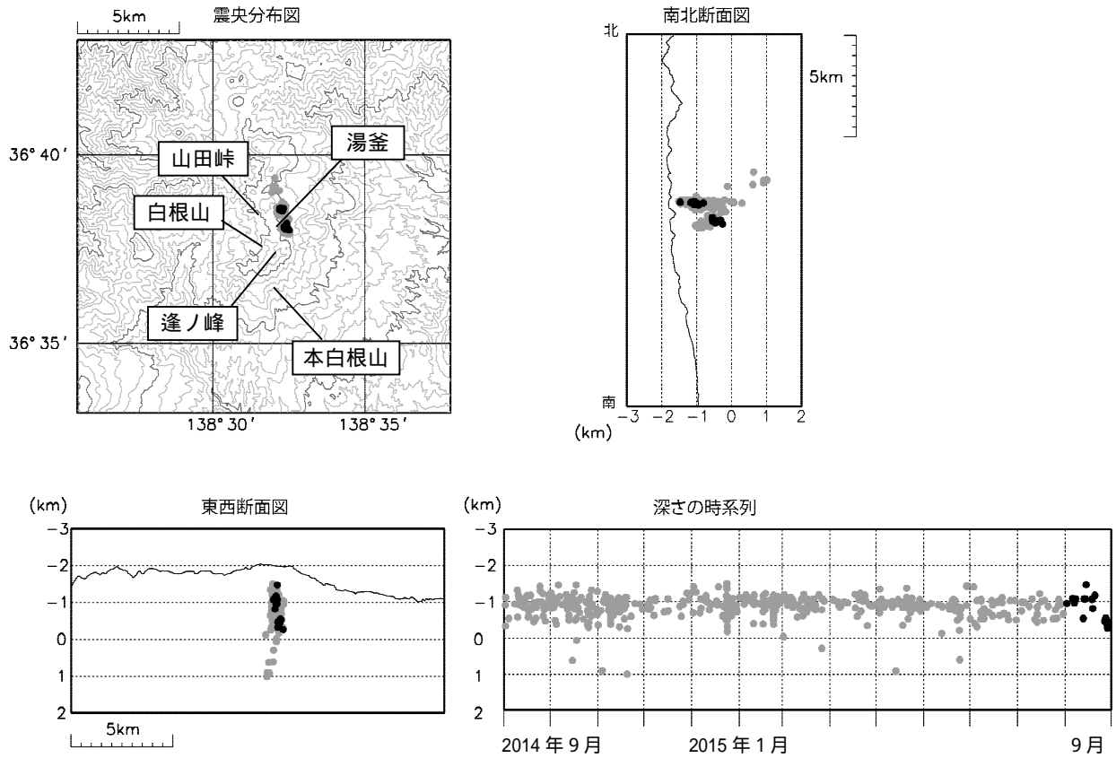
図1 草津白根山 震源分布図(2014年9月1日~2015年9月30日)
