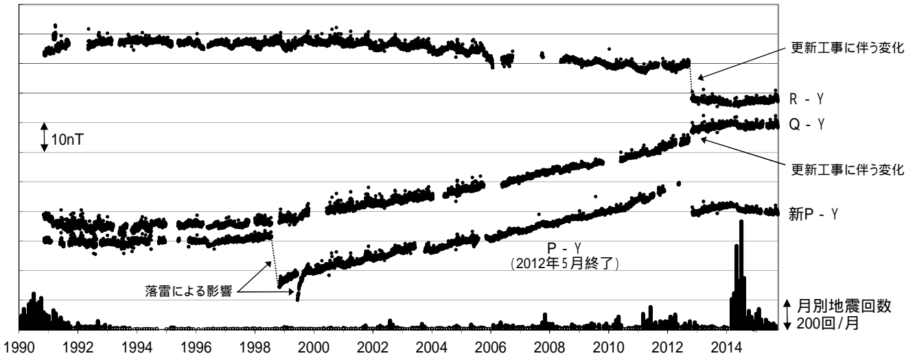
図6 草津白根山 全磁力連続観測による全磁力値の変化及び月別地震回数(1990年～2015年9月28日) 連続観測点P、Q、Rおよび新Pにおける八ヶ岳地球電磁気観測所(東京大学)(Y)との全磁力の夜間日 平均值差。最下段は草津白根山で観測された月別地震回数を示しています。全磁力連続観測で、2014 年5月頃からみられていた湯釜近傍地下の温度上昇を示すと考えられる変化は、2014年7月以降停 滞しています。グラフの空白部分は欠測を示します。
