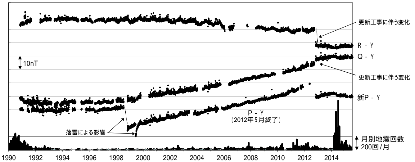
図 6 草津白根山 全磁力連続観測による全磁力値の変化及び月別地震回数（1990 年～2015 年 7 月 26 日）連続観測点 P、Q、R および新 P における八ヶ岳地球電磁気観測所（東京大学）（Y）との全磁力の夜間日平均値差。最下段は草津白根山で観測された月別地震回数を示しています。全磁力連続観測で、2014 年 5 月頃からみられていた湯釜近傍地下の温度上昇を示すと考えられる変化は、2014 年 7 月以降停滞しています。グラフの空白部分は欠測を示します。
