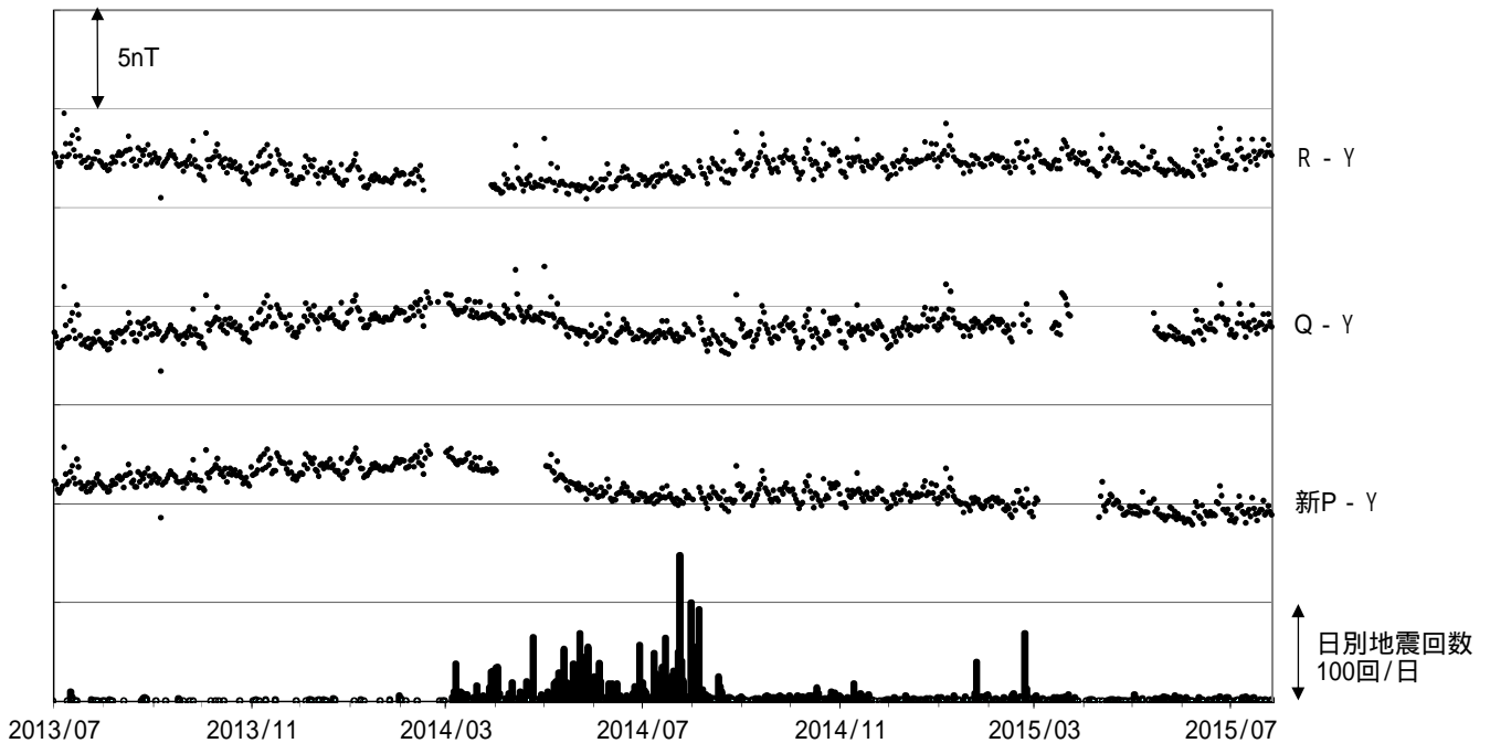
図 7 草津白根山 全磁力連続観測による全磁力値の変化及び日別地震回数（2013 年 7 月～2015 年 7 月 26 日）連続観測点 P、Q、R および新 P における八ヶ岳地球電磁気観測所（東京大学）（Y）との全磁力の夜間日平均値差。最下段は草津白根山で観測された日別地震回数を示しています。全磁力連続観測で、2014 年 5 月頃からみられていた湯釜近傍地下の温度上昇を示すと考えられる変化は、2014 年 7 月以降停滞しています。グラフの空白部分は欠測を示します。
