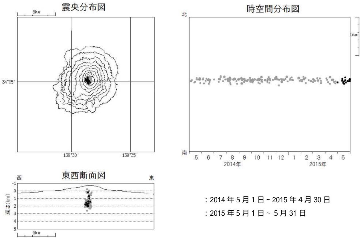
図6 三宅島 震源分布図(2014年5月1日~2015年5月31日)
