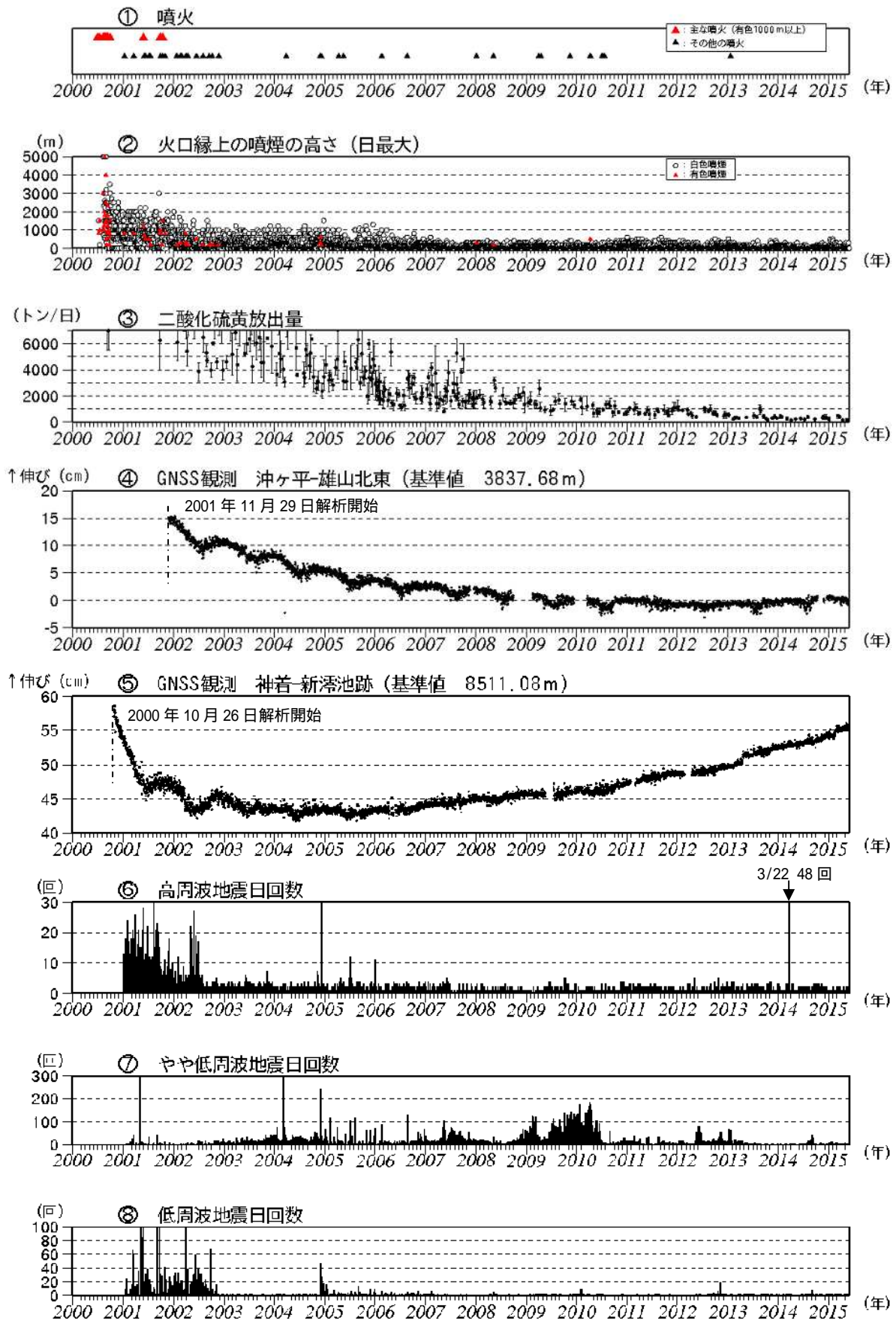
図4 三宅島 火山活動経過図（2000年1月1日～2015年5月31日）
