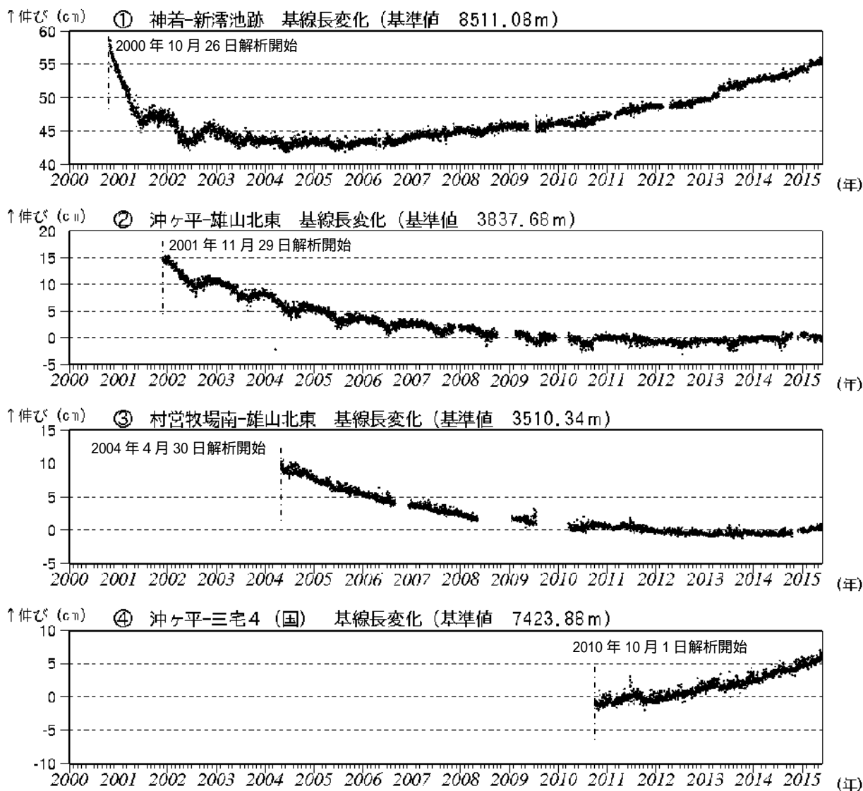
図5 三宅島 GNSS 連続観測結果(2000年1月1日~2015年5月31日) (国): 国土地理院 ・ 基線 ~ は図8(観測点配置図)の ~ にそれぞれ対応します。 ・ グラフの空白部分は欠測を示します。 ・ 2010年10月以降のデータについては、電離層の影響を補正する等、解析方法を改良しています。
