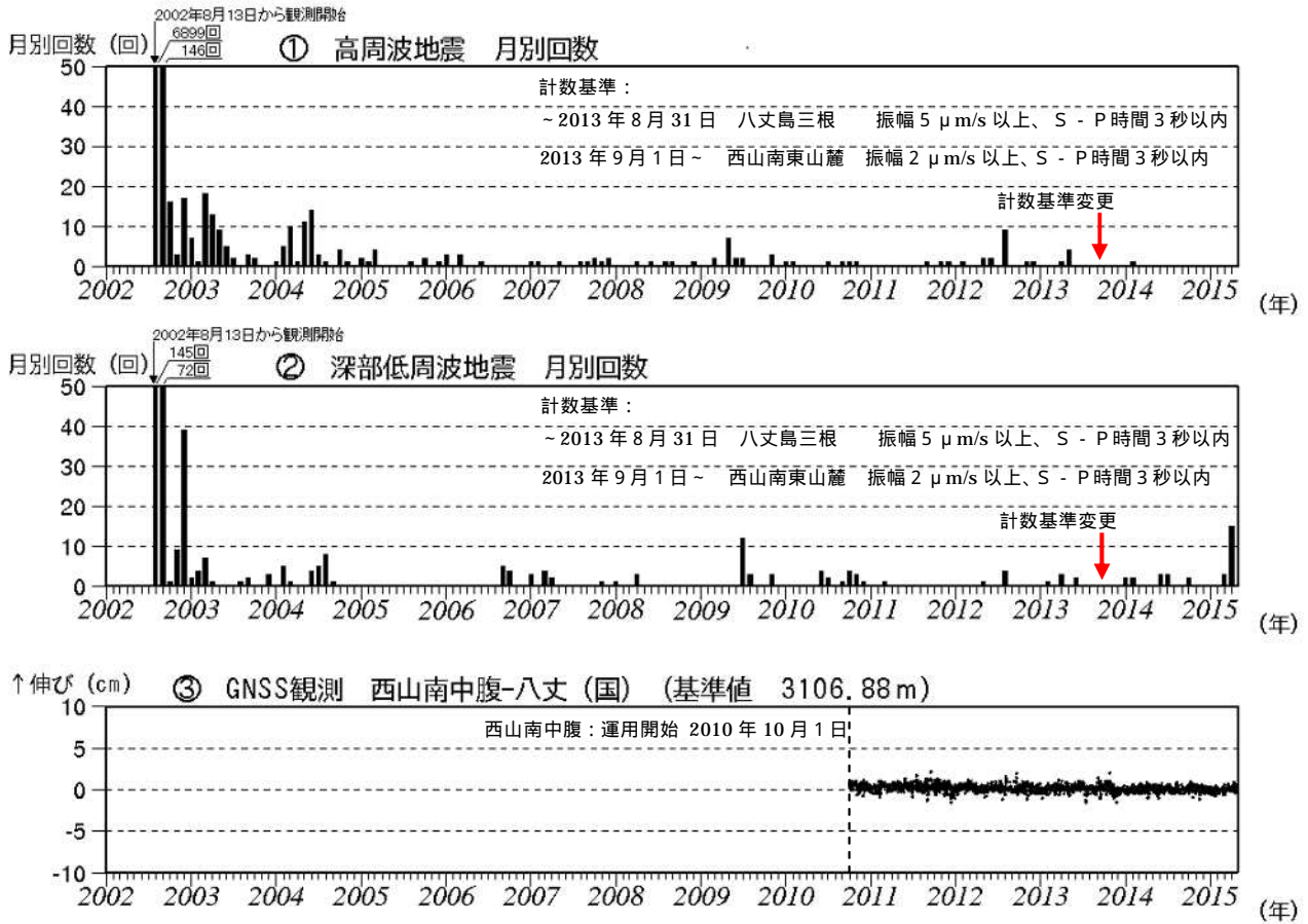
図2 八丈島 火山活動経過図(2002年8月13日~2015年4月30日)
