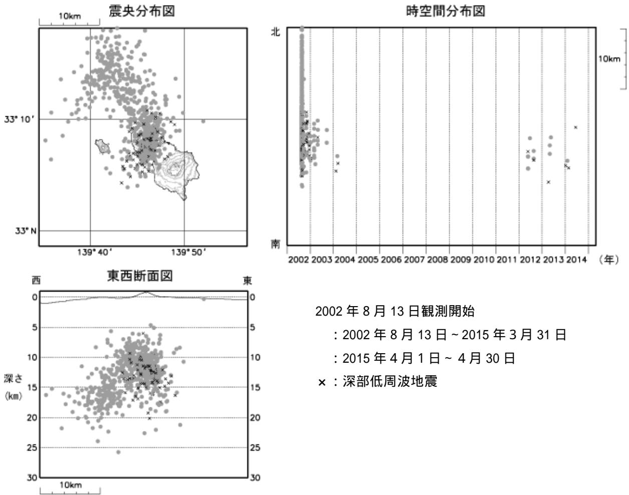
図3 八丈島 震源分布図(2002年8月13日~2015年4月30日) 今期間、八丈島付近に震源が決定された高周波地震及び深部低周波地震はありませんでした。
