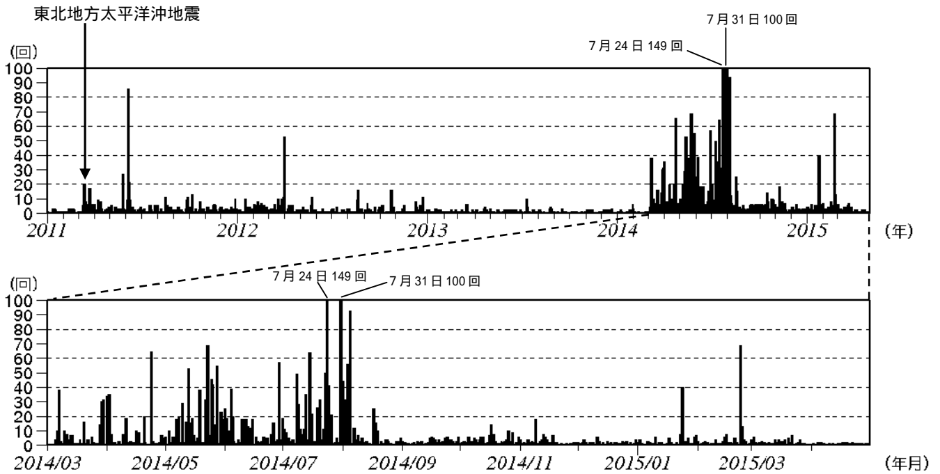
図 2 草津白根山 日別地震回数 (2011 年 1 月 1 日 ~ 2015 年 4 月 30 日)
