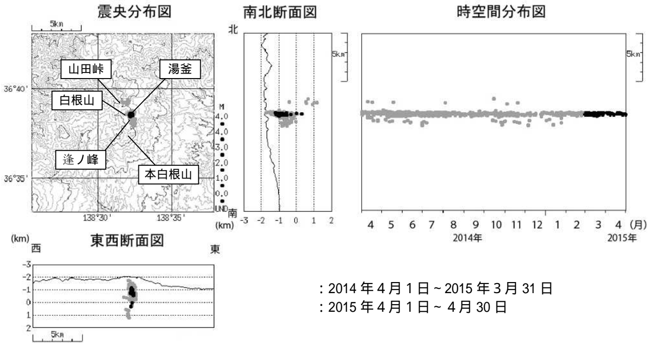
図 1 草津白根山 震源分布図 (2014 年 4 月 1 日 ~ 2015 年 4 月 30 日)
