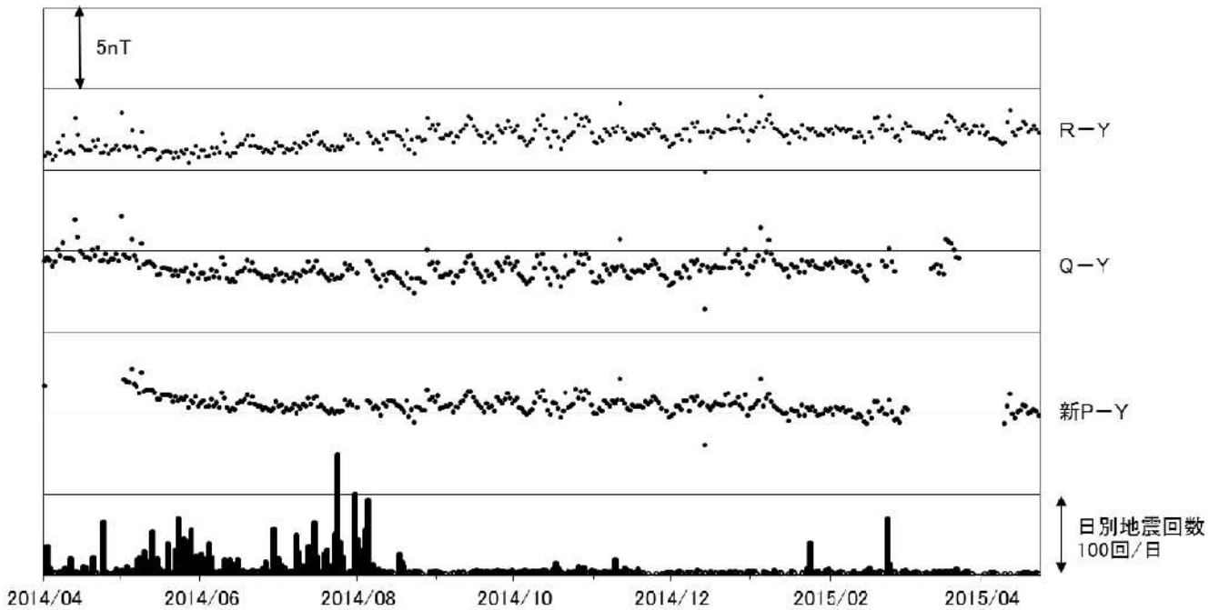
図 9 草津白根山 全磁力連続観測による全磁力値の変化及び日別地震回数（2014 年 3 月～2015 年 4 月 23 日） 連続観測点 P、Q、R および新 P における八ヶ岳地球電磁気観測所（東京大学）(Y)との全磁力の夜間日平均値差。最下段は草津白根山で観測された日別地震回数を示しています。
