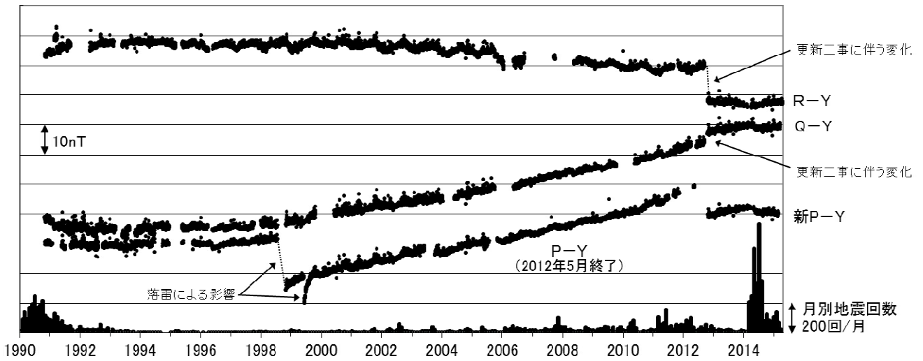
図 8 草津白根山 全磁力連続観測による全磁力値の変化及び月別地震回数（1990 年～2015 年 4 月 23 日） 連続観測点 P、Q、R および新 P における八ヶ岳地球電磁気観測所（東京大学）(Y)との全磁力の夜間日平均値差。最下段は草津白根山で観測された月別地震回数を示しています。
