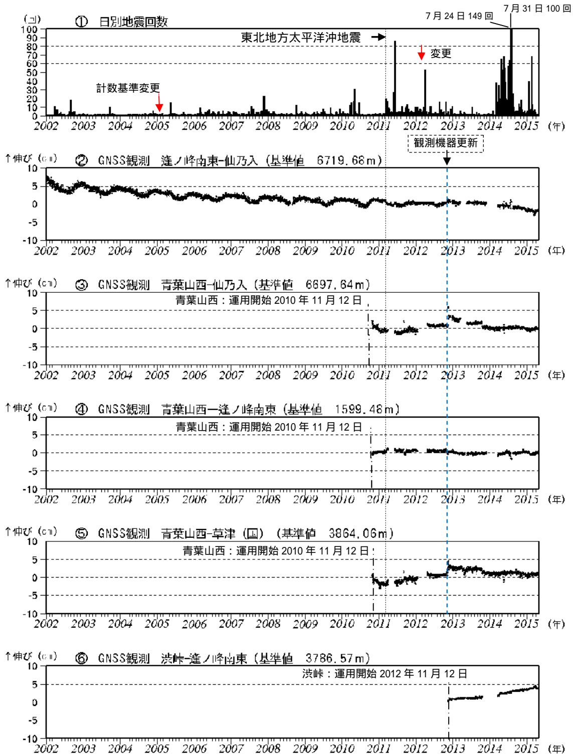
図3 草津白根山 火山活動経過図 (2002年1月1日~2015年4月30日)
