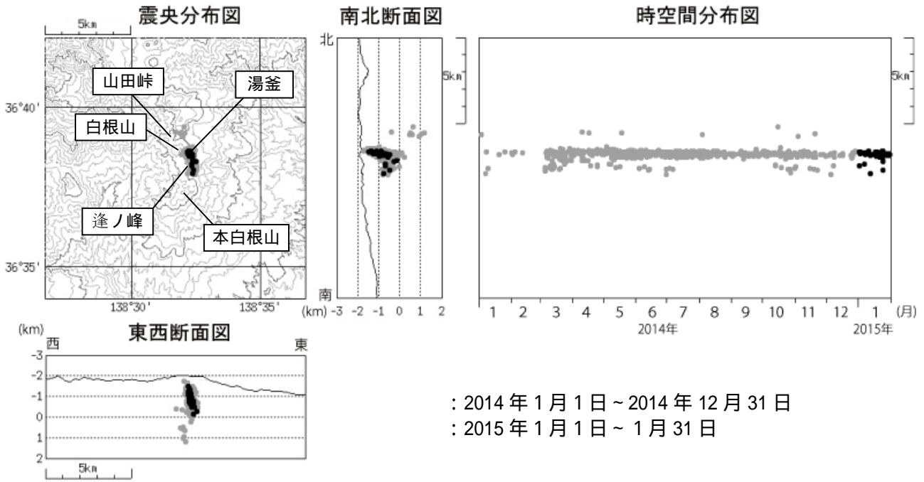
図 1 草津白根山 震源分布図 (2014 年 1 月 1 日 ~ 2015 年 1 月 31 日)
