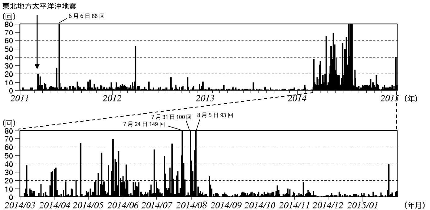
図 2 草津白根山 日別地震回数 (2011 年 1 月 1 日 ~ 2015 年 1 月 31 日)
