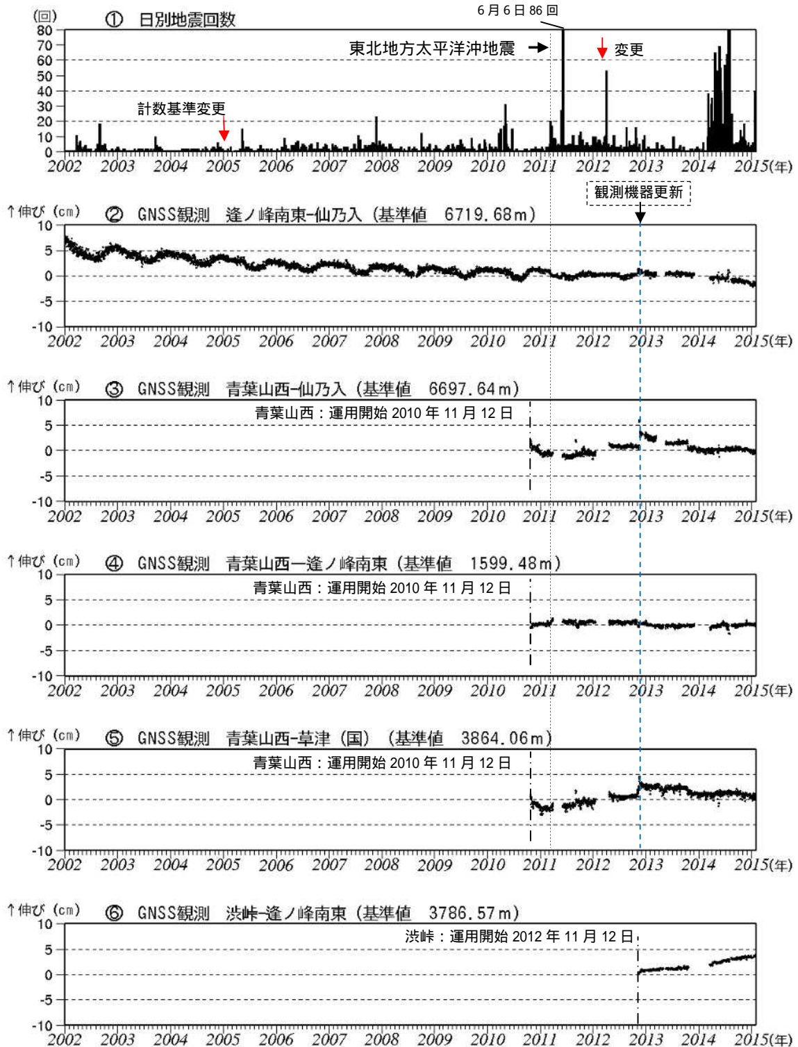
図3 草津白根山 火山活動経過図 (2002年1月1日~2015年1月31日)
