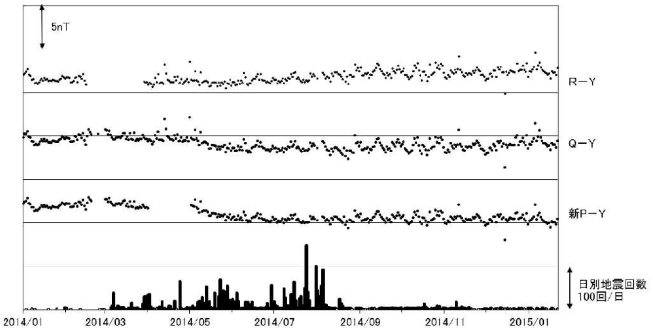
図 7 草津白根山 全磁力連続観測による全磁力値の変化及び日別地震回数(2014年1月~2015年1月21日) 連続観測点P、Q、Rおよび新Pにおける八ヶ岳地球電磁気観測所(東京大学)(Y)との全磁力の夜間日平均値差。最下段は草津白根山で観測された日別地震回数を示しています。
