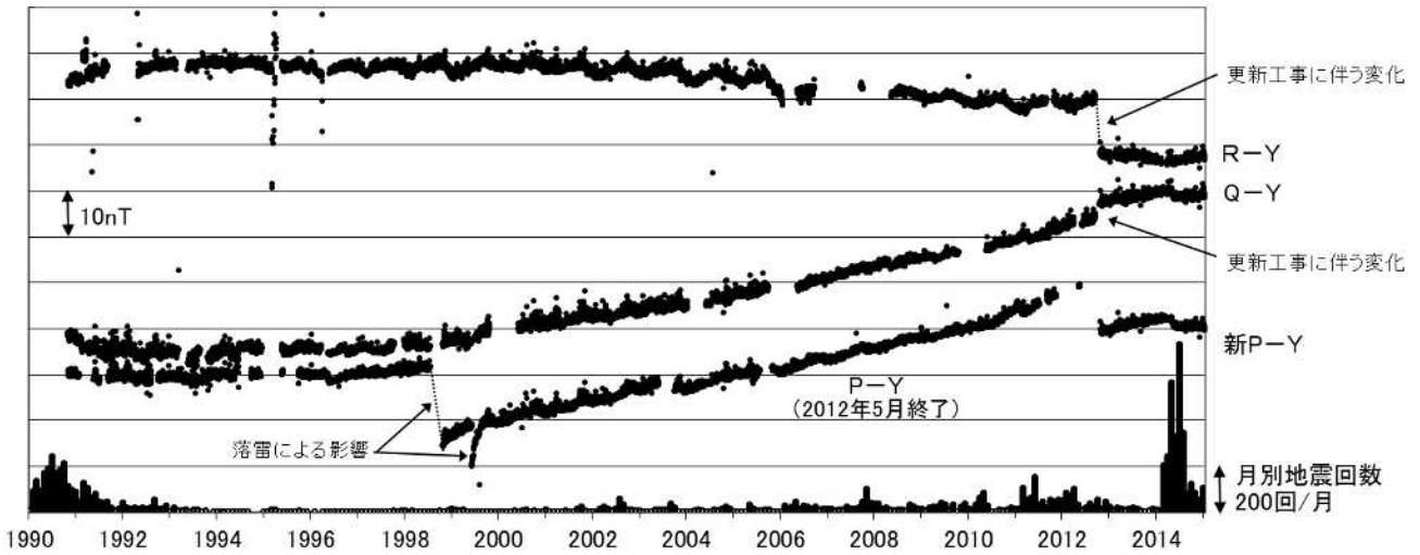
図 6 草津白根山 全磁力連続観測による全磁力値の変化及び月別地震回数(1990年~2015年1月21日) 連続観測点P、Q、Rおよび新Pにおける八ヶ岳地球電磁気観測所(東京大学)(Y)との全磁力の夜間日平均値差。最下段は草津白根山で観測された月別地震回数を示しています。
