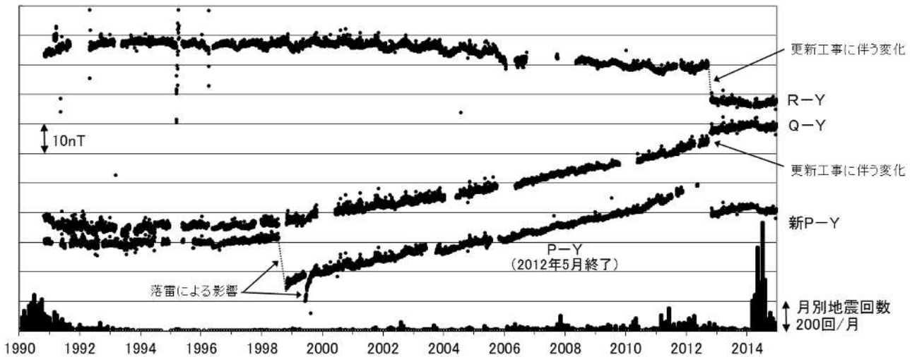
図9 草津白根山 全磁力連続観測による全磁力値の変化及び月別地震回数(1990年~2014年12月25日) 連続観測点P、Q、Rおよび新Pにおける八ヶ岳地球電磁気観測所(東京大学)(Y)との全磁力の夜間日平均値差。最下段は草津白根山で観測された月別地震回数を示しています。
