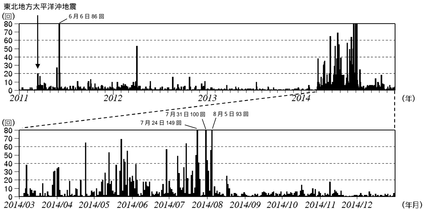
図2 草津白根山 日別地震回数（2011年1月1日～2014年12月31日）
