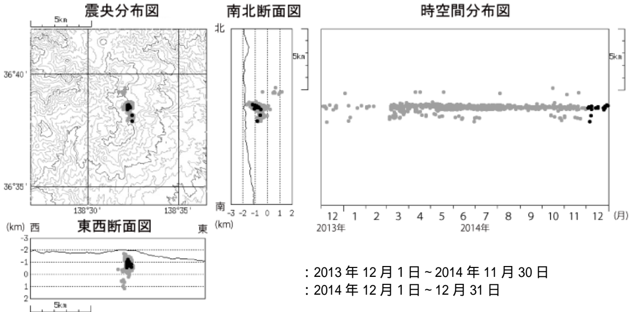
図1 草津白根山 震源分布図（2013年12月1日～2014年12月31日）
