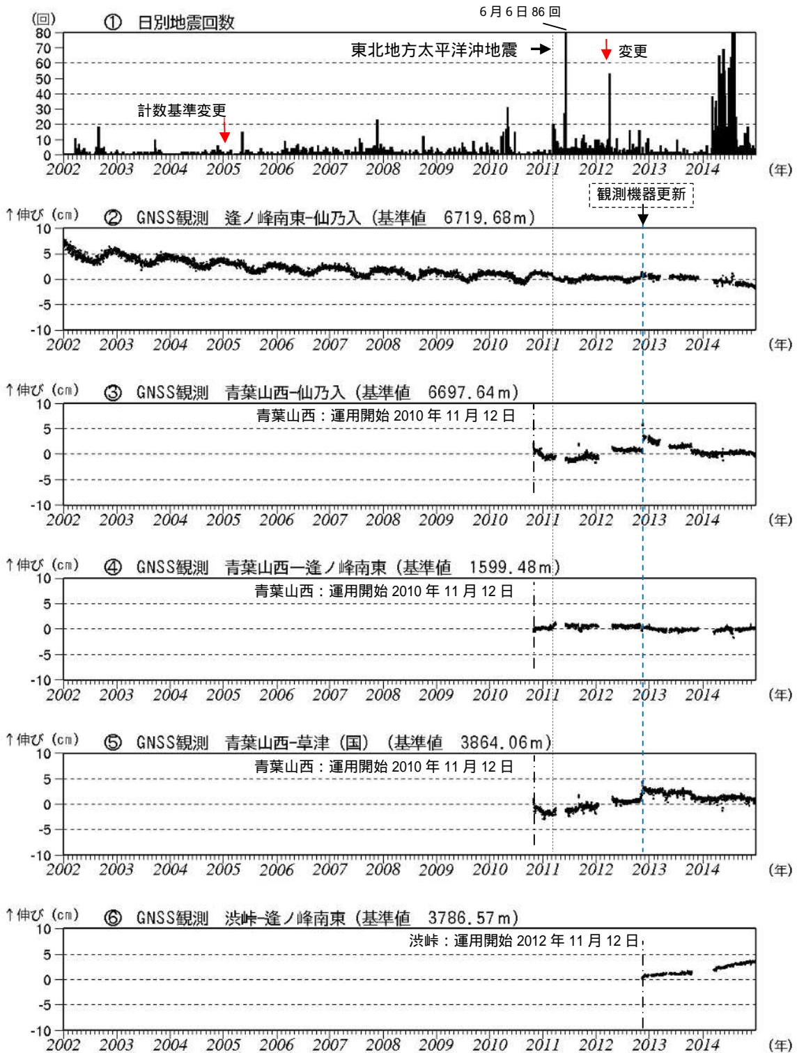
図3 草津白根山 火山活動経過図 (2002年1月1日~2014年12月31日)
