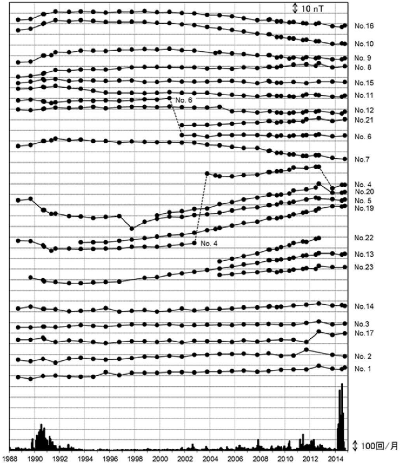
図8 草津白根山 全磁力繰り返し観測による全磁力値の変化（1988年9月～2014年10月）
