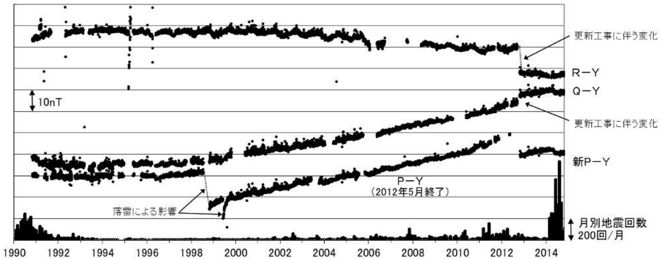
図6 草津白根山 全磁力連続観測による全磁力値の変化及び月別地震回数(1990年～2014年10月26日) 連続観測点P、Q、Rおよび新Pにおける八ヶ岳地球電磁気観測所(東京大学)(Y)との全磁力の夜間日平均値差。最下段は草津白根山で観測された月別地震回数を示しています。
