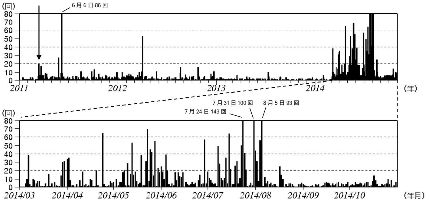
図2 草津白根山 日別地震回数（2011年1月1日～2014年10月31日）
