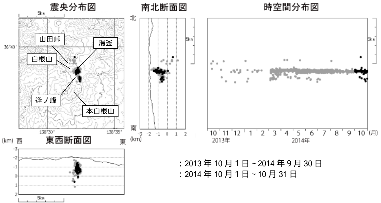
図1 草津白根山 震源分布図（2013年10月1日～2014年10月31日）
