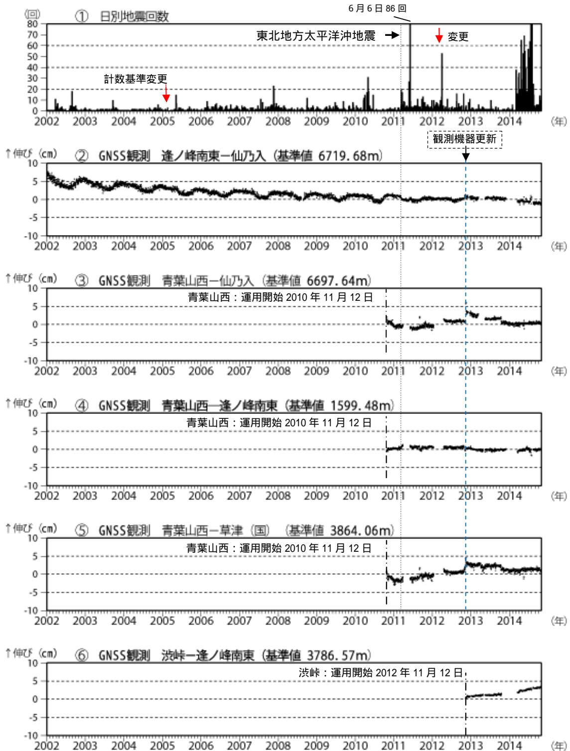
図3 草津白根山 火山活動経過図（2002年1月1日～2014年10月31日）
