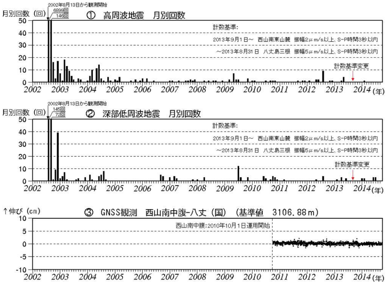
図2 八丈島 火山活動経過図(2002年8月13日～2014年9月30日)
