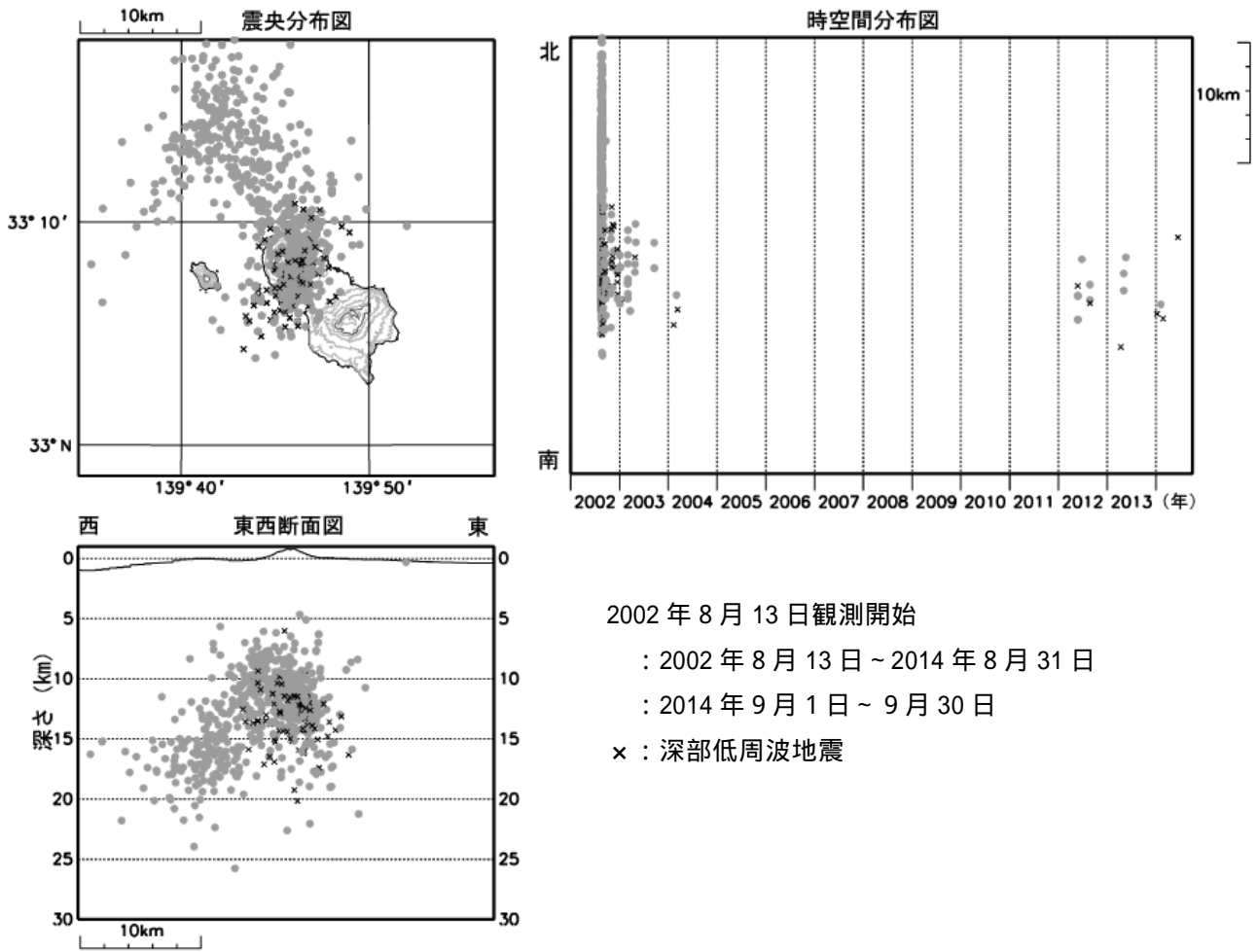
図3 八丈島 震源分布図(2002年8月13日～2014年9月30日) 今期間、八丈島付近に震源が決定された高周波地震及び深部低周波地震はありませんでした。
