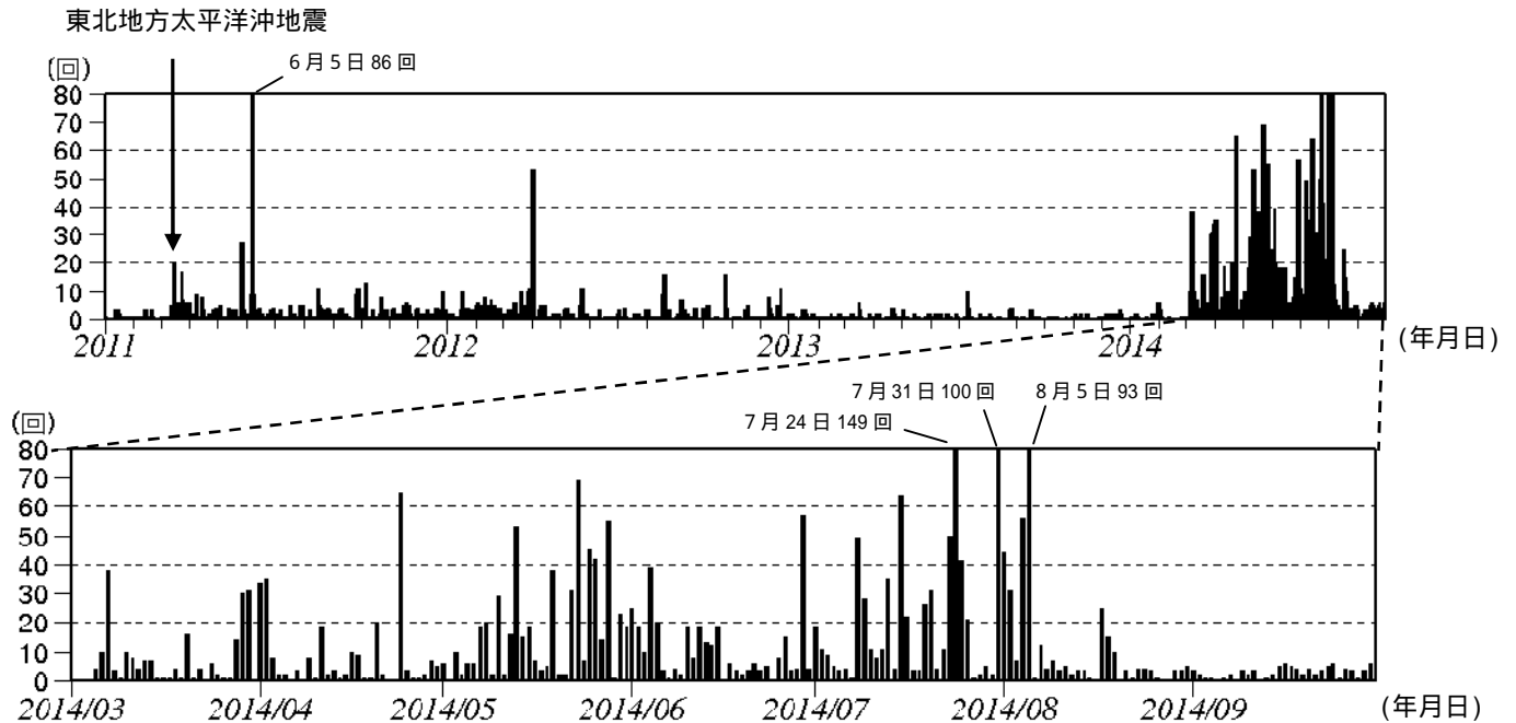
図2 草津白根山 日別地震回数(2011年1月1日~2014年9月30日)
