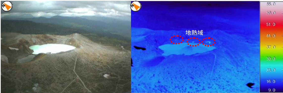
2014年6月23日15時25分 湯釜火口の南西上空から撮影 図6 草津白根山 湯釜火口周辺の状況及び地表面温度分布 湯釜の湖面に硫黄の浮遊物が認められました。 赤線内が高温領域を示しています。
