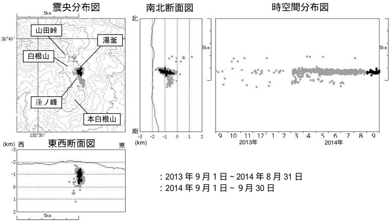
図1 草津白根山 震源分布図(2013年9月1日~2014年9月30日)
