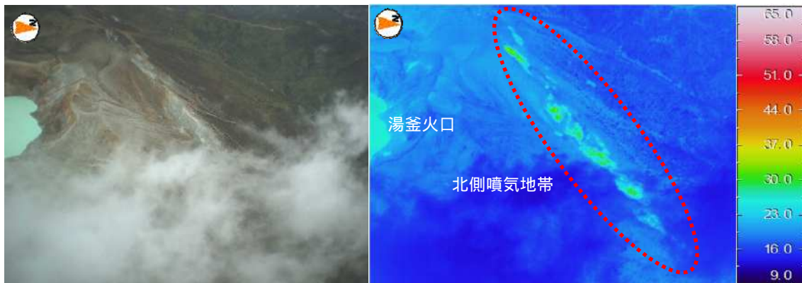
2014年9月24日10時26分 湯釜火口の北東上空から撮影
