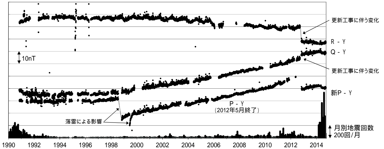
図 8 草津白根山 全磁力連続観測による全磁力値の変化及び月別地震回数(1990年~2014年9月24日) 連続観測点 P、Q、R および新 P における八ヶ岳地球電磁気観測所(東京大学)(Y)との全磁力の夜間日平均値差。最下段は草津白根山で観測された月別地震回数を示しています。
