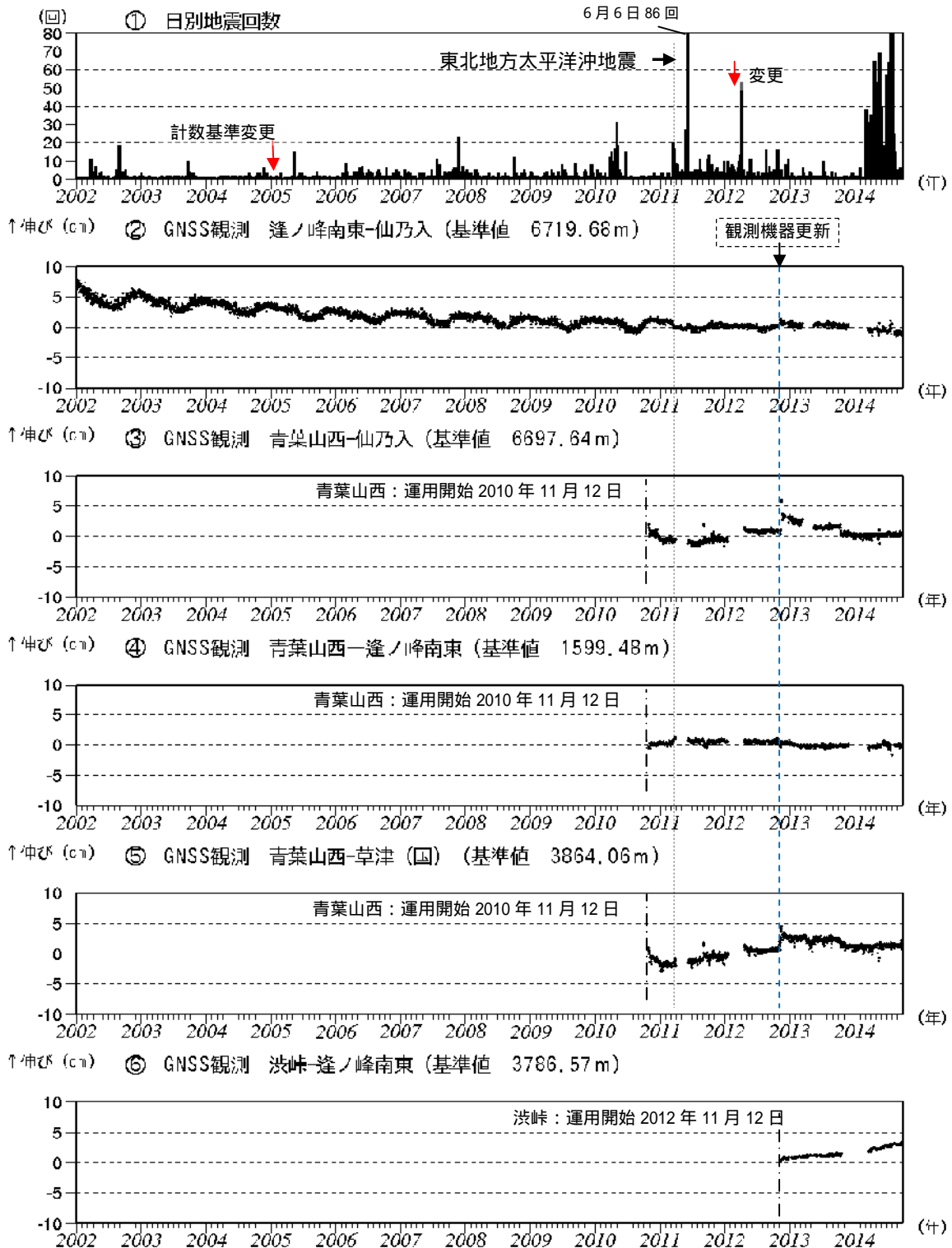
図3 草津白根山 火山活動経過図 (2002年1月1日~2014年9月30日)
