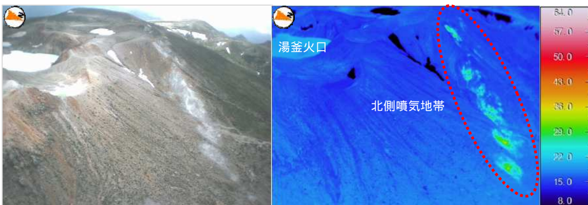
2014年6月23日15時25分 湯釜火口の北東上空から撮影 図7 草津白根山 北側噴気地帯周辺の状況及び地表面温度分布 赤線内が高温領域を示しています。
