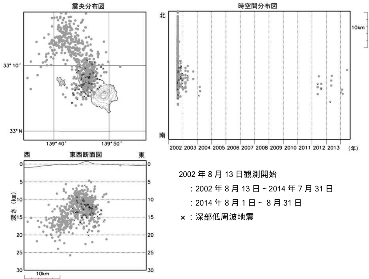
図3 八丈島 震源分布図(2002年8月13日~2014年8月31日)
