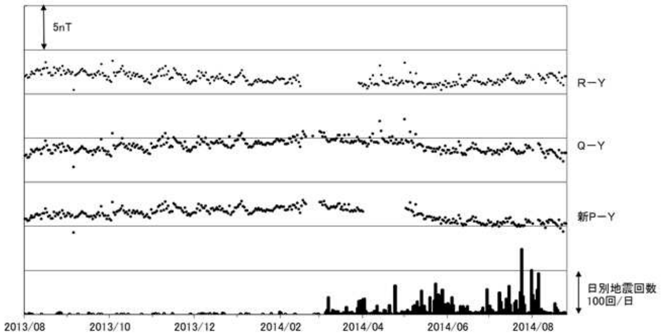
図7 草津白根山 全磁力連続観測による全磁力値の変化及び日別地震回数(2013年8月~2014年8月25日) ・連続観測点P、Q、Rおよび新Pにおける八ヶ岳地球電磁気観測所(東京大学)(Y)との全磁力の夜間日平均値差。最下段は草津白根山で観測された日別地震回数を示しています。 ・2014年5月頃からみられていた湯釜近傍地下の温度上昇を示すと考えられる全磁力変化は、7月以降停滞しています。
