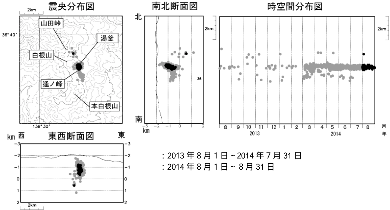
図1 草津白根山 震源分布図(2013年8月1日~2014年8月31日)
