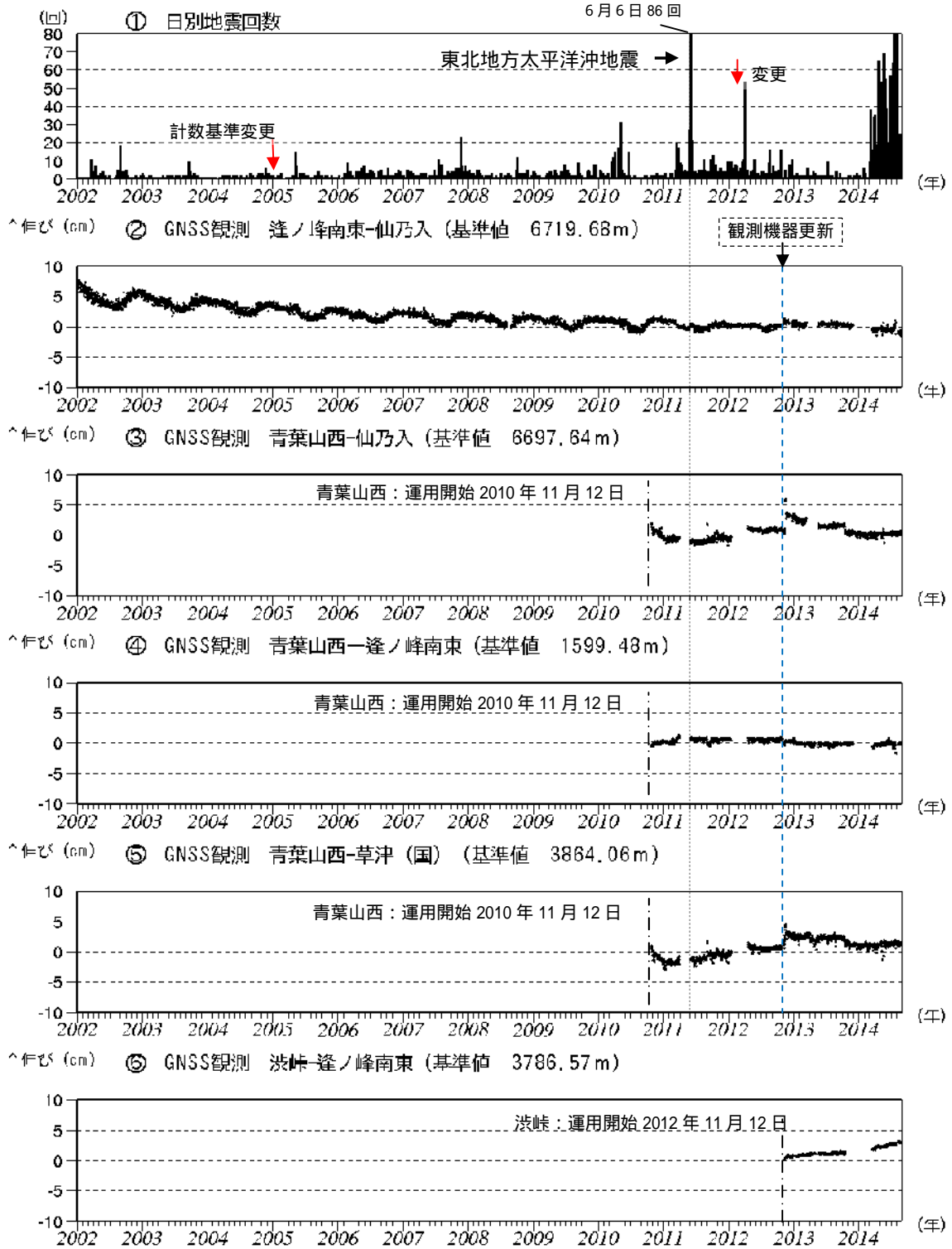
図3 草津白根山 火山活動経過図 (2002年1月1日~2014年8月31日)
