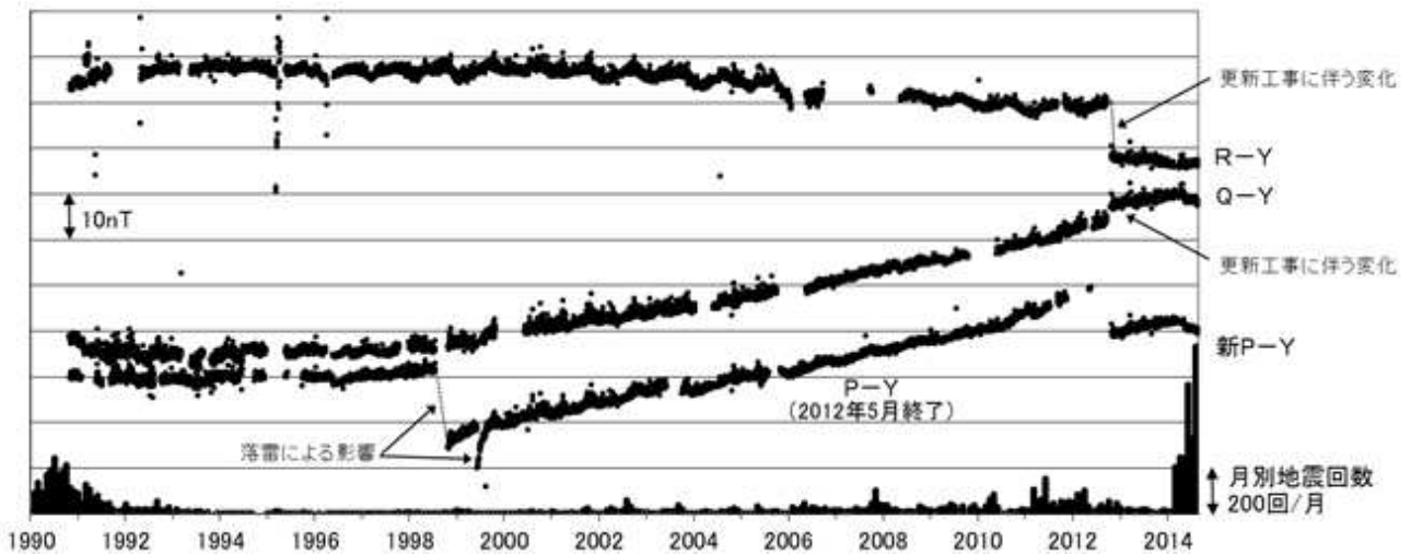
図6 草津白根山 全磁力連続観測による全磁力値の変化及び月別地震回数(1990年~2014年8月25日) ・連続観測点P、Q、Rおよび新Pにおける八ヶ岳地球電磁気観測所(東京大学)(Y)との全磁力の夜間日平均値差。最下段は草津白根山で観測された月別地震回数を示しています。
