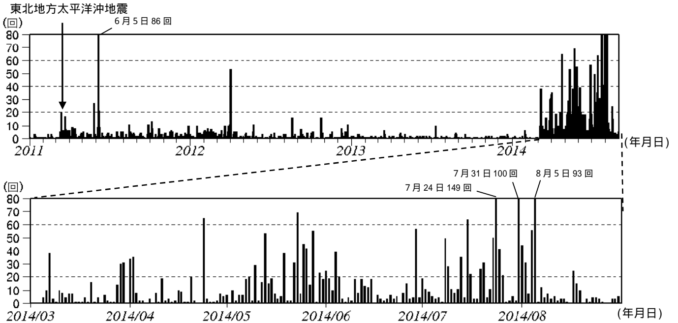
図2 草津白根山 日別地震回数(2011年1月1日~2014年8月31日)
