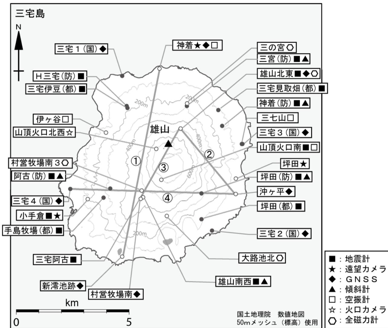
図 8 三宅島 観測点配置図
