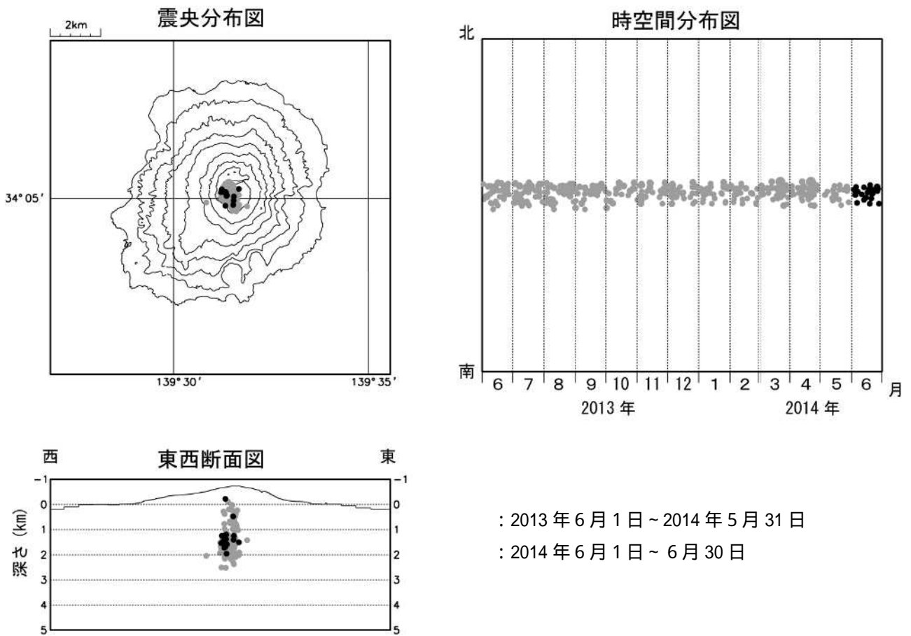
図6 三宅島 震源分布図(2013年6月1日~2014年6月30日)
