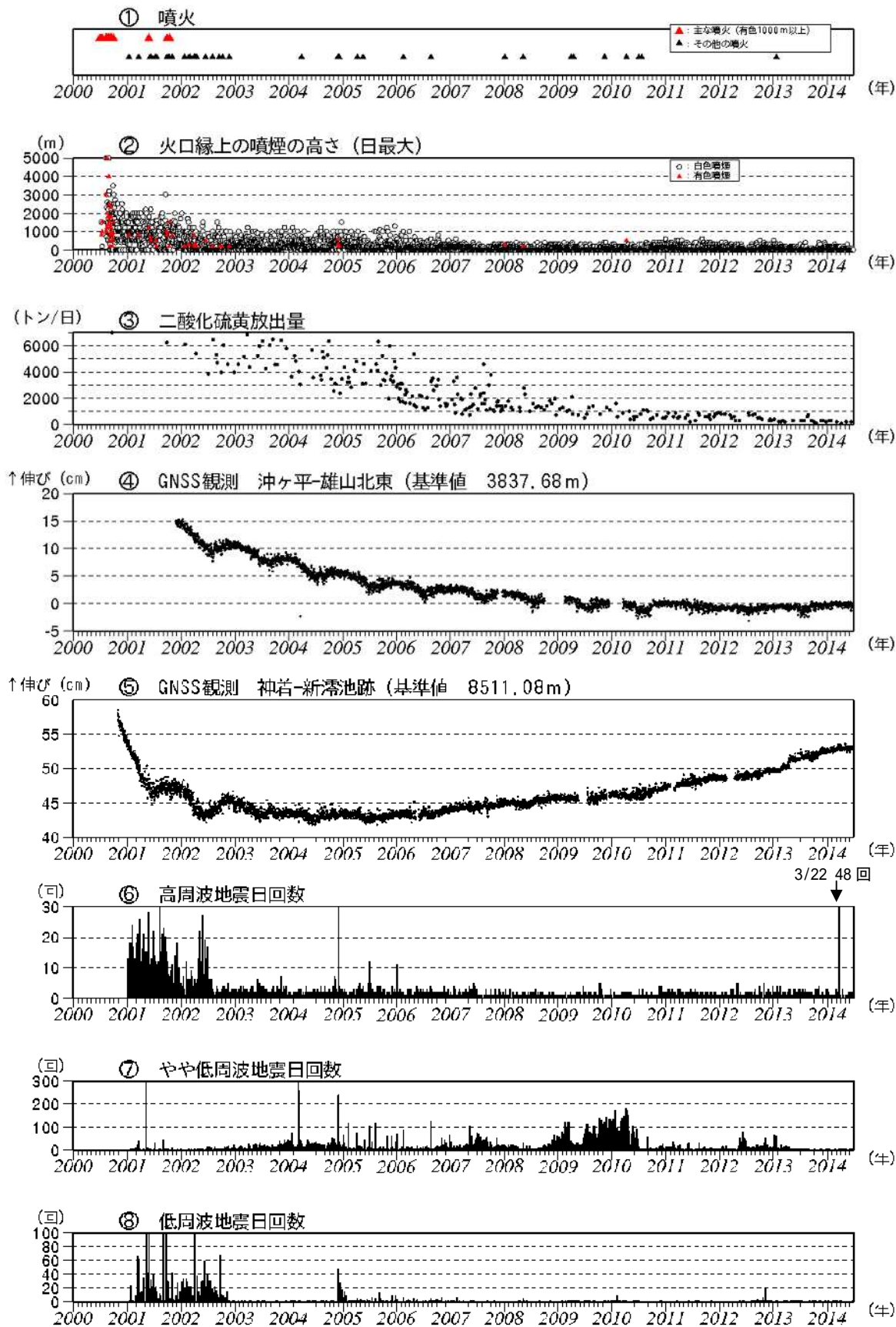
図4 三宅島 火山活動経過図（2000年1月～2014年6月）
