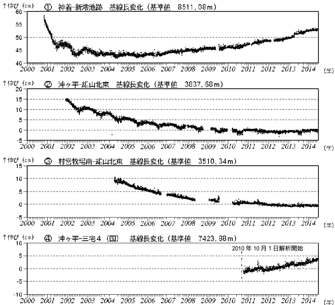
図 5 三宅島 GNSS 連続観測結果(2000 年 1 月～2014 年 6 月) (国): 国土地理院
