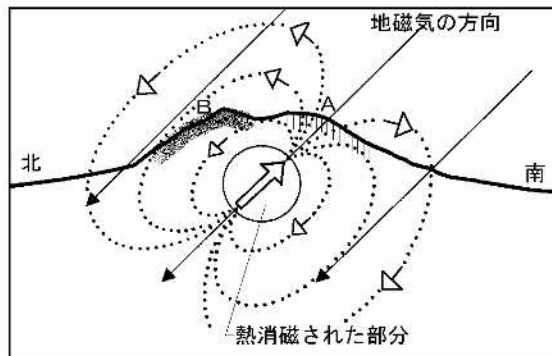
図11 熱消磁に伴う全磁力変化のモデル
