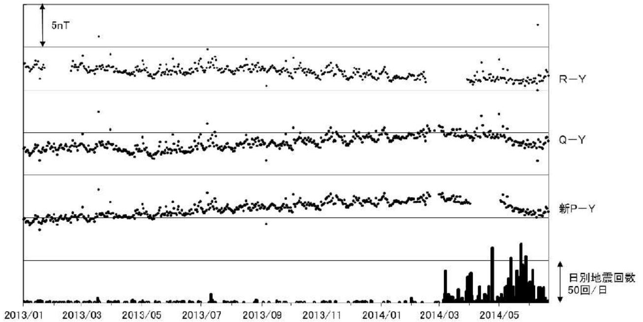
図 9 全磁力連続観測による全磁力値の変化及び日別地震回数(2013年1月~2014年6月20日) 連続観測点P、Q、Rおよび新Pにおける八ヶ岳地球電磁気観測所(東京大学)(Y)との全磁力の夜間日平均値差。最下段は草津白根山で観測された日別地震回数を示しています。
