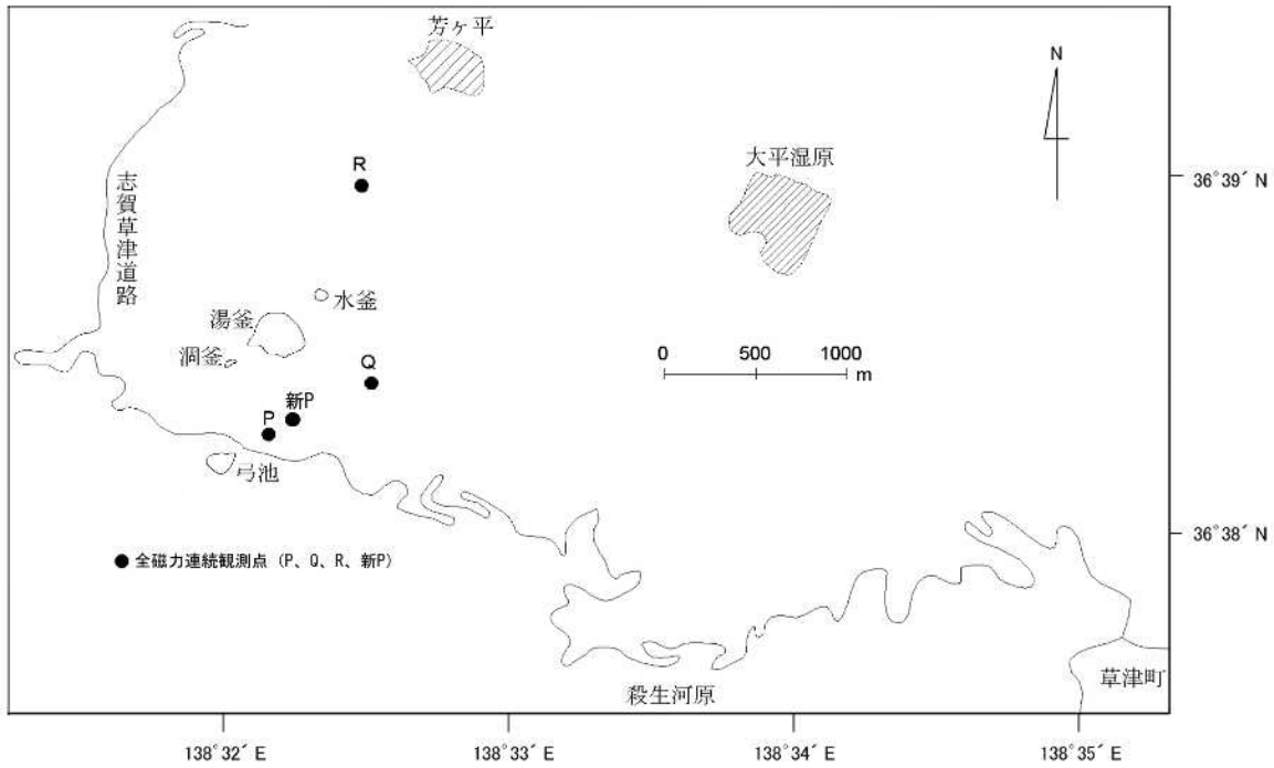
図 10 草津白根山の全磁力観測点配置図
