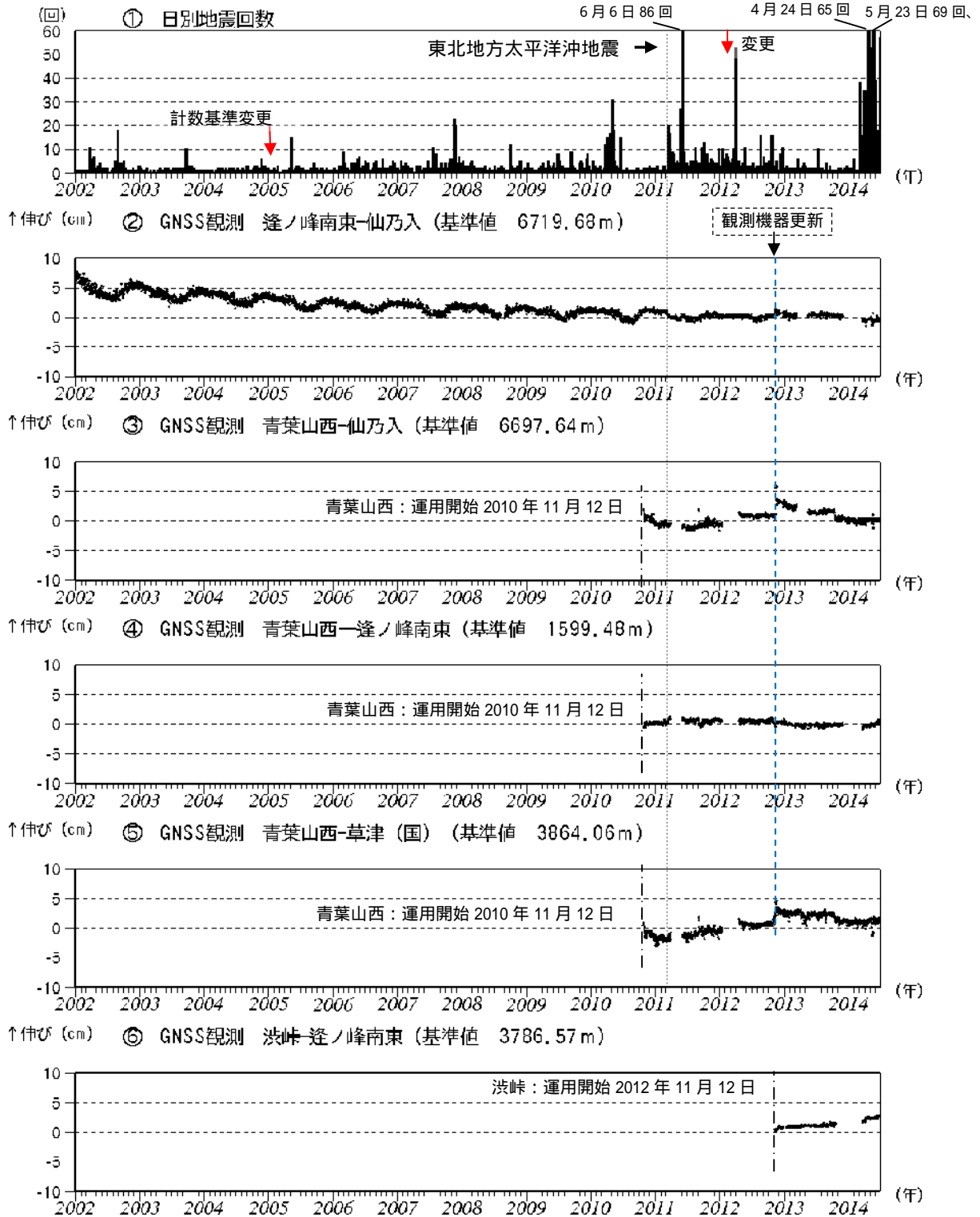
図3 草津白根山 火山活動経過図 (2002年1月1日~2014年6月30日)
