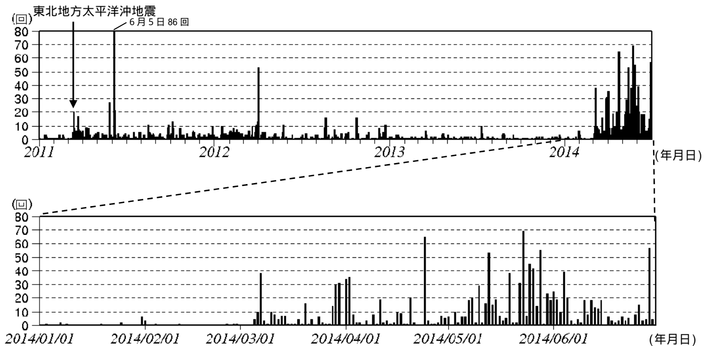
図 2 草津白根山 日別地震回数(2011 年 1 月 1 日～2014 年 6 月 30 日)
