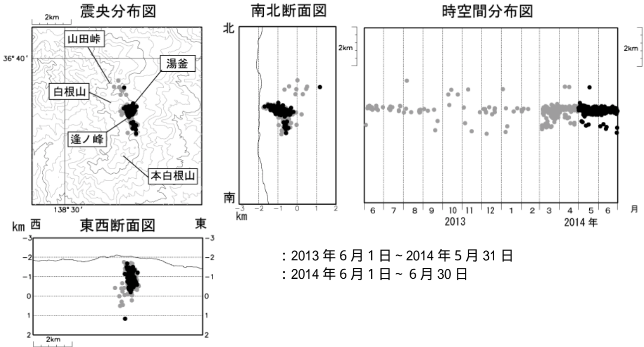
図 1 草津白根山 震源分布図(2013 年 6 月 1 日～2014 年 6 月 30 日)
