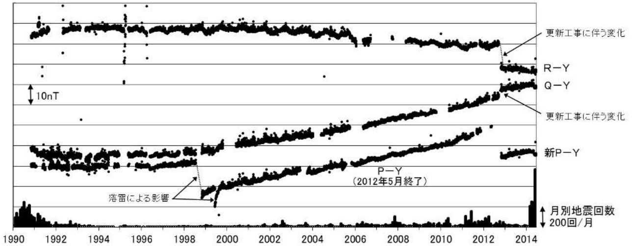
図 8 全磁力連続観測による全磁力値の変化及び月別地震回数(1990年~2014年6月20日) 連続観測点P、Q、Rおよび新Pにおける八ヶ岳地球電磁気観測所(東京大学)(Y)との全磁力の夜間日平均値差。最下段は草津白根山で観測された月別地震回数を示しています。
