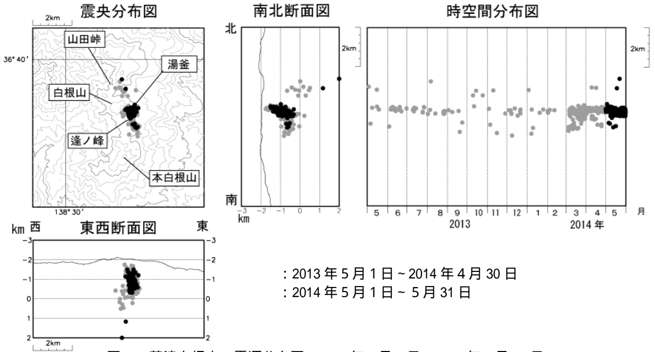
図 1 草津白根山 震源分布図 (2013 年 5 月 1 日 ~ 2014 年 5 月 31 日)
