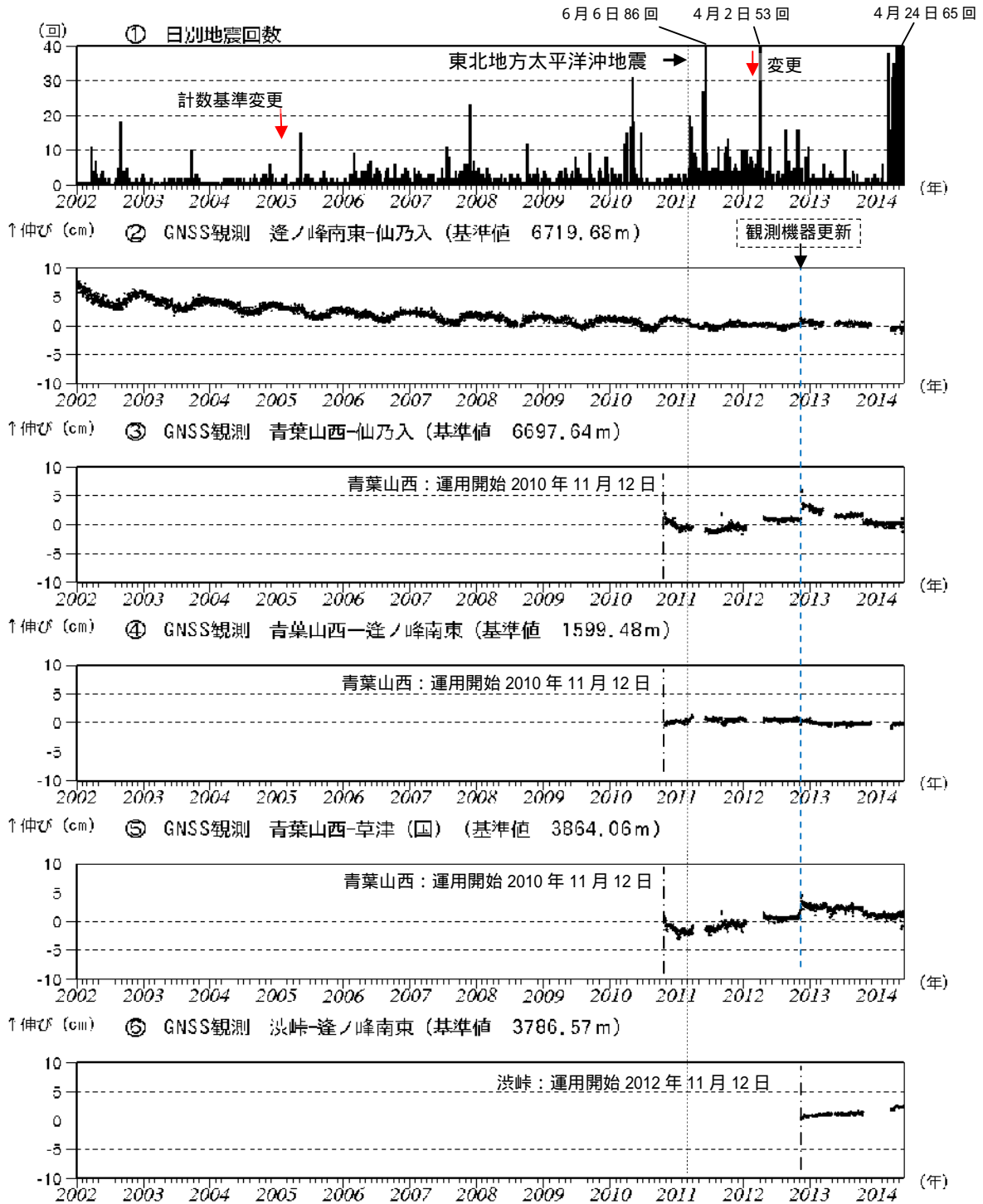
図3 草津白根山 火山活動経過図 (2002年1月1日~2014年5月31日)
