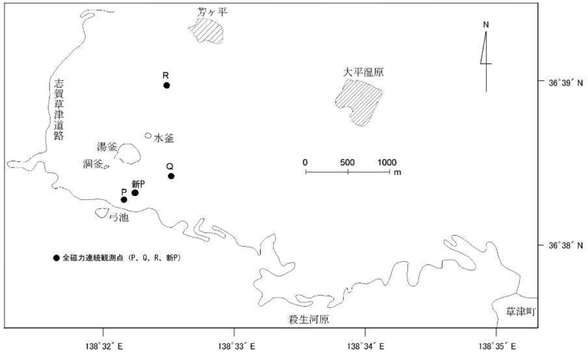
図6 草津白根山の全磁力観測点配置図
