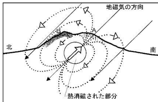
図7 熱消磁に伴う全磁力変化のモデル
