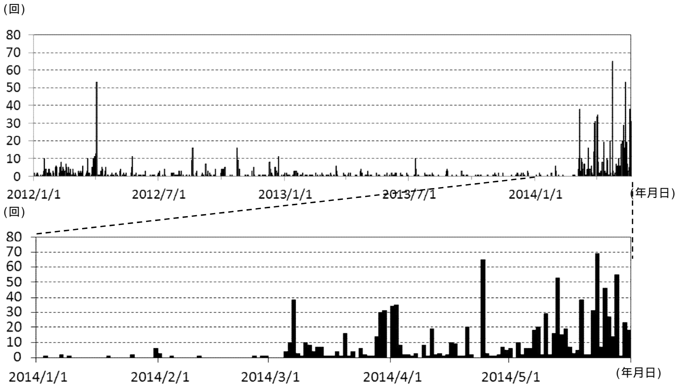
図 2 草津白根山 日別地震回数 (2012 年 1 月 1 日 ~ 2014 年 5 月 31 日)
