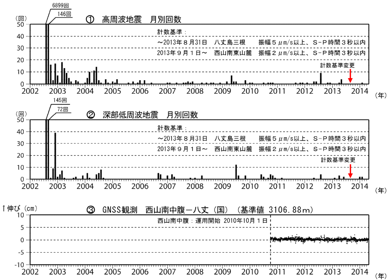
図2 八丈島 火山活動の経過図(2002年8月13日~2014年4月30日)
