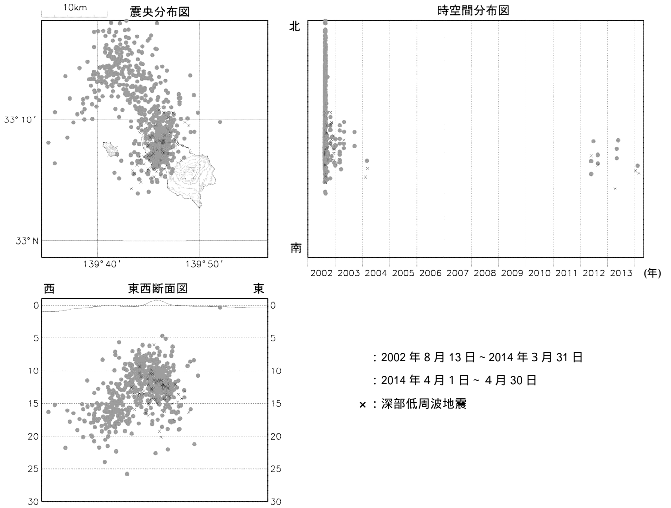
図3 八丈島 震源分布図(2002年8月13日~2014年4月30日) 今期間、八丈島付近に震源が決定された高周波地震及び深部低周波地震はありませんでした。
