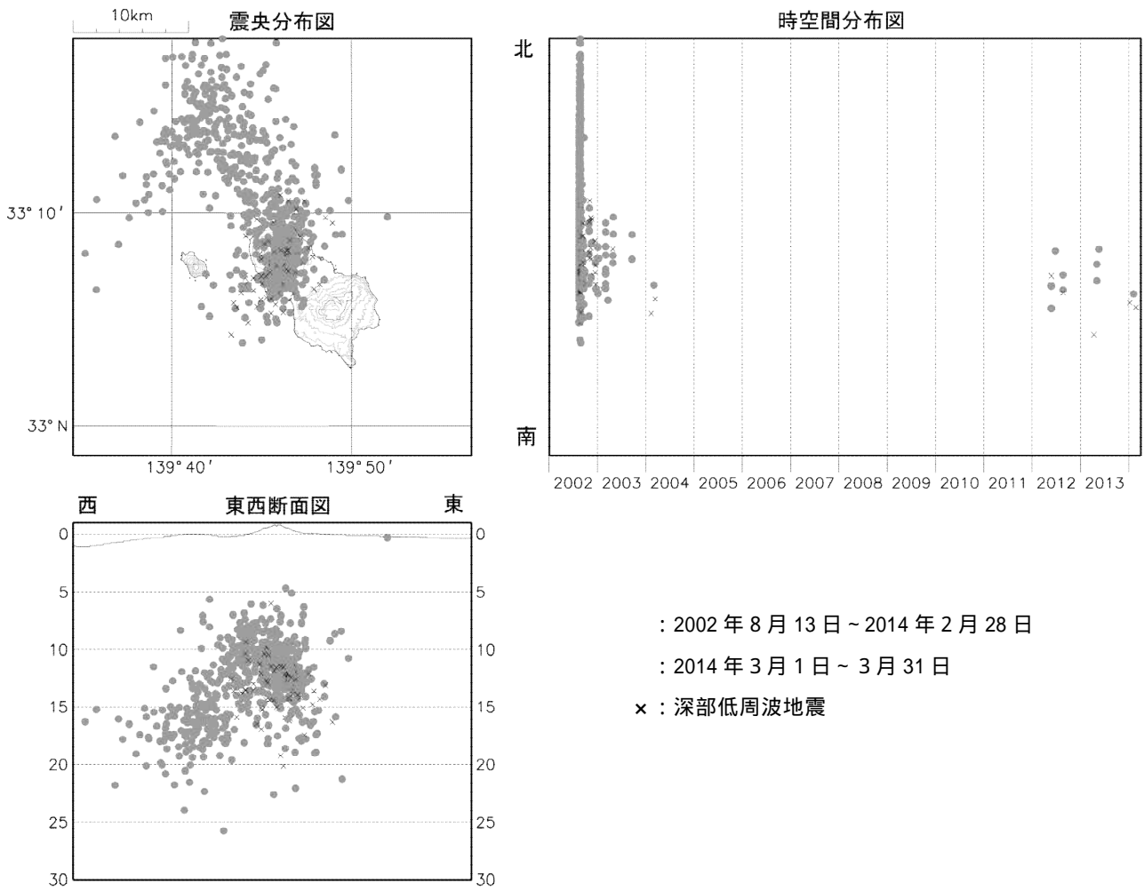
図3 八丈島 震源分布図(2002年8月13日~2014年3月31日) 今期間、八丈島付近に震源が決定された高周波地震及び深部低周波地震はありませんでした。
