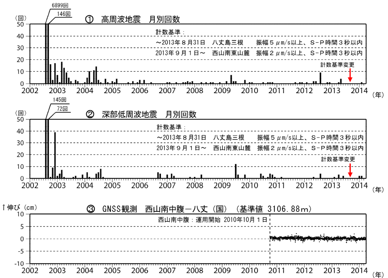
図2 八丈島 火山活動の経過図(2002年8月13日~2014年3月31日)
