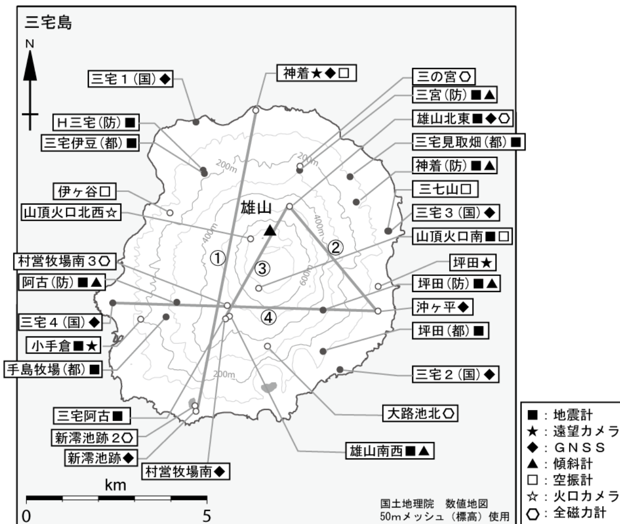
図10 三宅島 観測点配置図
