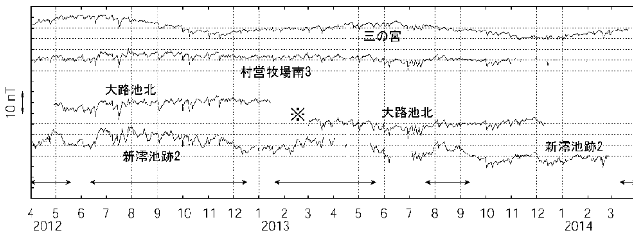
図7 三宅島 全磁力連続観測による全磁力値の変化(2012年4月~2014年3月) 基準点: 雄山北東
