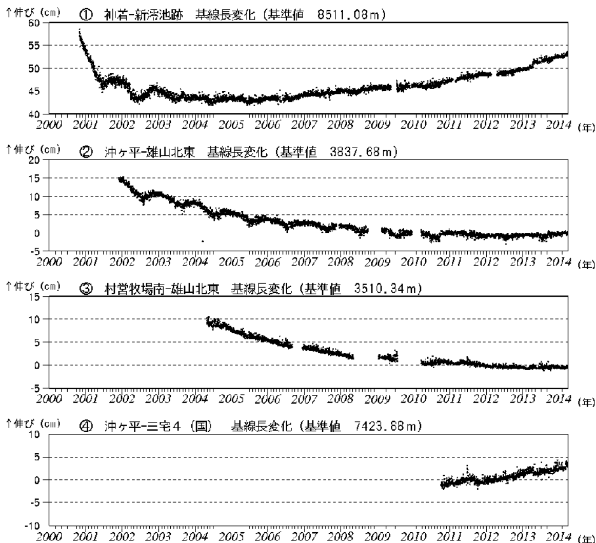
図5 三宅島 GNSS連続観測結果(2000年1月~2014年3月) (国): 国土地理院
