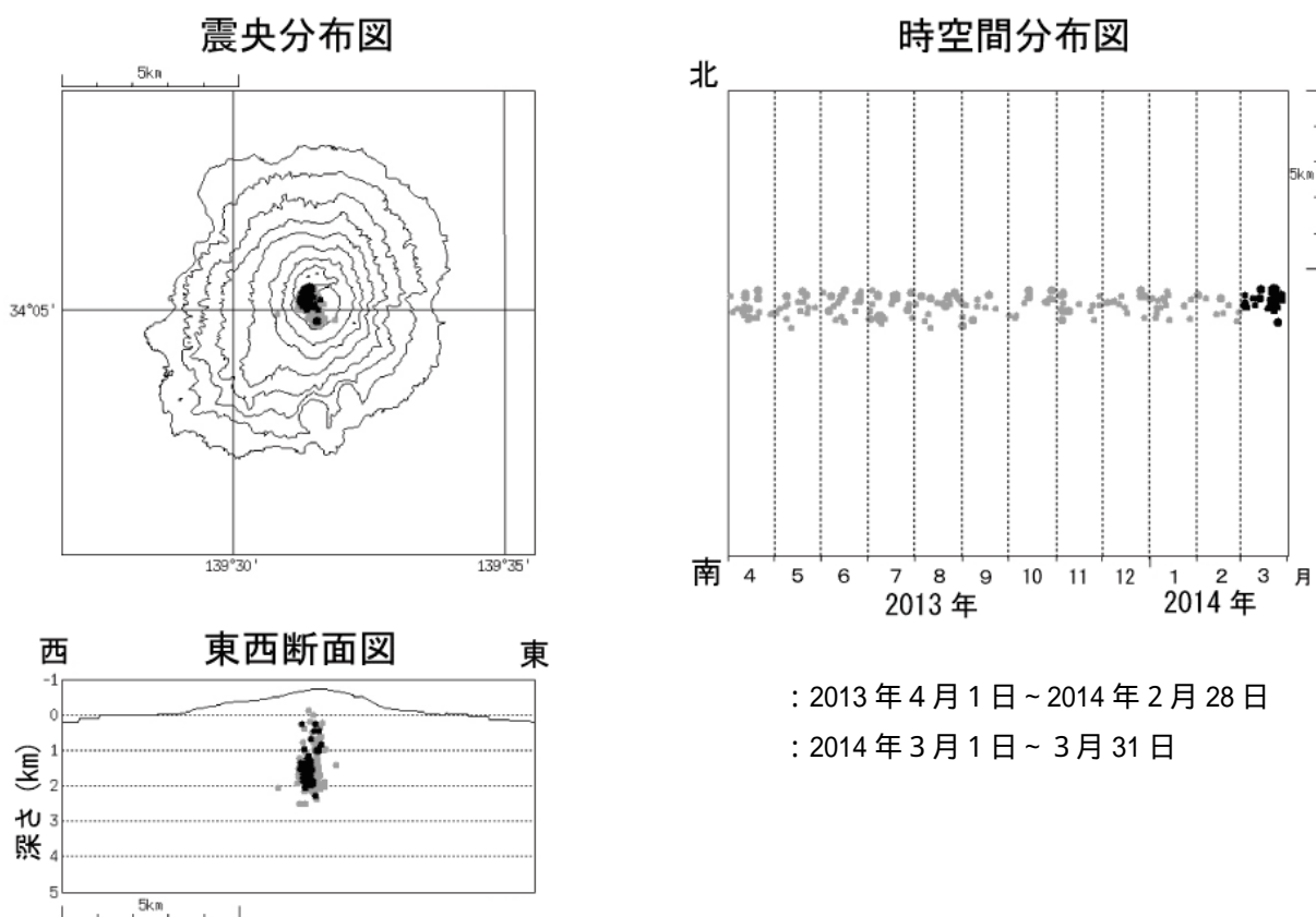
図8 三宅島 震源分布図(2013年4月1日~2014年3月31日)
