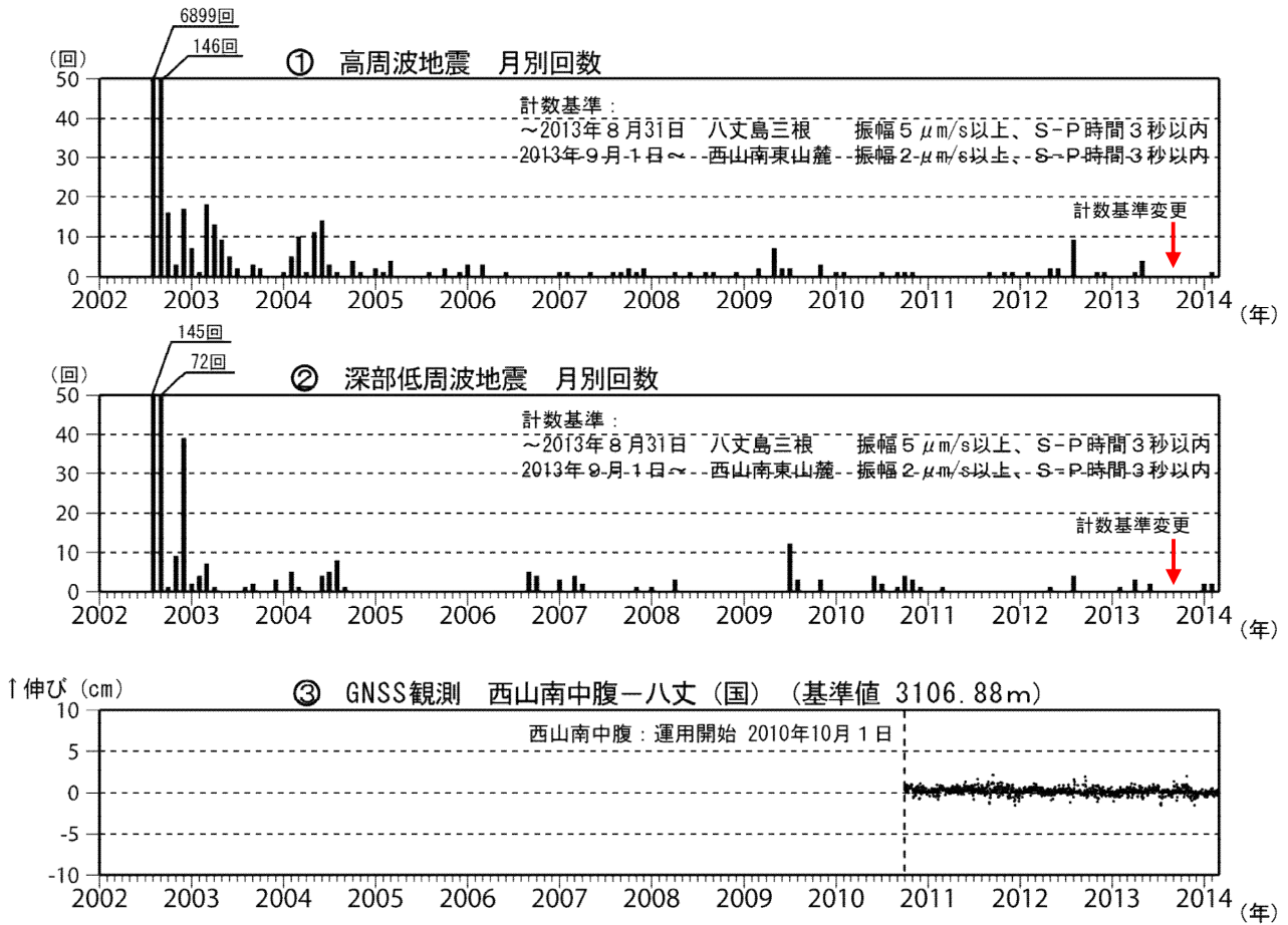
図2 八丈島 火山活動の経過図(2002年8月13日~2014年2月28日)
