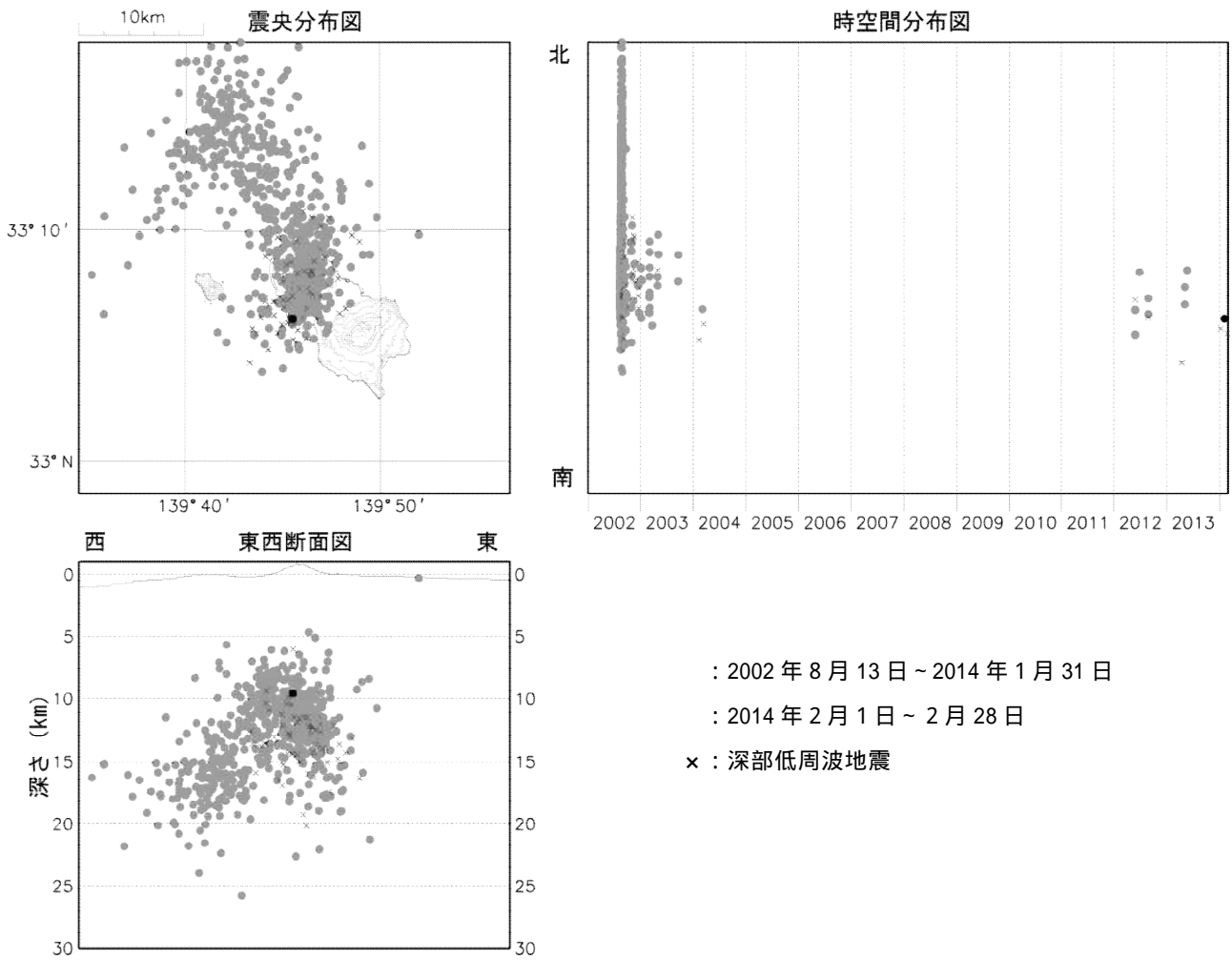
図3 八丈島 震源分布図(2002年8月13日~2014年2月28日)
