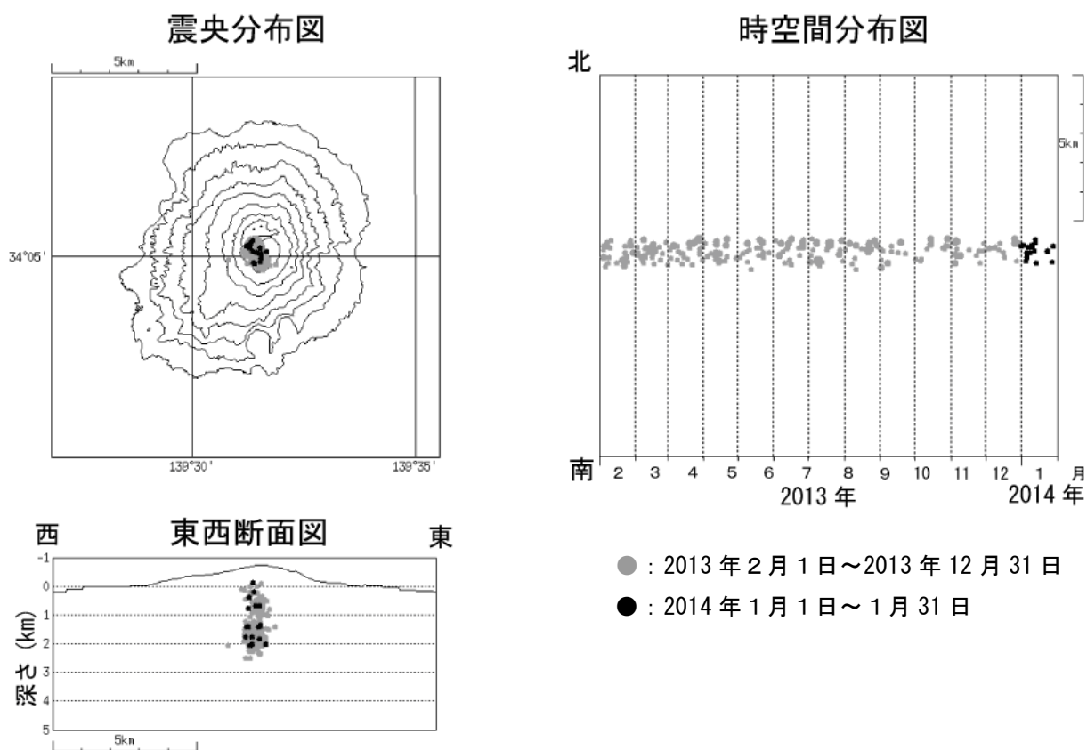
図5 三宅島 震源分布図（2013 年 2 月 1 日～2014 年 1 月 31 日）
