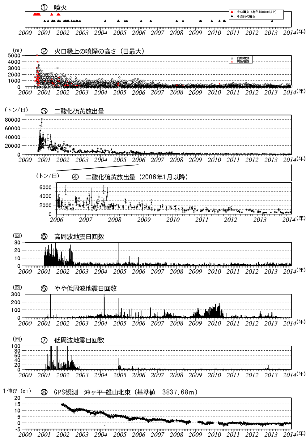
図 2 三宅島 最近の火山活動の経過図 (2000 年 1 月～2014 年 1 月)
