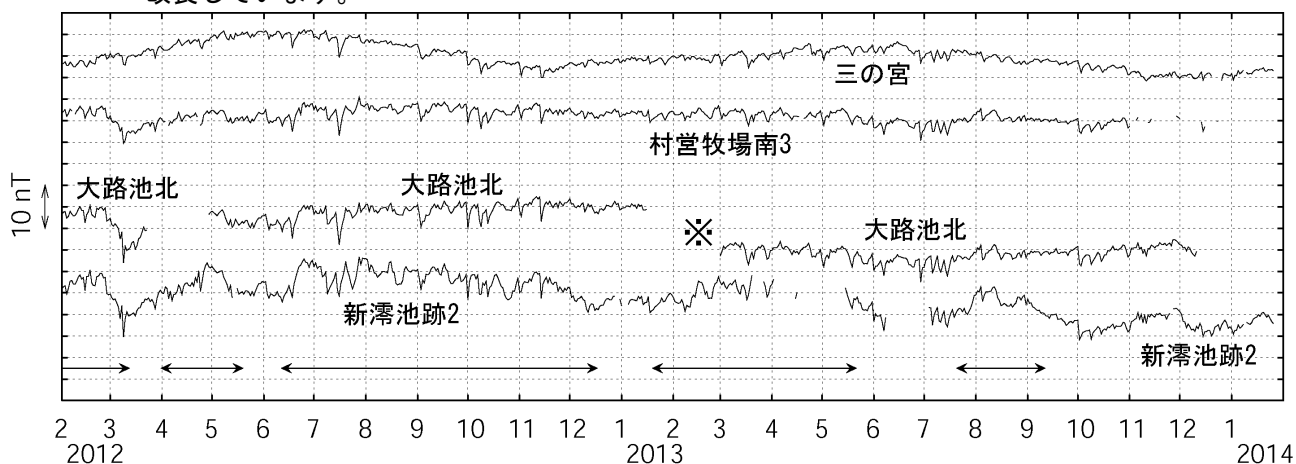
図4 三宅島 全磁力連続観測による全磁力値の変化（2012年2月～2014年1月） 基準点：雄山北東
