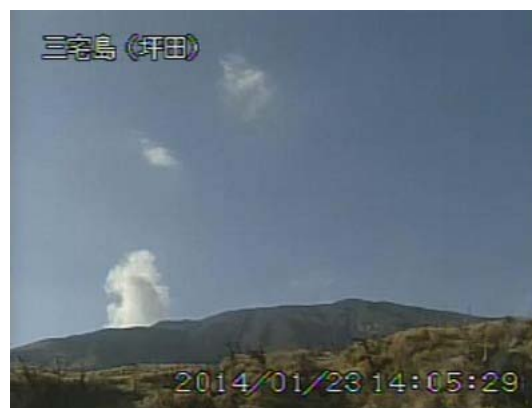
図 1 三宅島 山頂火口からの噴煙の状況 （1 月 23 日、坪田遠望カメラによる）
