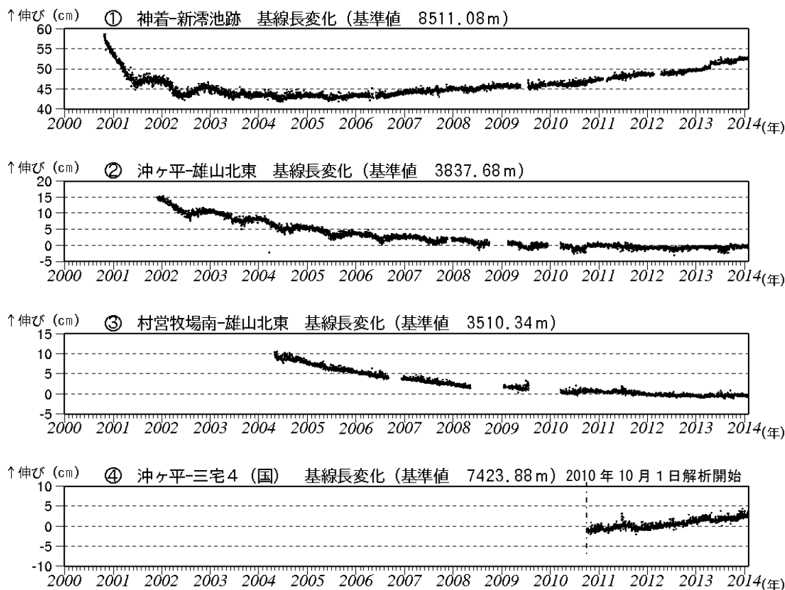
図3 三宅島 GPS 連続観測結果（2000年1月～2014年1月）（国）：国土地理院 ・基線①～④は図7（観測点配置図）の①～④にそれぞれ対応します。 ・グラフの空白部分は欠測を示します。 ・2010年10月以降のデータについては、電離層の影響を補正する等、解析方法を改良しています。
