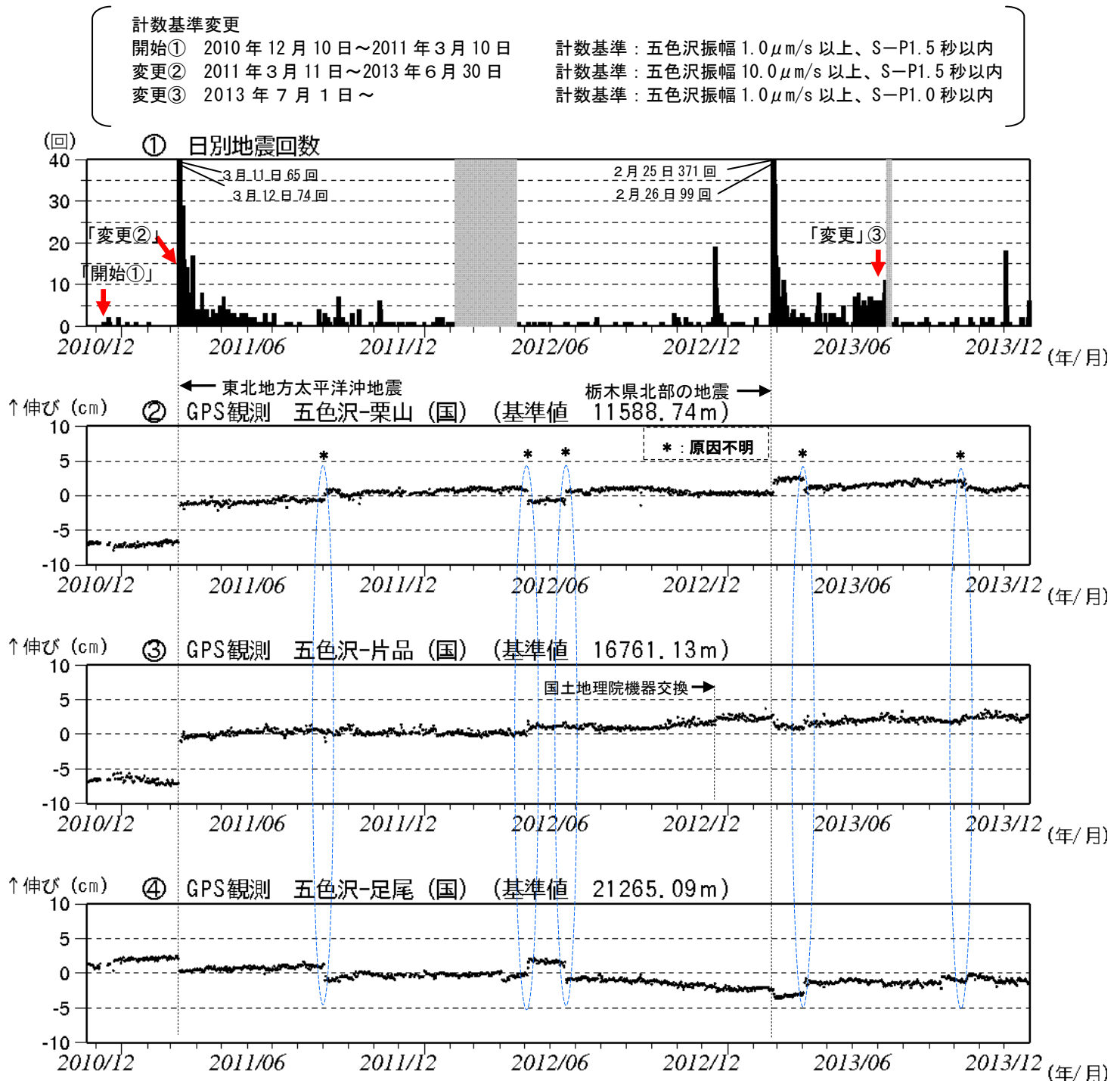
図2 日光白根山 火山活動経過図 (2010 年 11 月 20 日～2013 年 12 月 31 日)
