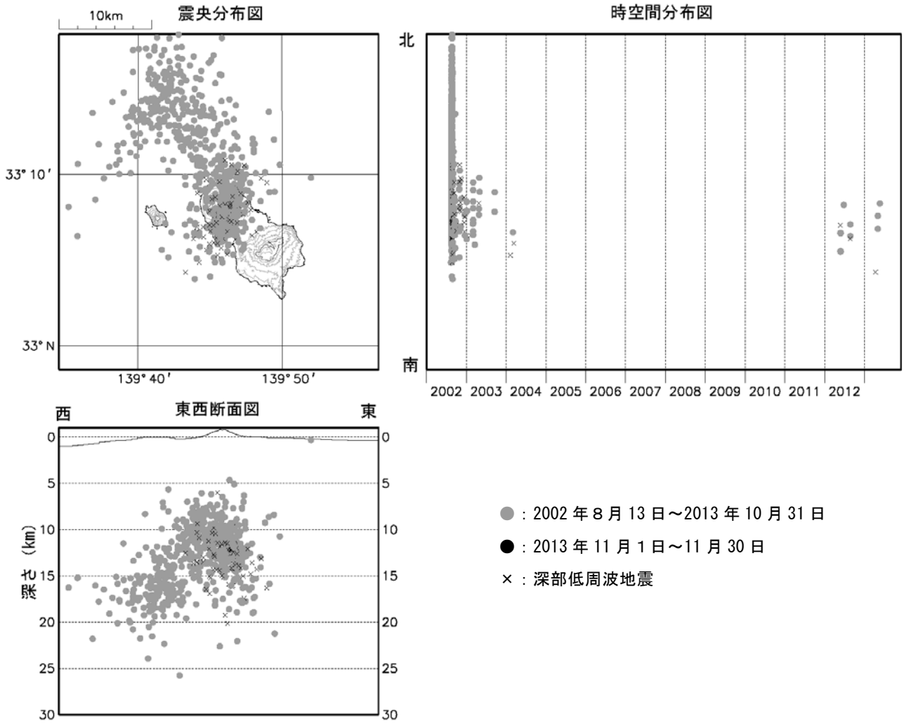
図3 八丈島 震源分布図（2002年8月13日～2013年11月30日） 今期間、八丈島付近に震源が決定された高周波地震及び深部低周波地震はありませんでした。
