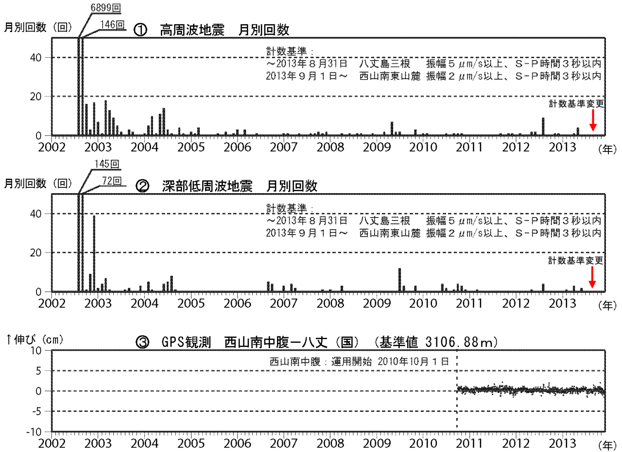
図2 八丈島 火山活動の経過図 (2002年8月13日~2013年11月30日)
